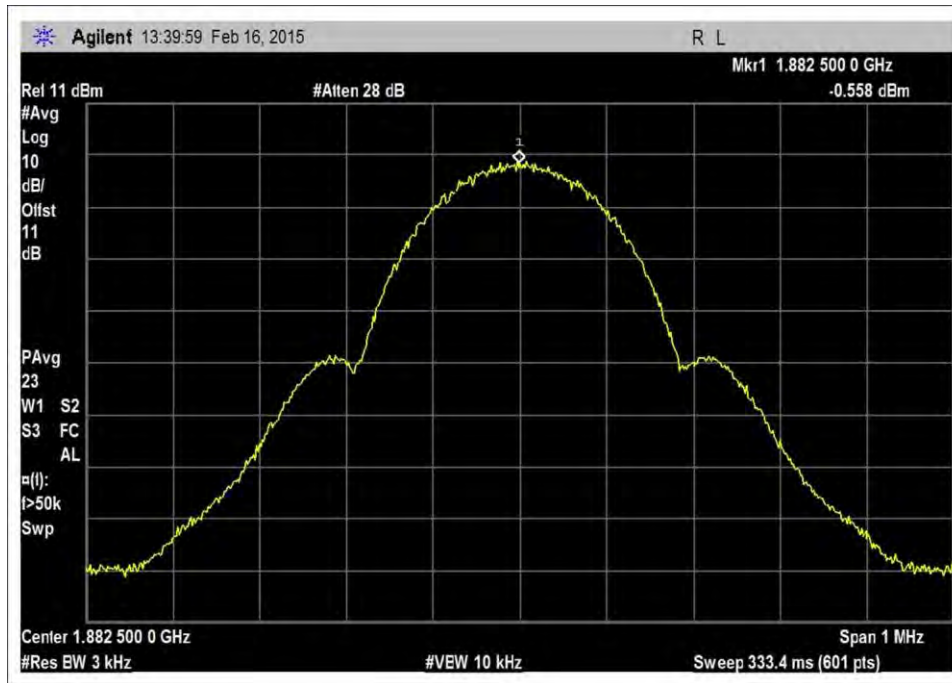
7.10_OBW_UL_1850-1915MHz_GSM_Output
