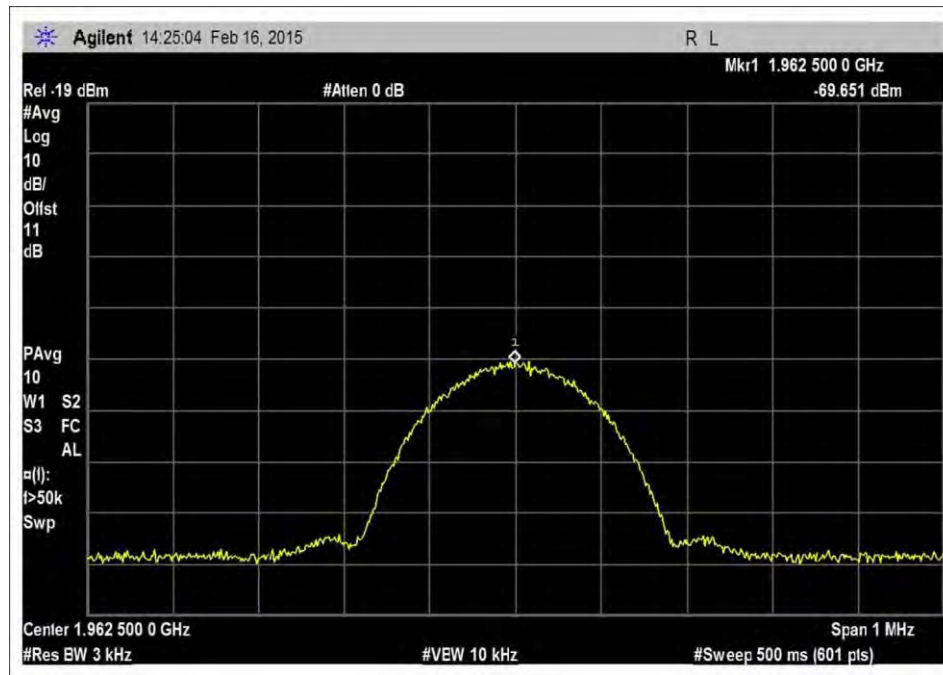
7.10_OBW_DL_1930-1995MHz_GSM__Input
