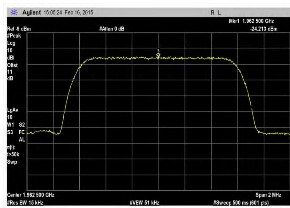
7.10_OBW_DL_1930-1995MHz_CDMA_Output
