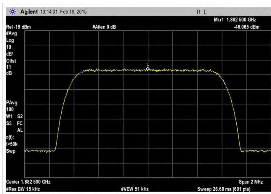
7.10_OBW_UL_1850-1915MHz_CDMA_Input
