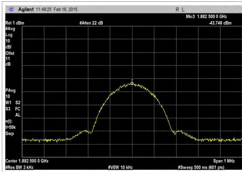
7.10_OBW_UL_1850-1915MHz_GSM__Input
