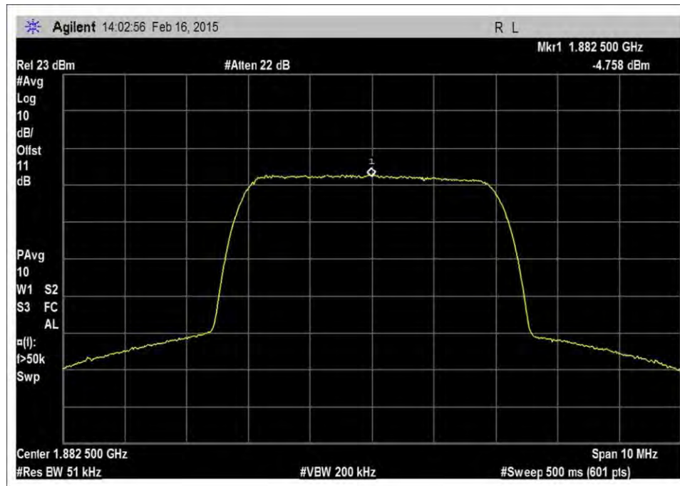
7.10_OBW_UL_1850-1915MHz_WCDMA_Output
