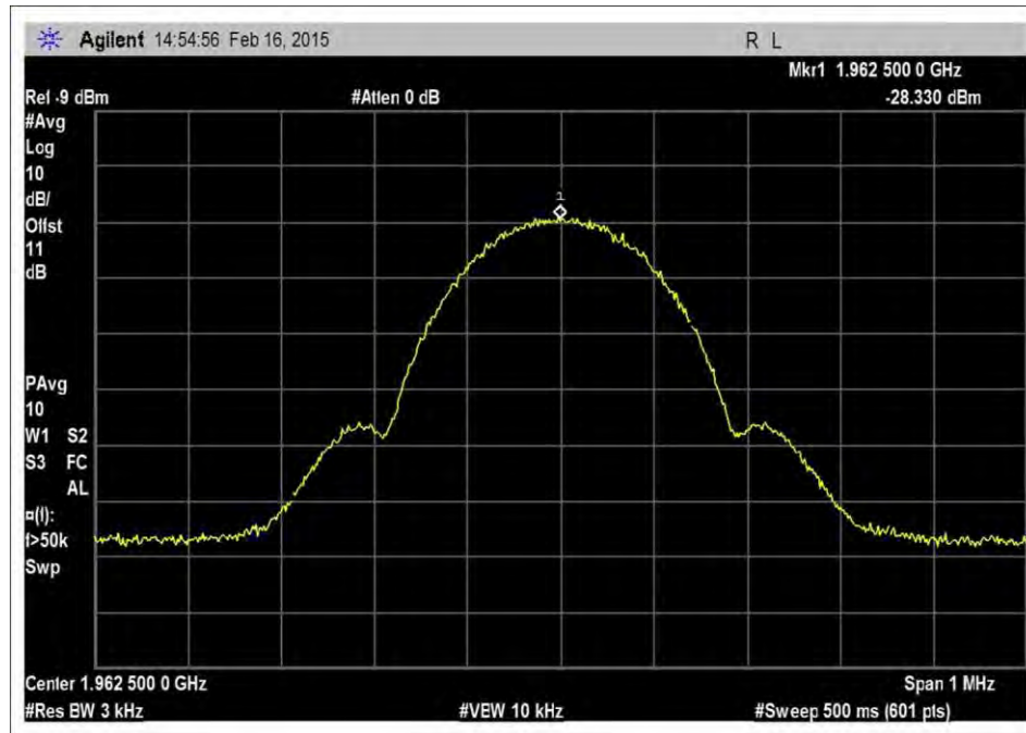
7.10_OBW_DL_1930-1995MHz_GSM_Output
