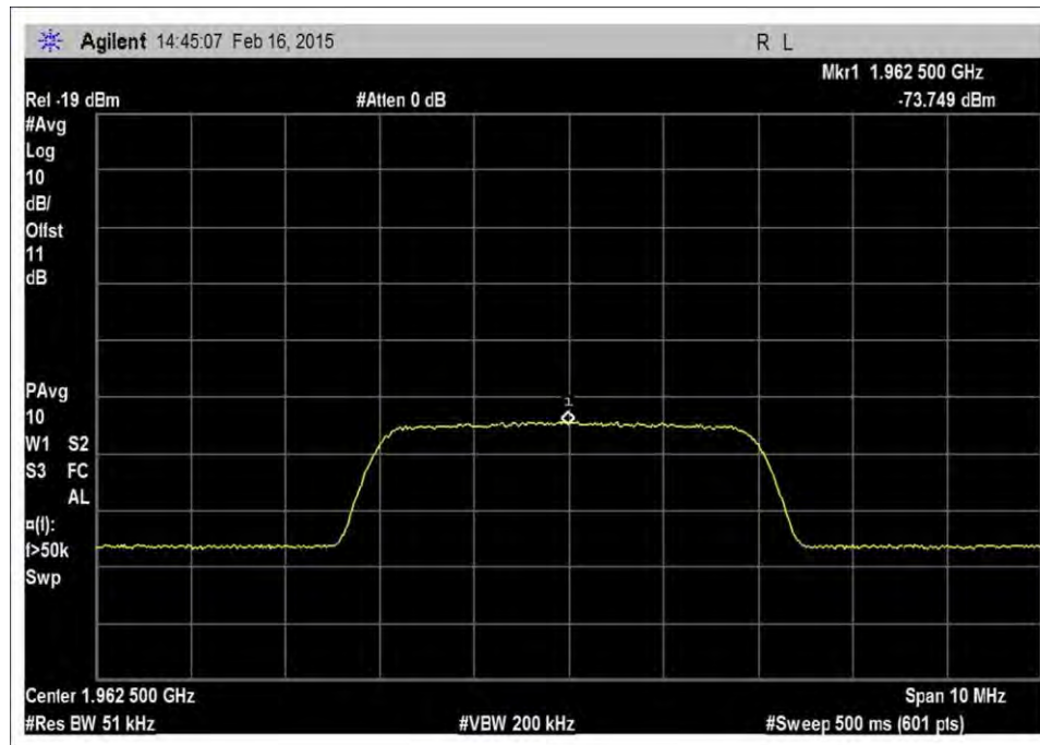
7.10_OBW_DL_1930-1995MHz_WCDMA_Input
