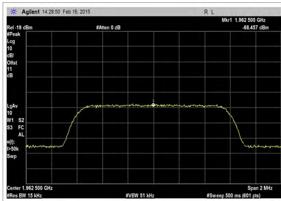
7.10_OBW_DL_1930-1995MHz_CDMA_Input
