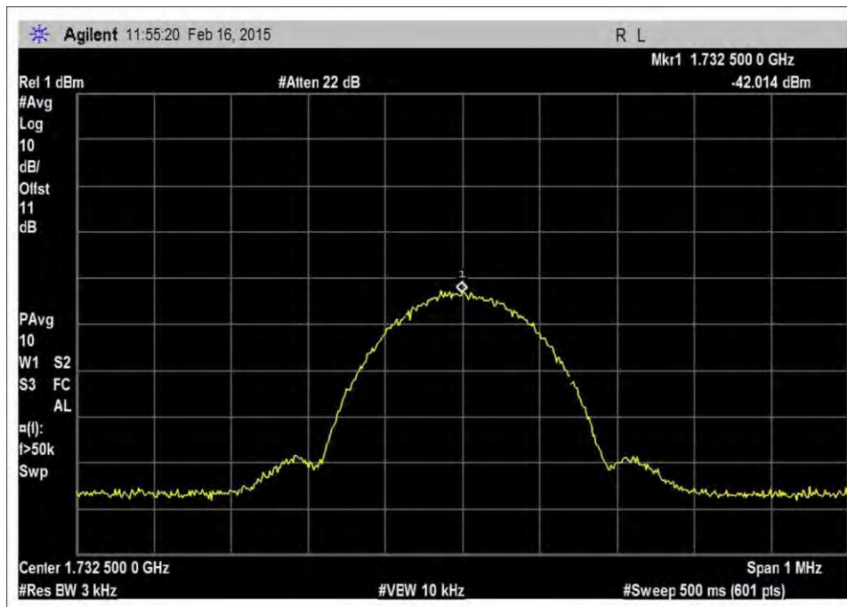
7.10_OBW_UL_1710-1755MHz_GSM__Input
