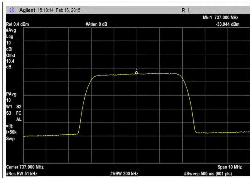
7.10_OBW_DL_728-746MHz_WCDMA_Output
