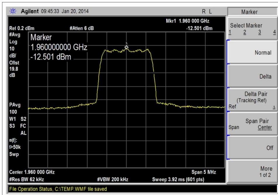
1930-1990MHz DL, CDMA-Output
