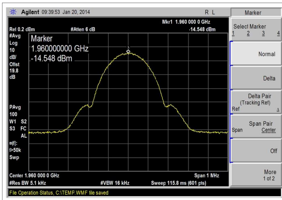
1930-1990MHz DL, GSM-Output
