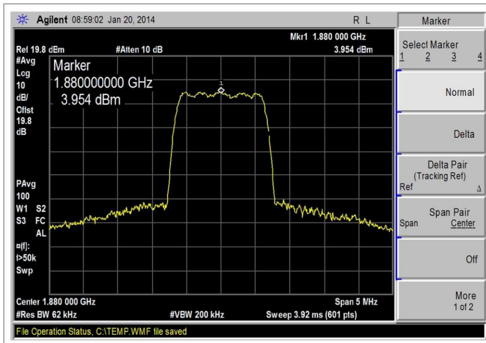
1850-1910MHz UL, CDMA-Output
