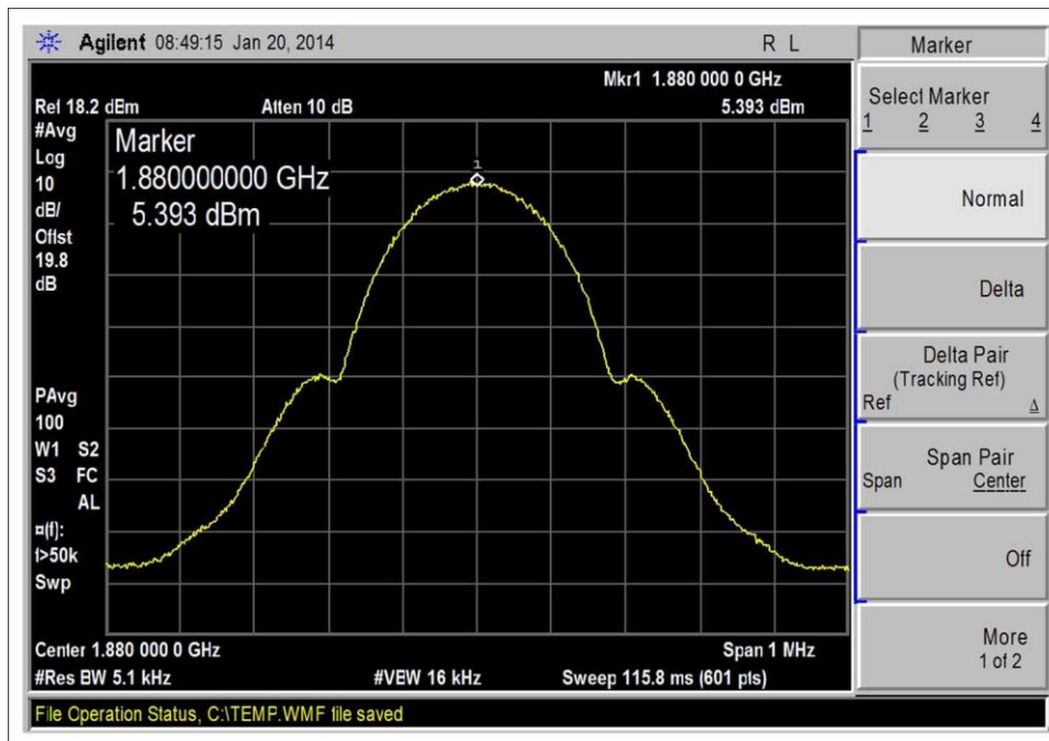
1850-1910MHz UL, GSM-Output
