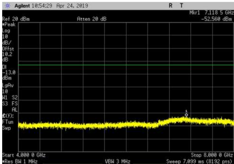
UL_824-849_GSM_4000-8000MHz_MC
