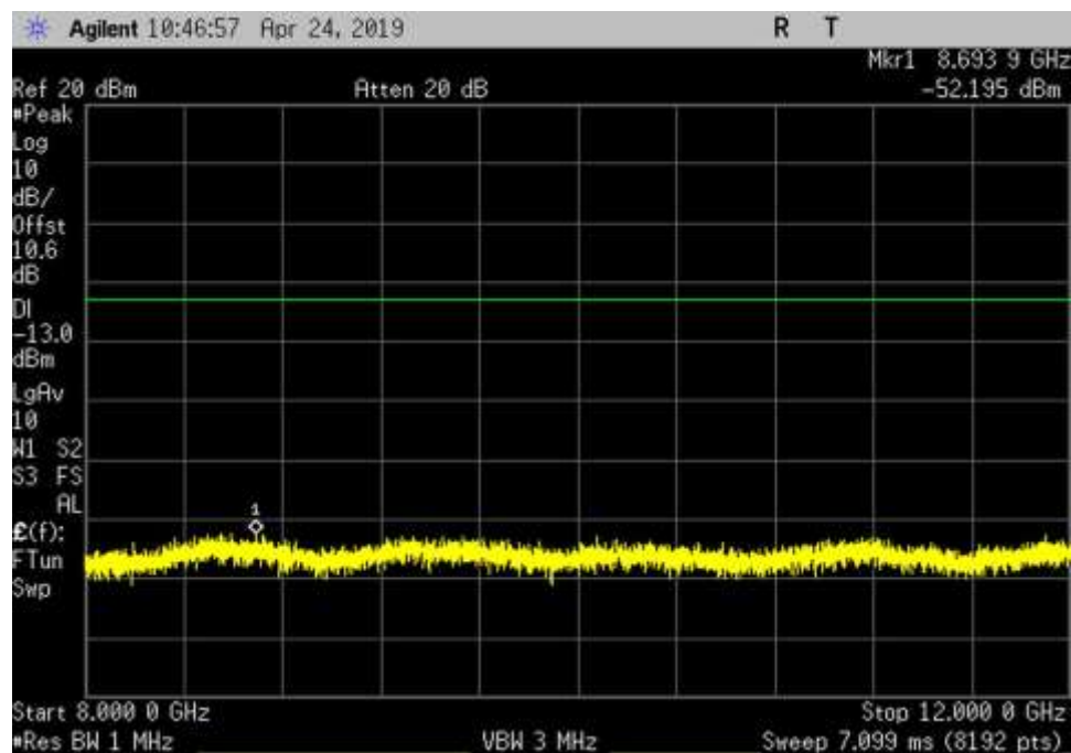
UL_1850-1915_GSM_8000-12000MHz_HC
