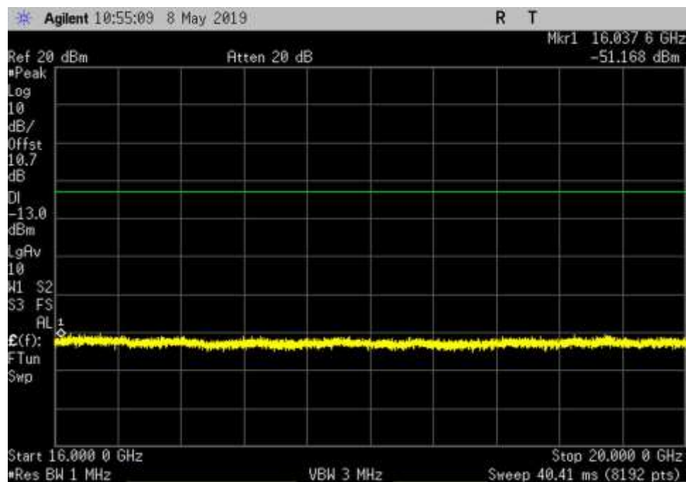
UL_2305-2315_GSM_16000-20000MHz_HC
