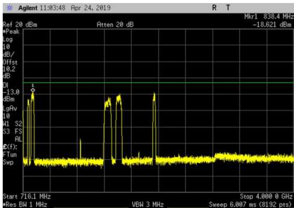
UL_698-716_GSM_716.1- 4000MHz_MC
