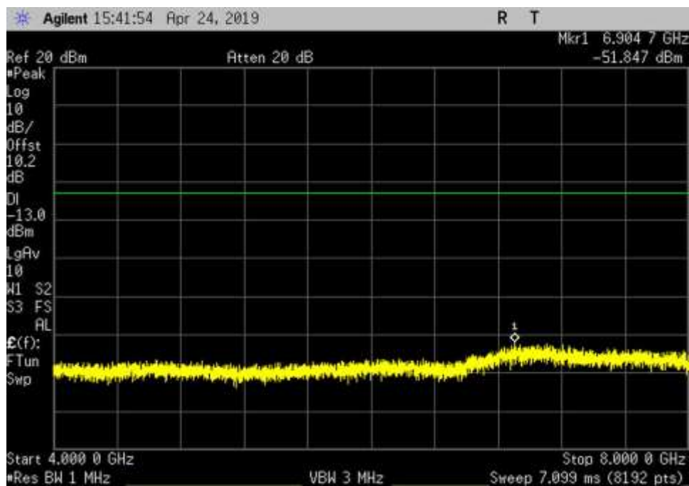
DL_869-894_AWGN_4000- 8000MHz_HC
