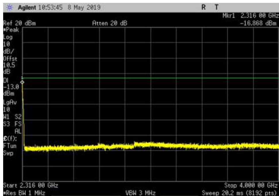
UL_2305-2315_GSM_2316- 4000MHz_HC
