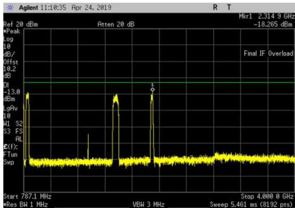
UL_776-787_GSM_787.1- 4000MHz_LC
