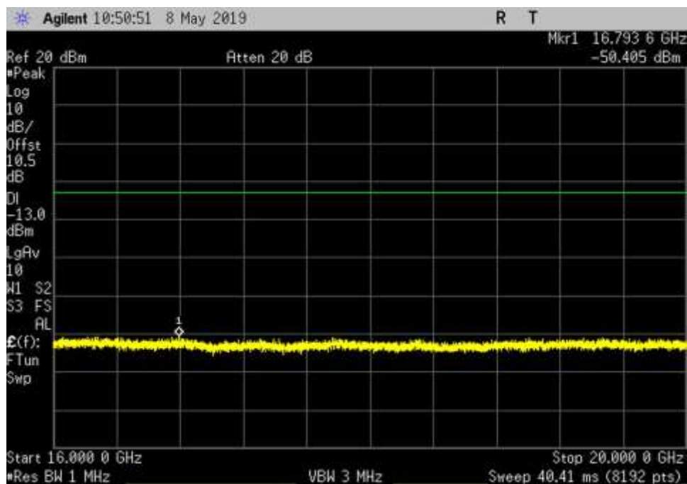
UL_2305-2315_GSM_16000- 20000MHz_LC
