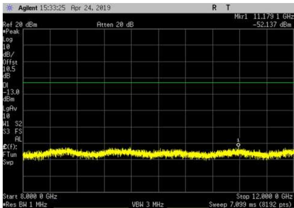
DL_1930-1995_AWGN_ 8000- 12000MHz_MC
