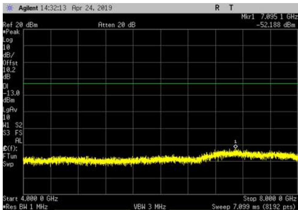
DL_869-894_GSM_4000-8000MHz_MC
