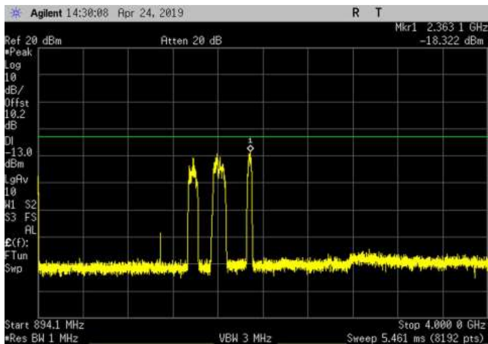
DL_869-894_GSM_ 894.1- 4000MHz_LC
