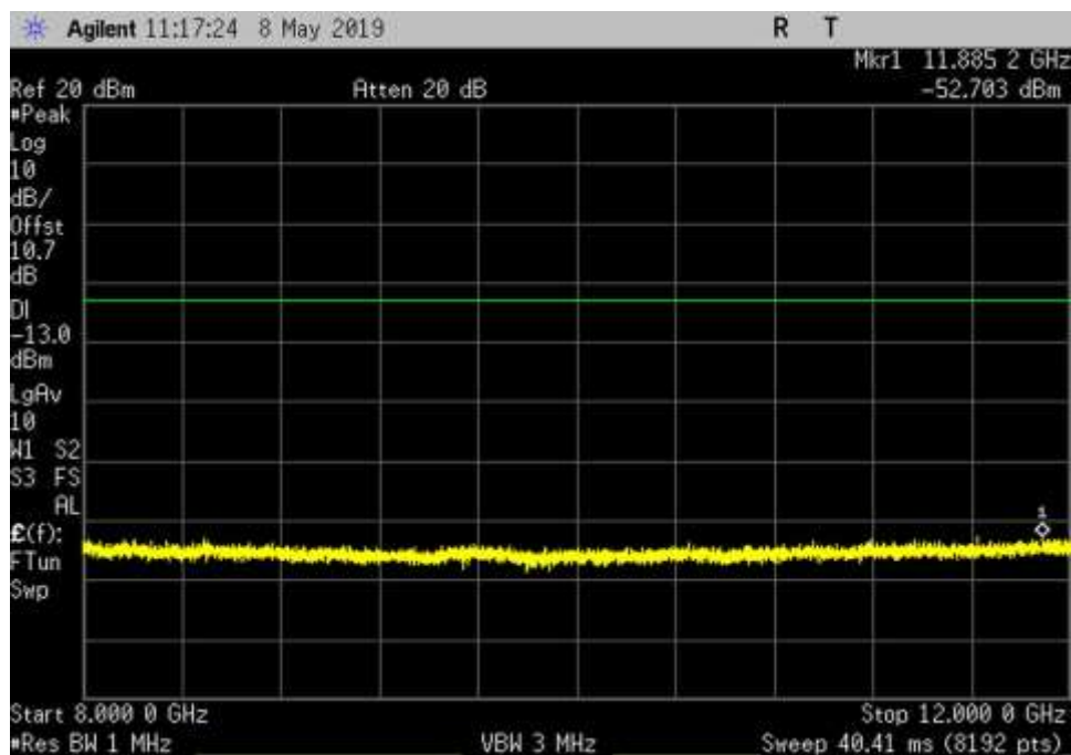
UL_2305-2315_GSM_8000-12000MHz_HC
