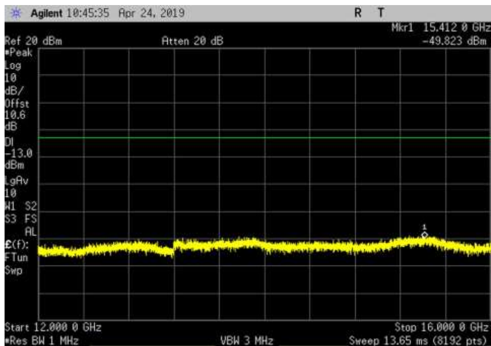
UL_1850-1915_GSM_12000- 16000MHz_MC
