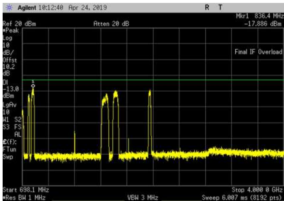
UL_663-698_GSM_698.1- 4000MHz_MC
