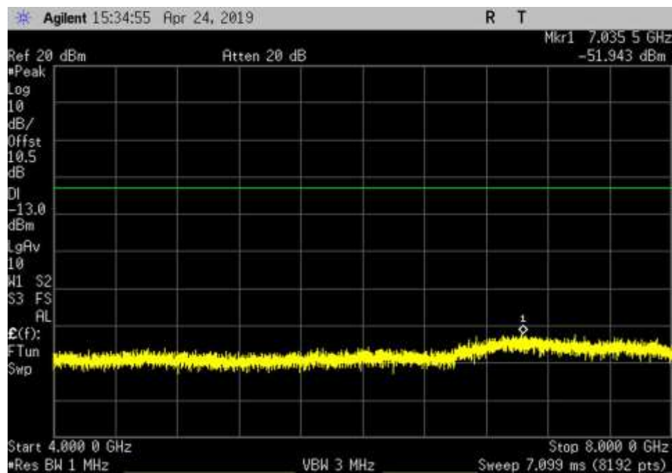
DL_1930-1995_AWGN_4000- 8000MHz_HC
