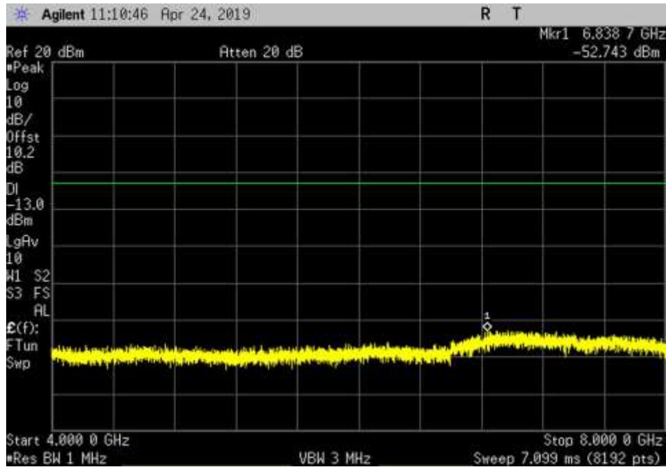
UL_776-787_GSM_4000-8000MHz_LC
