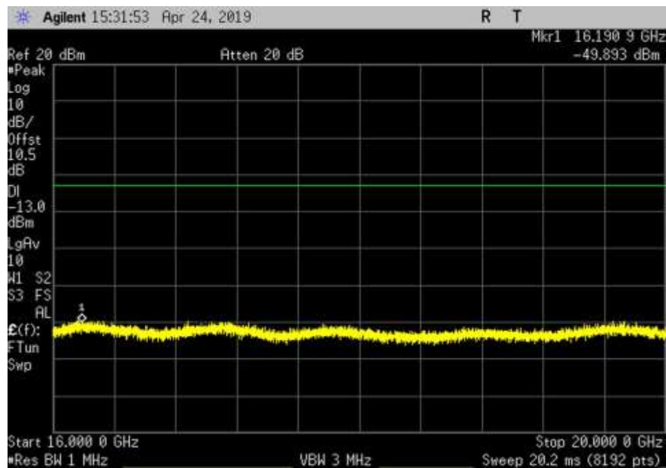
DL_1930-1995_AWGN_16000-20000MHz_LC
