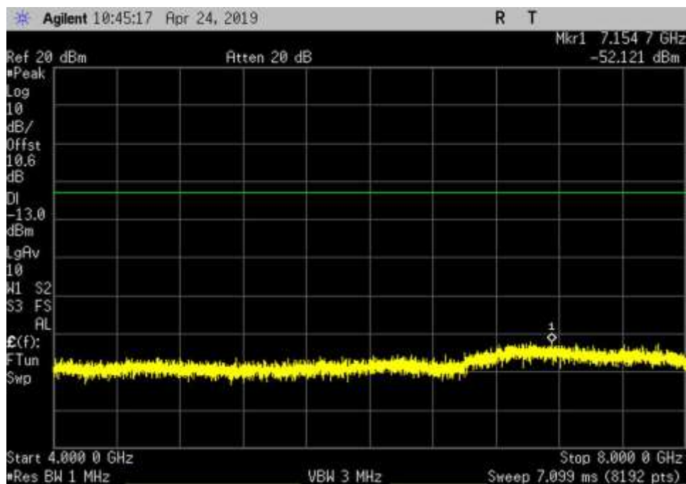
UL_1850-1915_GSM_4000-8000MHz_MC
