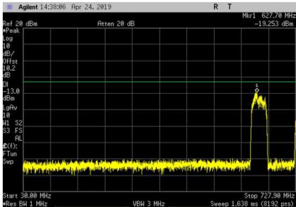
DL_728-746_GSM_30- 727.9MHz_MC
