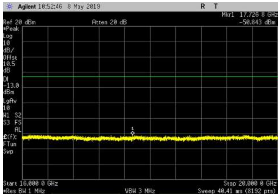
UL_2305-2315_GSM_16000-20000MHz_MC
