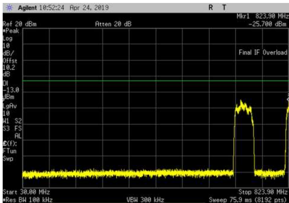
UL_824-849_GSM_30- 823.9MHz_LC
