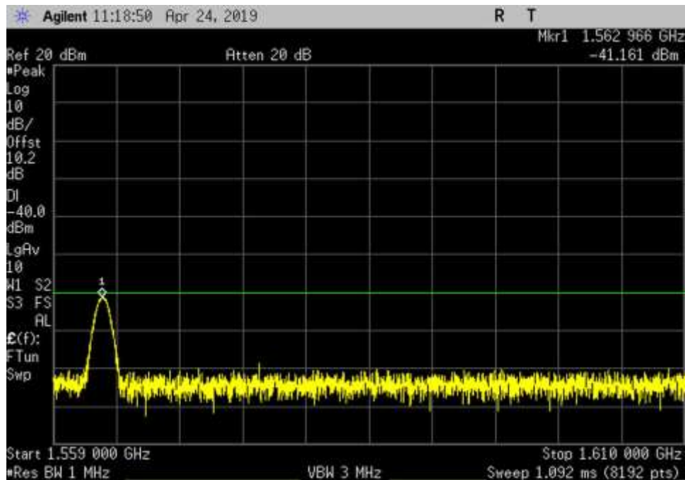
UL_776-787_GSM_1559-1610MHz_MC
