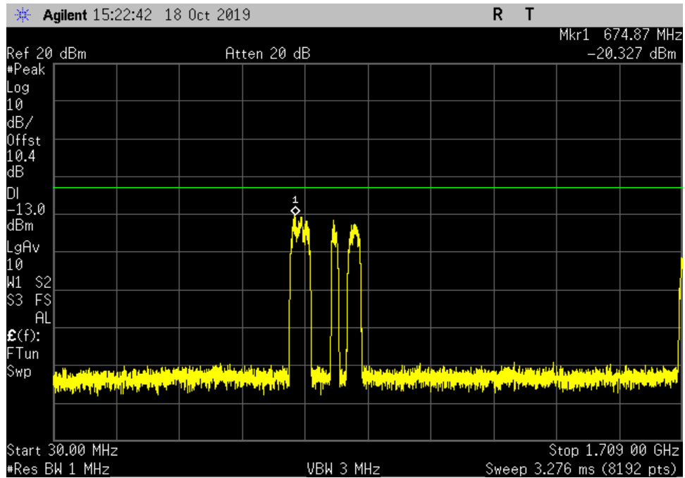
UL_1710-1755_GSM_30- 1709MHz_HC
