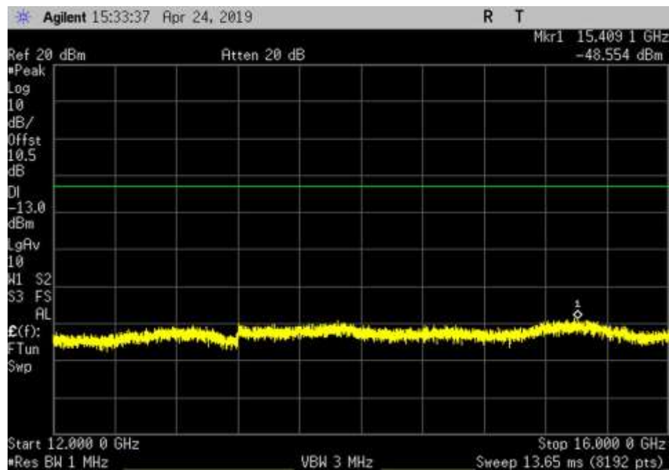
DL_1930-1995_AWGN_12000- 16000MHz_MC
