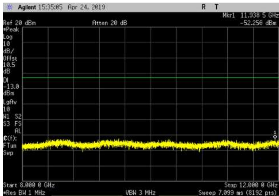
DL_1930-1995_AWGN_8000-12000MHz_HC
