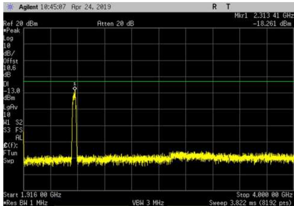
UL_1850-1915_GSM_1916- 4000MHz_MC
