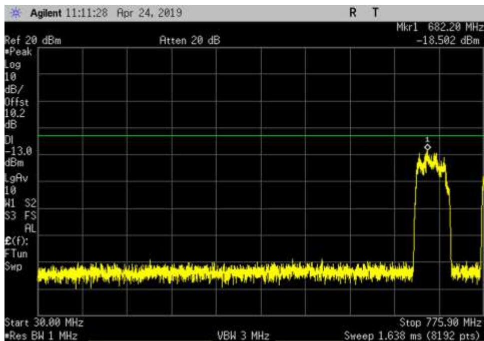
UL_776-787_GSM_30- 775.9MHz_MC
