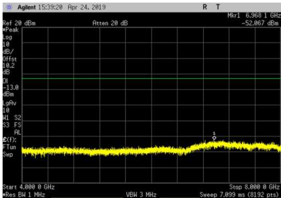
DL_869-894_AWGN_4000- 8000MHz_MC
