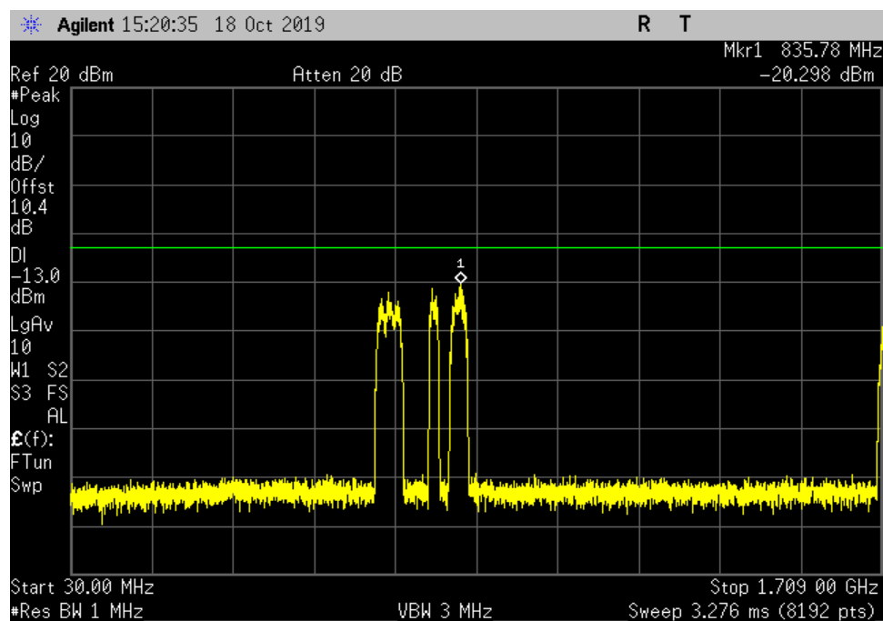
UL_1710-1755_GSM_30-1709MHz_MC
