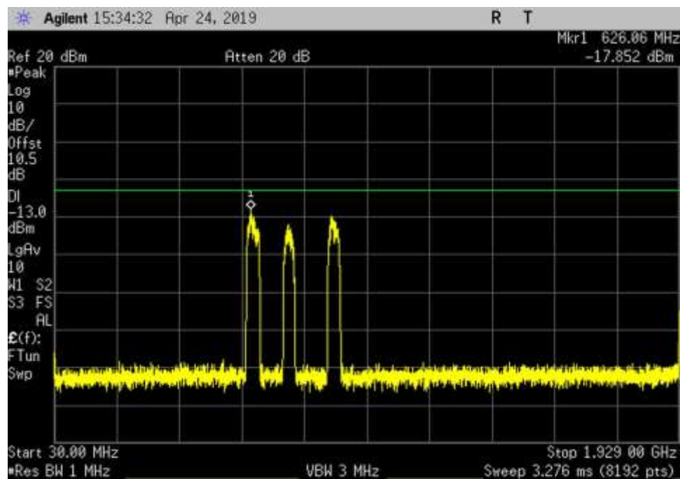
DL_1930-1995_AWGN_30- 1929MHz_HC
