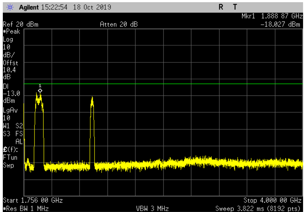
UL_1710-1755_GSM_1756- 4000MHz_HC
