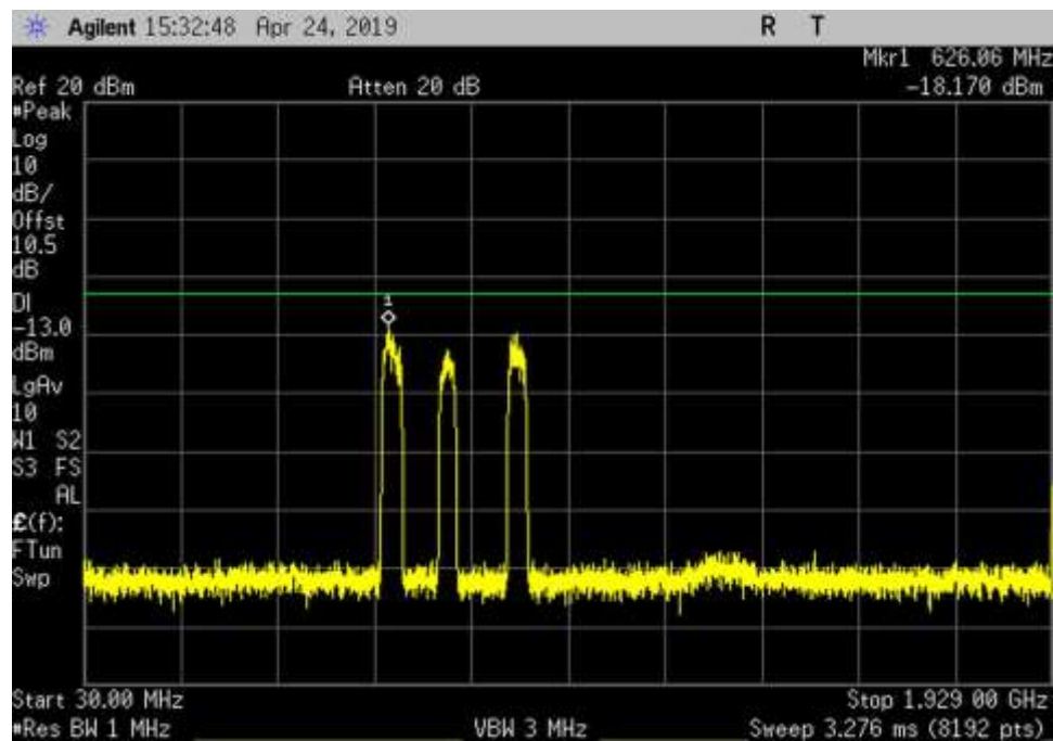
DL_1930-1995_AWGN_30- 1929MHz_MC
