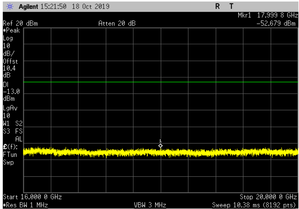
UL_1710-1755_GSM_16000-20000MHz_MC
