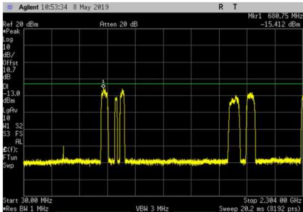
UL_2305-2315_GSM_30- 2304MHz_HC
