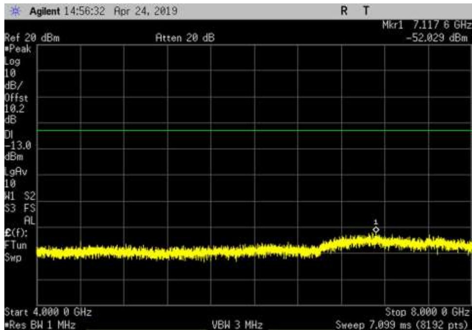
DL_746-757_GSM_4000- 8000MHz_HC
