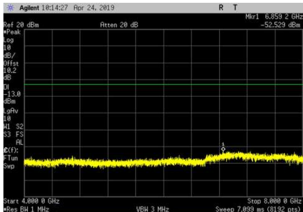
UL_663-698_GSM_4000-8000MHz_HC
