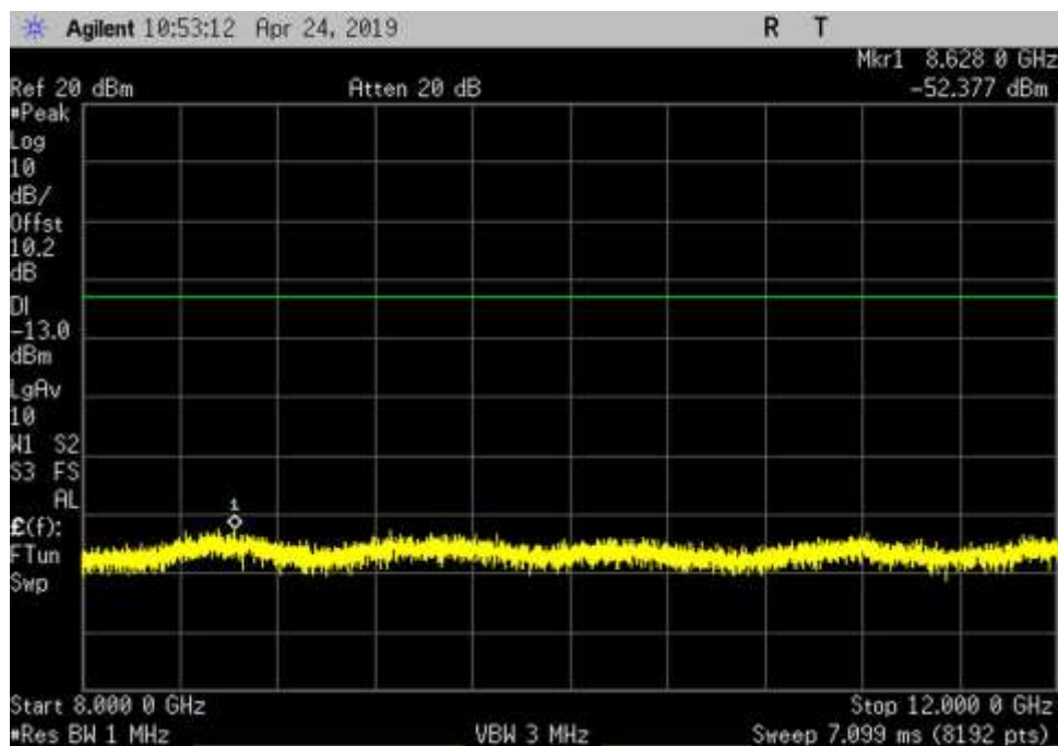
UL_824-849_GSM_8000- 12000MHz_LC
