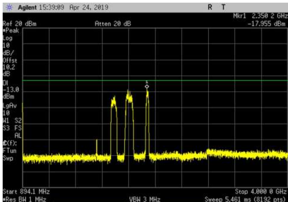
DL_869-894_AWGN_894.1-4000MHz_MC
