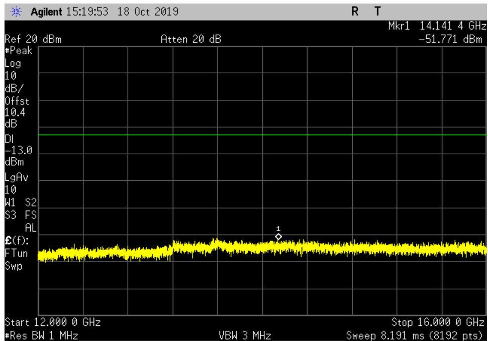
UL_1710-1755_GSM_12000- 16000MHz_LC
