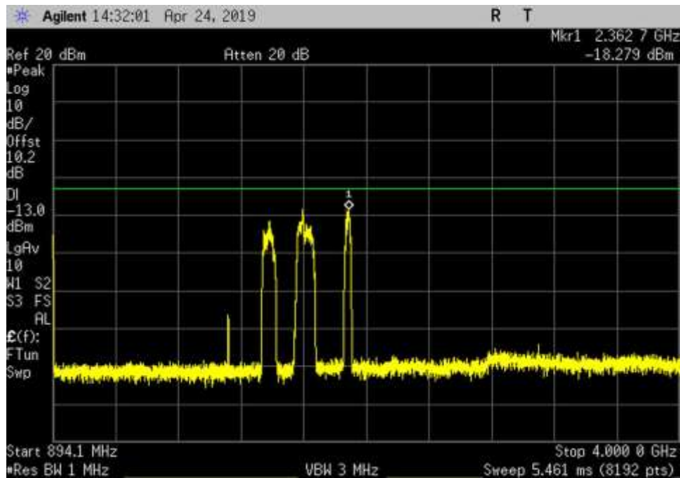
DL_869-894_GSM_894.1- 4000MHz_MC
