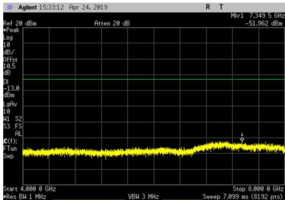
DL_1930-1995_AWGN_4000- 8000MHz_MC
