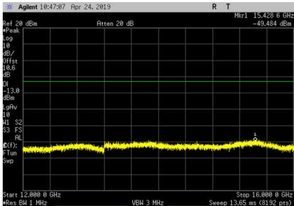
UL_1850-1915_GSM_12000- 16000MHz_HC
