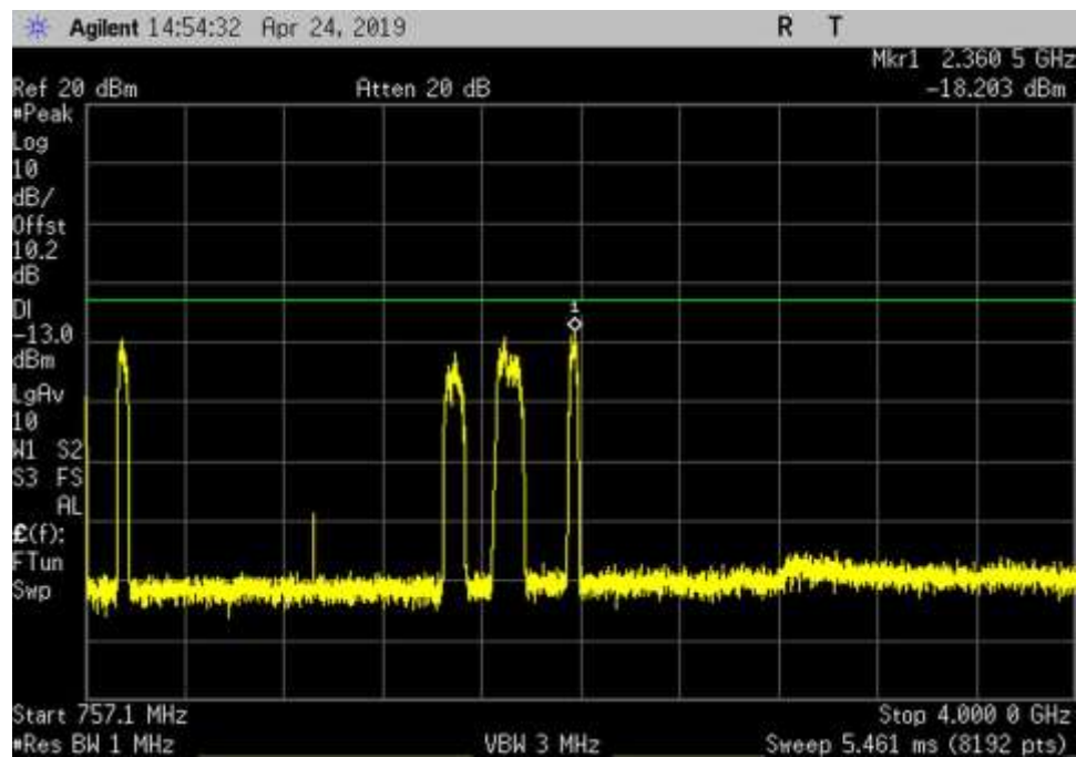
DL_746-757_GSM_757.1- 4000MHz_MC
