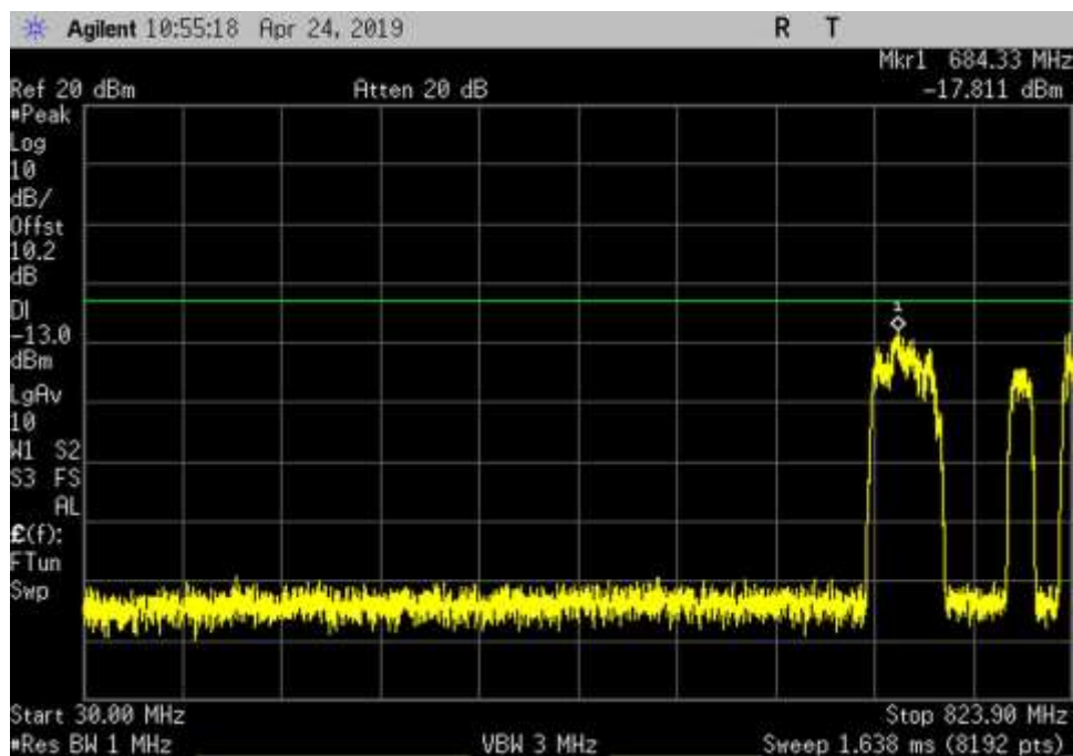
UL_824-849_GSM_30- 823.9MHz_HC
