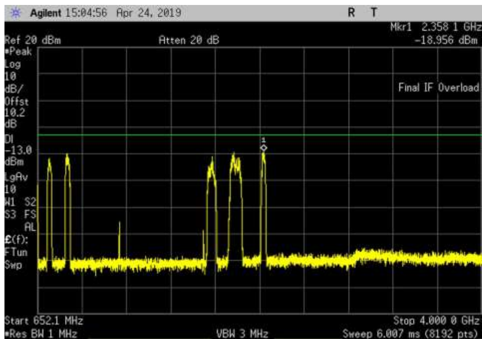
DL_617-652_GSM_652.1- 4000MHz_MC
