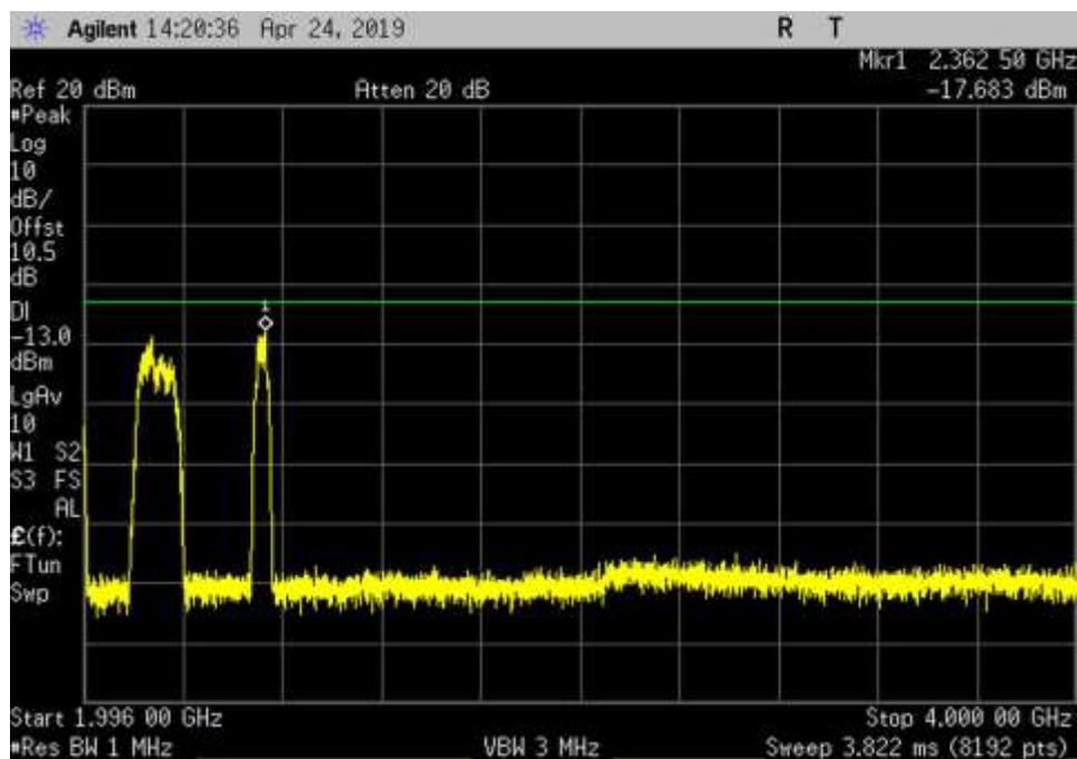
DL_1930-1995_GSM_ 1996- 4000MHz_LC
