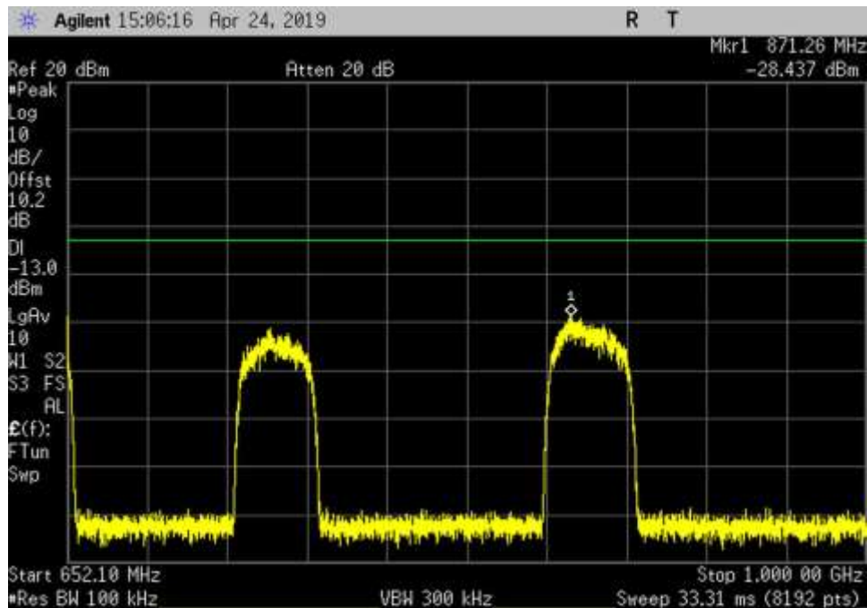
DL_617-652_GSM_ 652.1- 1000MHz_HC
