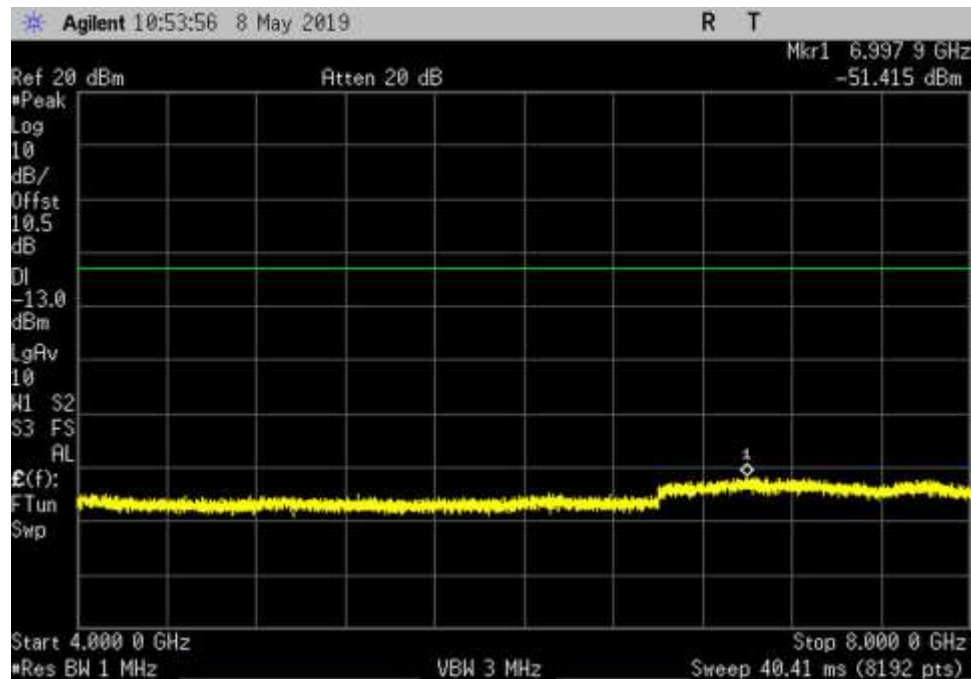
UL_2305-2315_GSM_4000-8000MHz_HC
