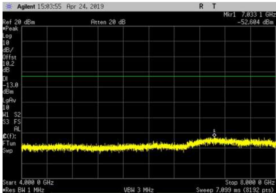
DL_617-652_GSM_4000- 8000MHz_LC
