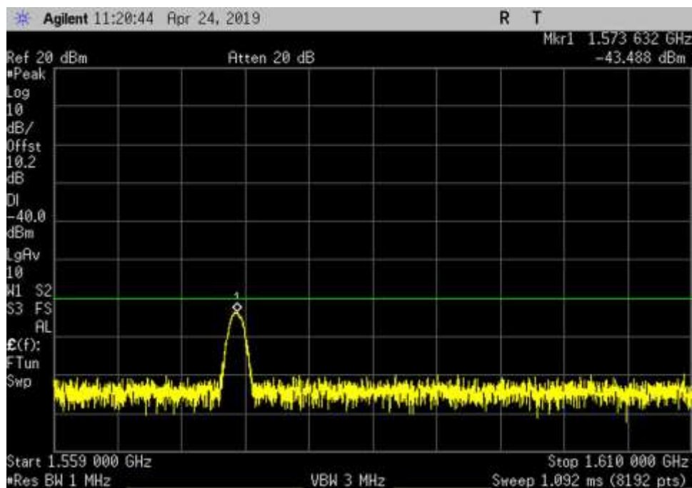
UL_776-787_GSM_1559-1610MHz_HC
