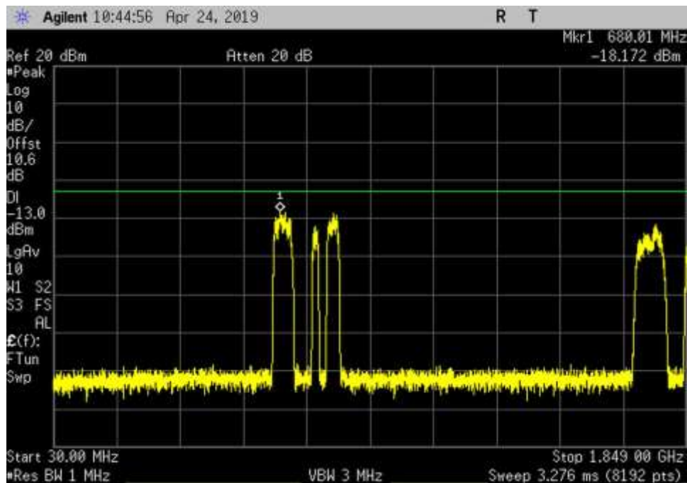
UL_1850-1915_GSM_30-1849MHz_MC
