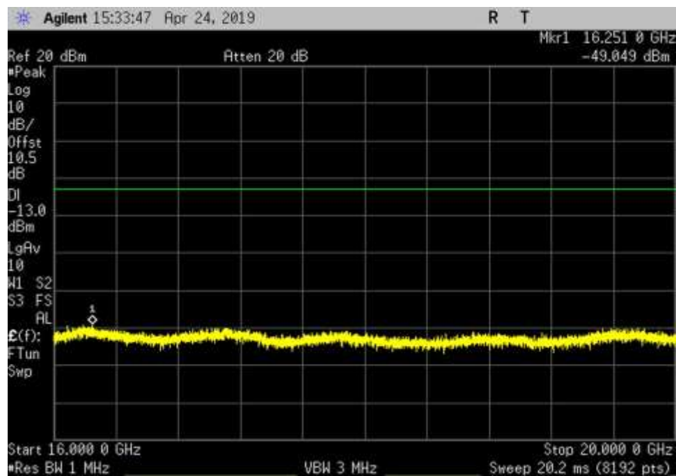
DL_1930-1995_AWGN_16000-20000MHz_MC
