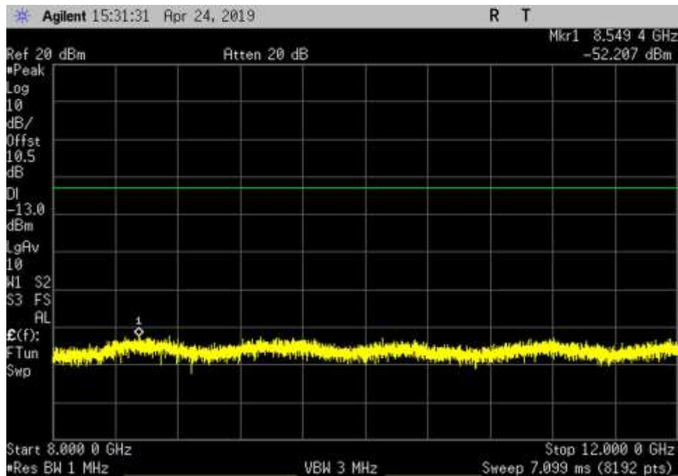
DL_1930-1995_AWGN_ 8000- 12000MHz_LC
