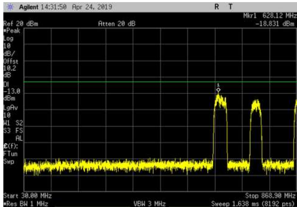
DL_869-894_GSM_30- 868.9MHz_MC
