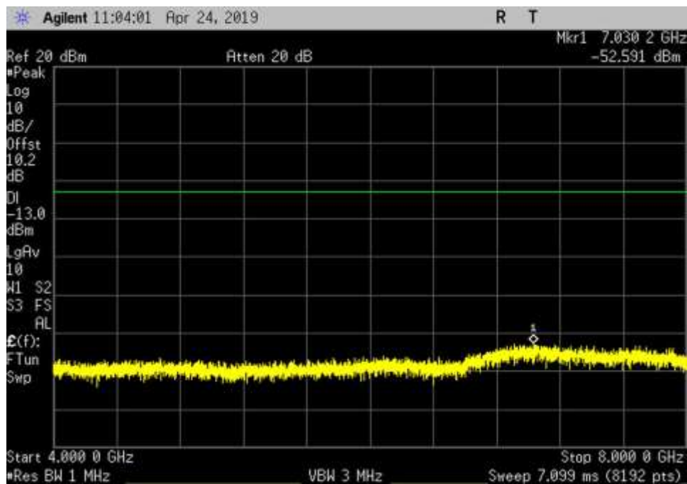
UL_698-716_GSM_4000-8000MHz_MC
