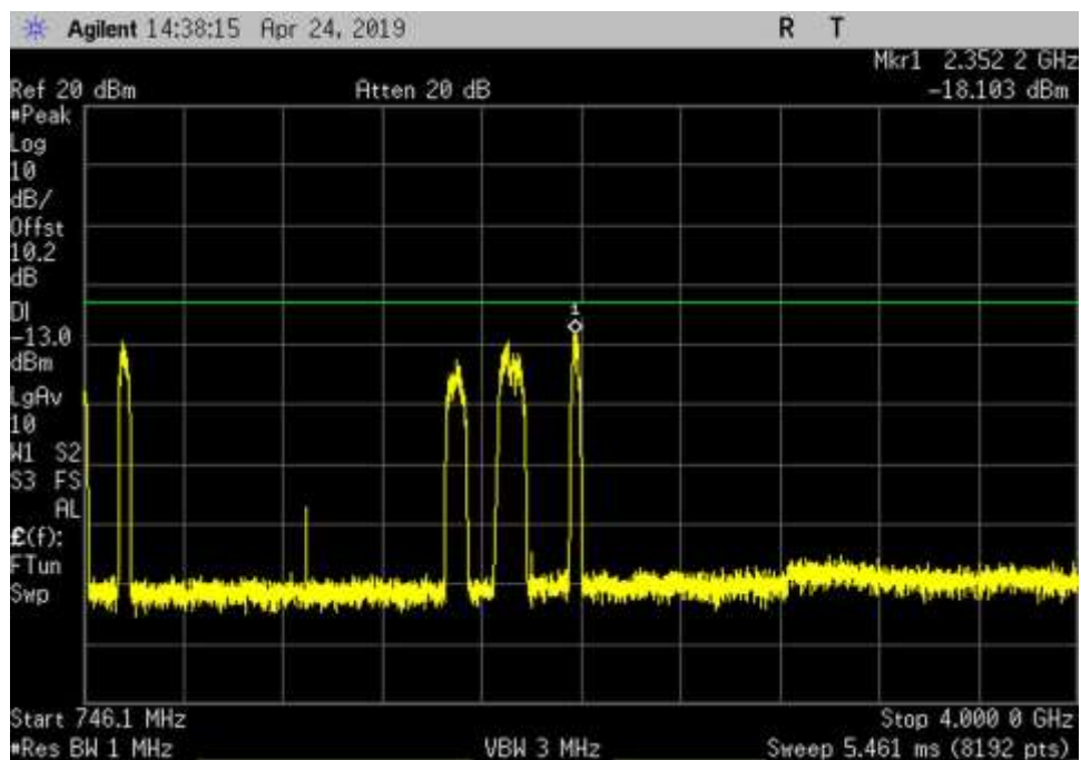
DL_728-746_GSM_746.1- 4000MHz_MC
