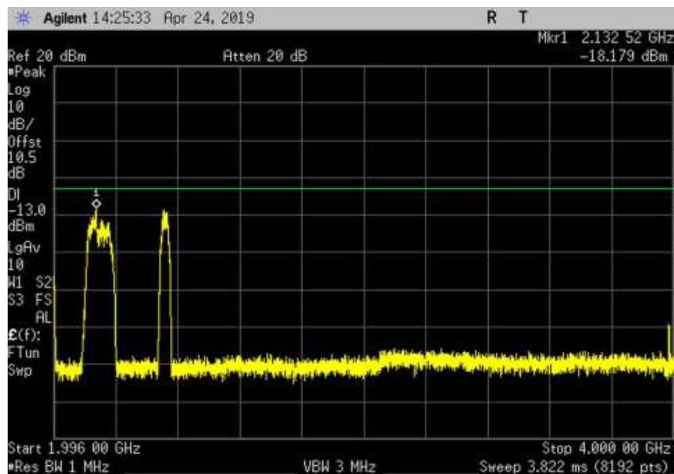
DL_1930-1995_GSM_1996-4000MHz_HC
