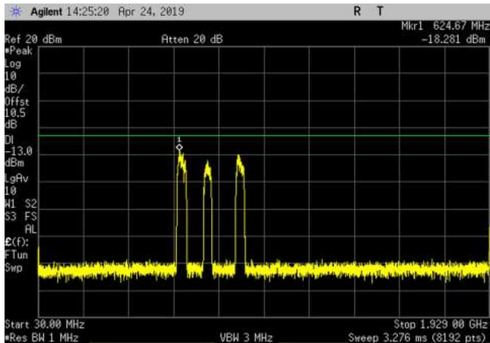
DL_1930-1995_GSM_ 30- 1929MHz_HC
