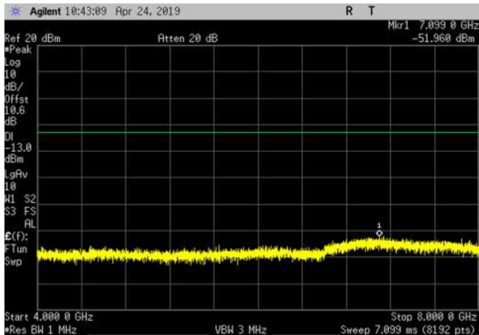
UL_1850-1915_GSM_4000-8000MHz_LC
