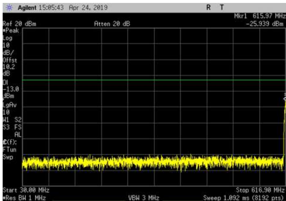
DL_617-652_GSM_30- 616.9MHz_HC
