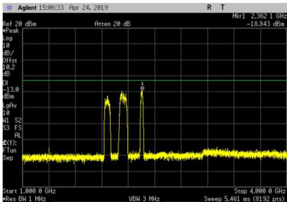
DL_617-652_GSM_ 1000- 4000MHz_HC
