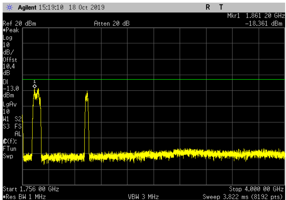
UL_1710-1755_GSM_1756- 4000MHz_LC
