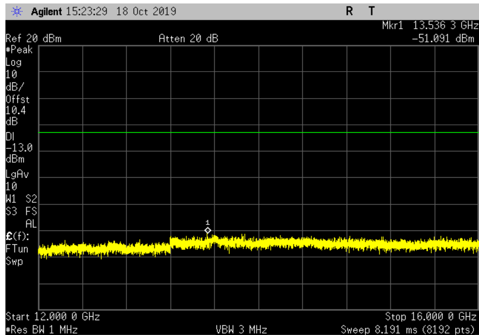
UL_1710-1755_GSM_12000- 16000MHz_HC
