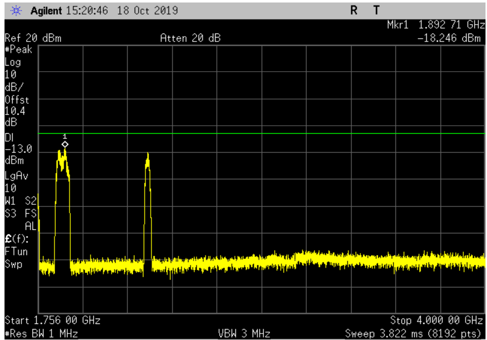
UL_1710-1755_GSM_1756- 4000MHz_MC
