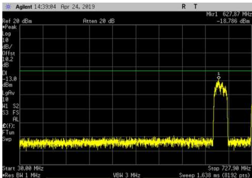
DL_728-746_GSM_30- 727.9MHz_HC
