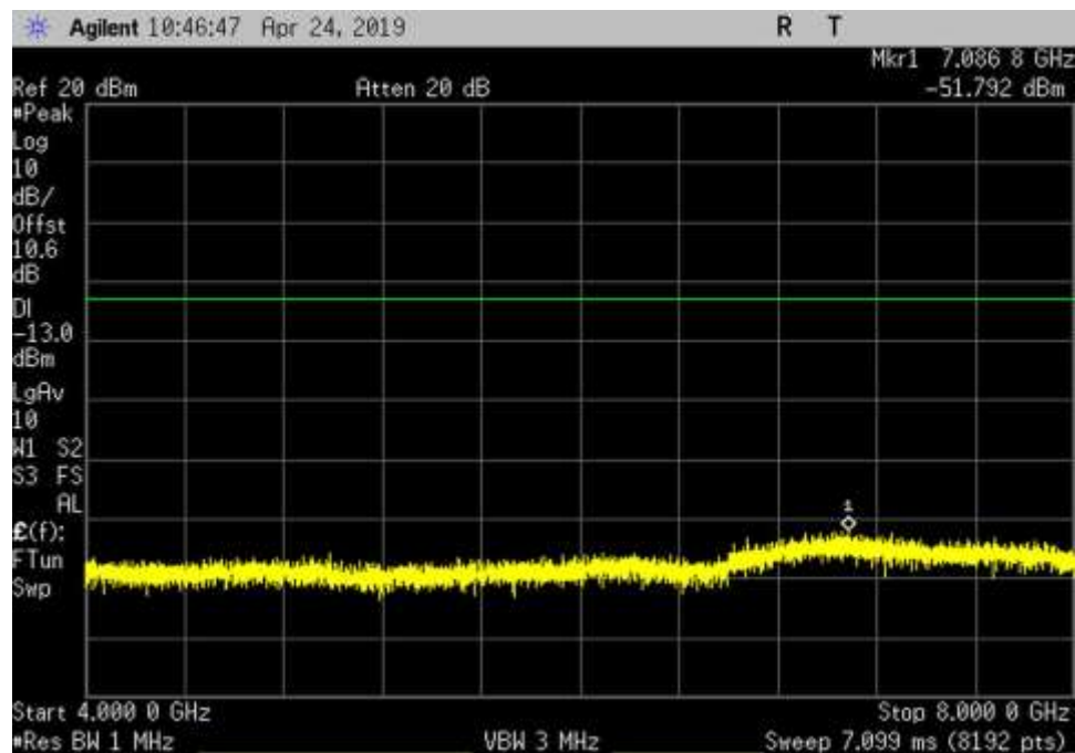
UL_1850-1915_GSM_4000-8000MHz_HC
