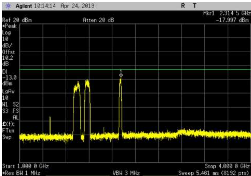
UL_663-698_GSM_1000- 4000MHz_HC
