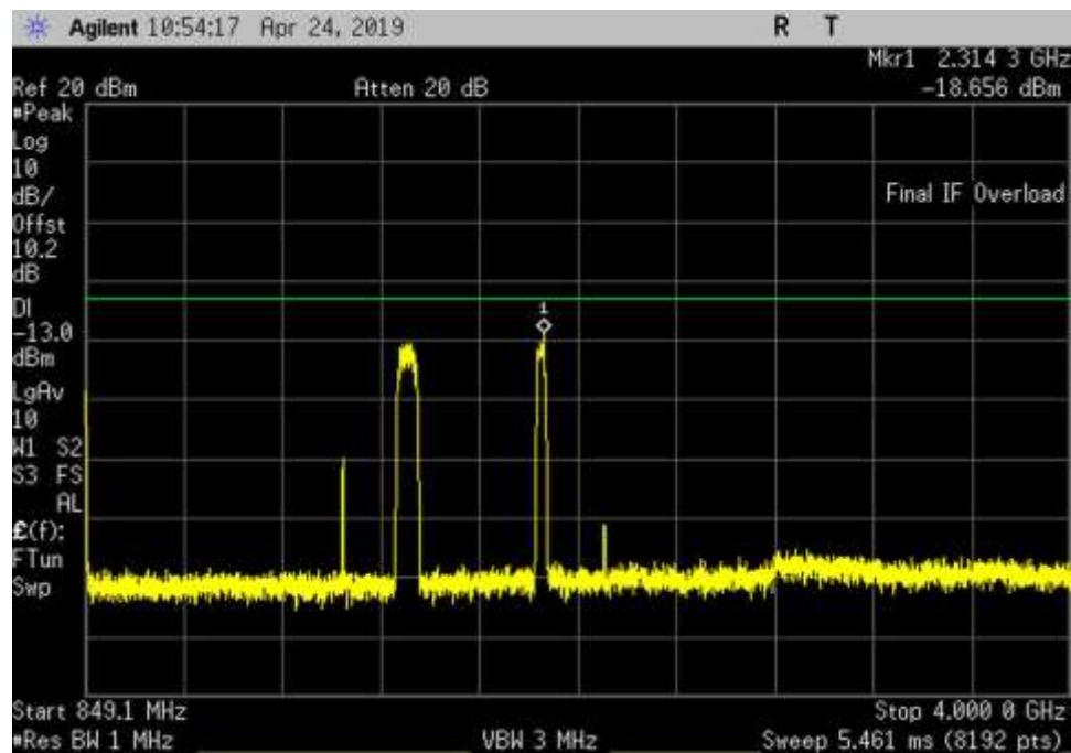
UL_824-849_GSM_849.1- 4000MHz_MC
