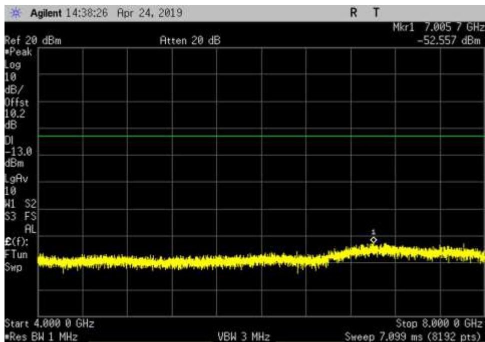
DL_728-746_GSM_4000-8000MHz_MC
