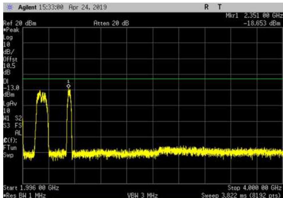
DL_1930-1995_AWGN_1996- 4000MHz_MC
