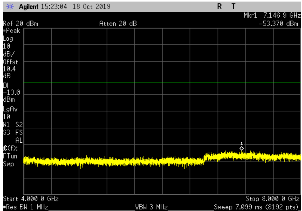
UL_1710-1755_GSM_4000-8000MHz_HC
