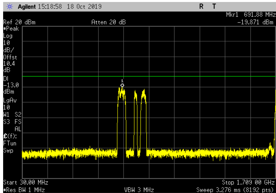
UL_1710-1755_GSM_30-1709MHz_LC
