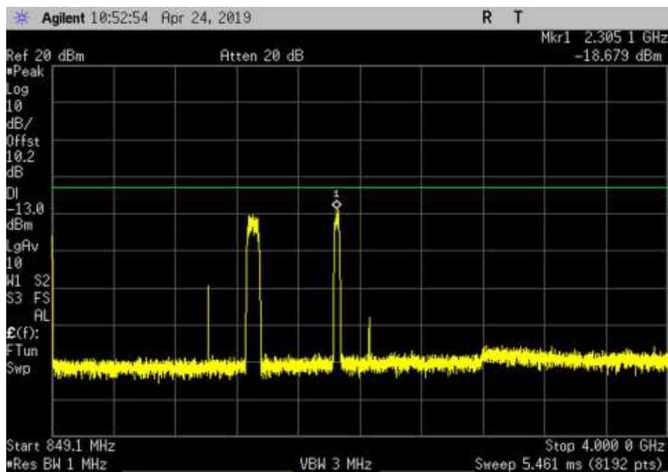
UL_824-849_GSM_849.1- 4000MHz_LC
