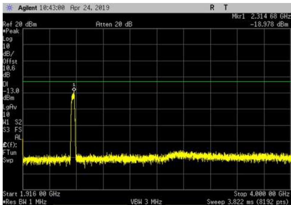
UL_1850-1915_GSM_1916-4000MHz_LC
