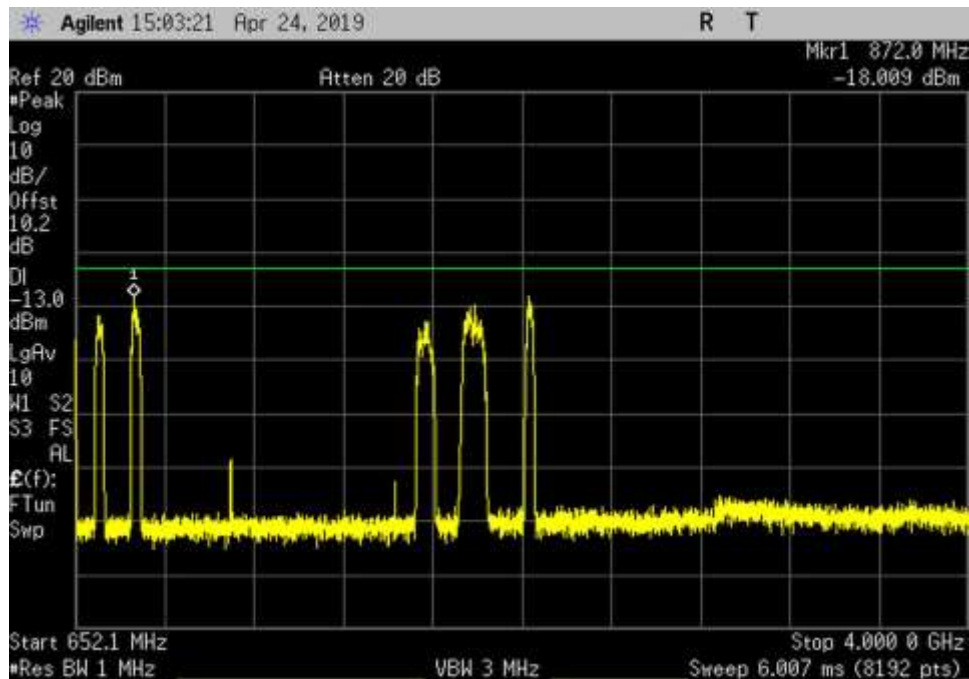
DL_617-652_GSM_652.1- 4000MHz_LC
