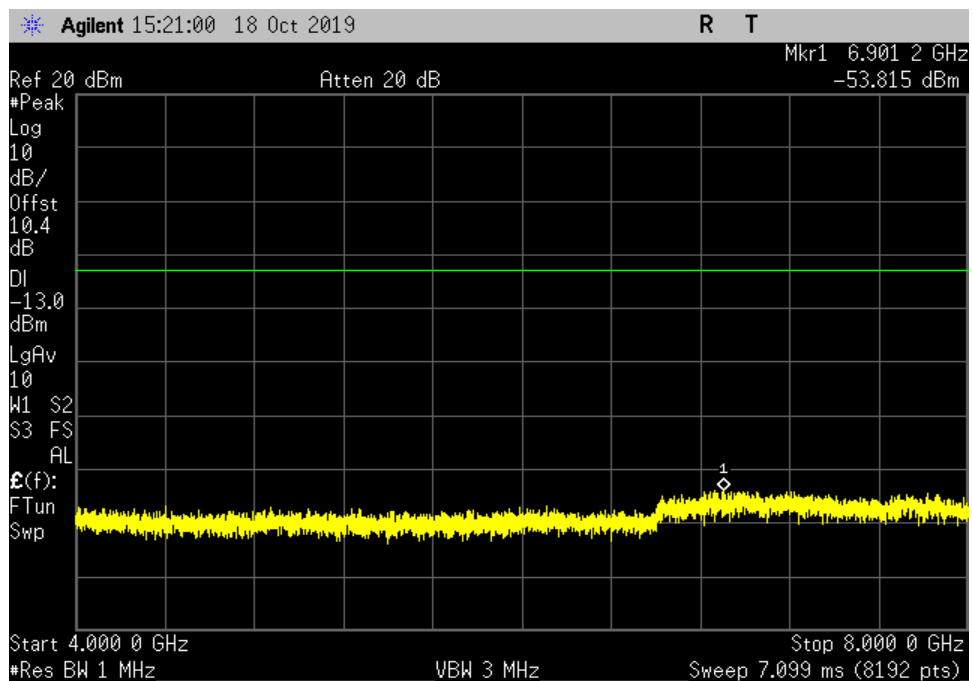
UL_1710-1755_GSM_4000- 8000MHz_MC
