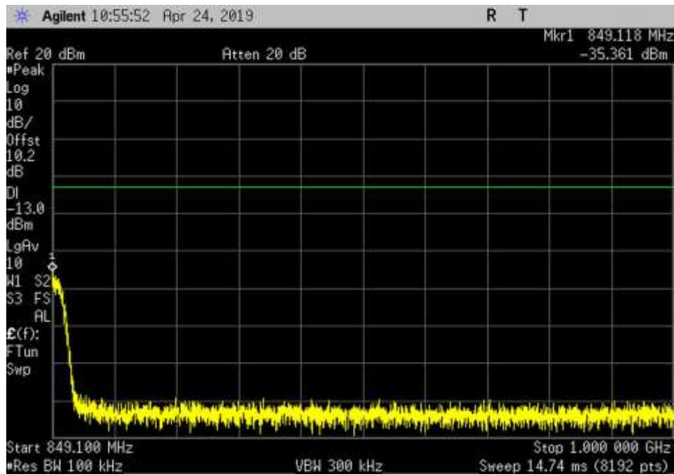
UL_824-849_GSM_849.1- 1000MHz_HC
