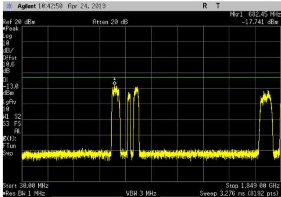
UL_1850-1915_GSM_30-1849MHz_LC
