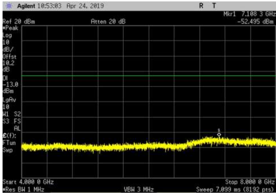
UL_824-849_GSM_4000-8000MHz_LC
