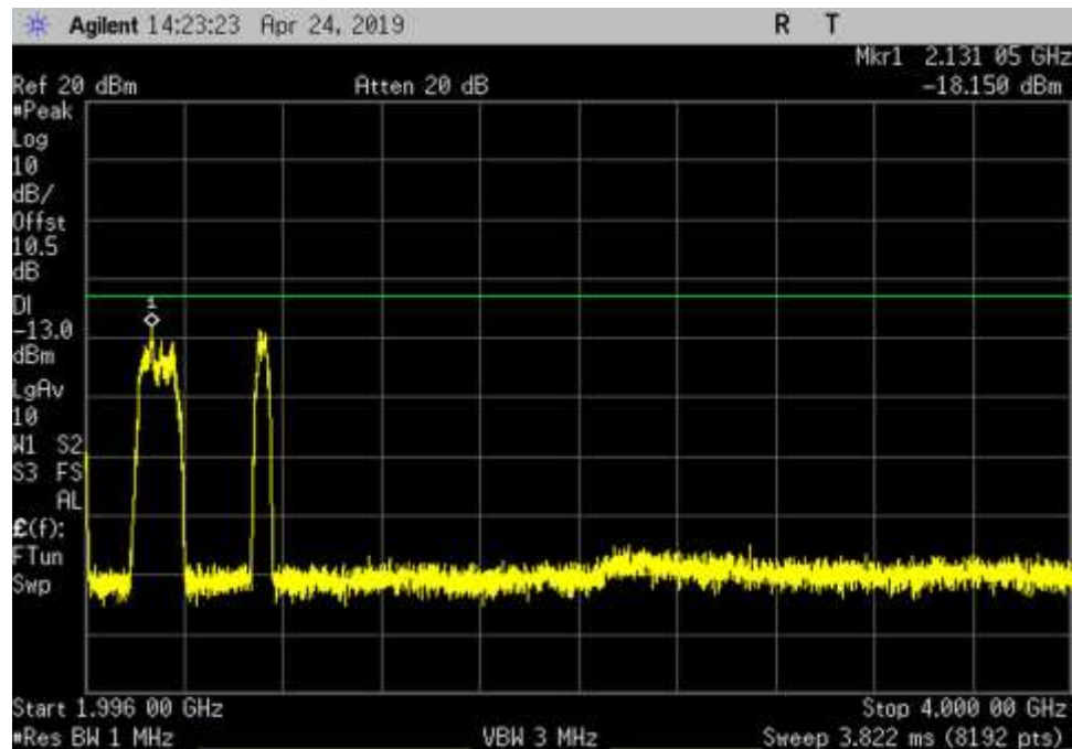
DL_1930-1995_GSM_1996-4000MHz_MC
