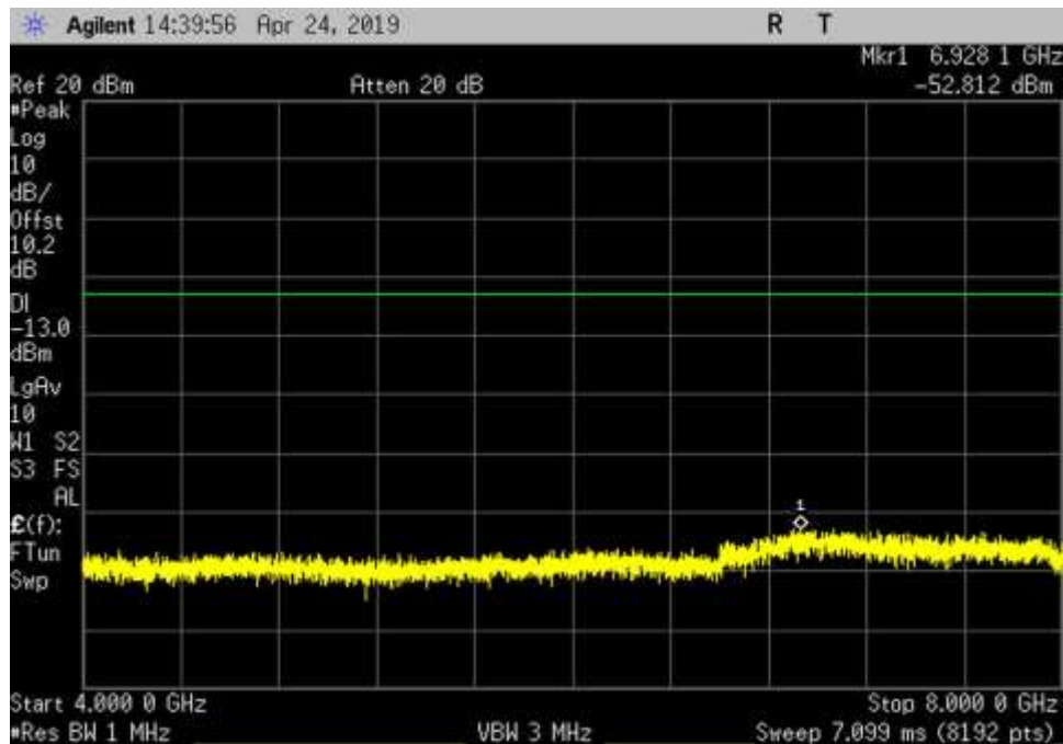
DL_728-746_GSM_4000- 8000MHz_HC
