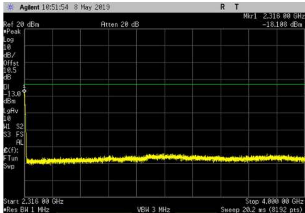
UL_2305-2315_GSM_2316- 4000MHz_MC
