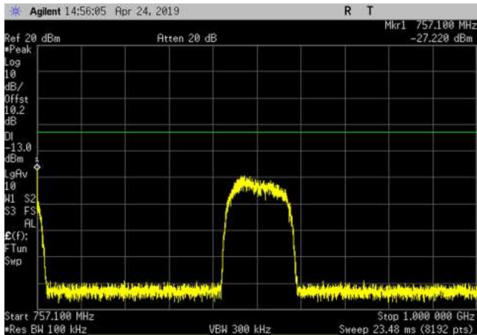
DL_746-757_GSM_757.1- 1000MHz_HC
