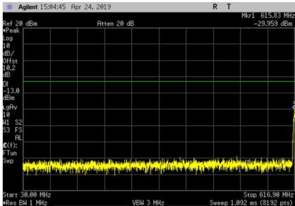
DL_617-652_GSM_30- 616.9MHz_MC
