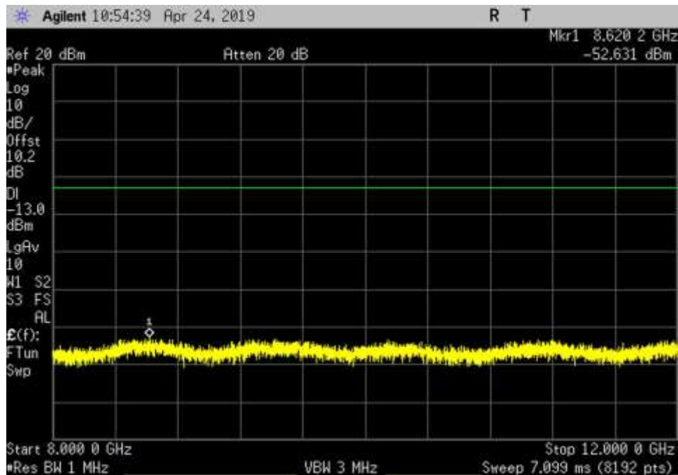
UL_824-849_GSM_8000-12000MHz_MC
