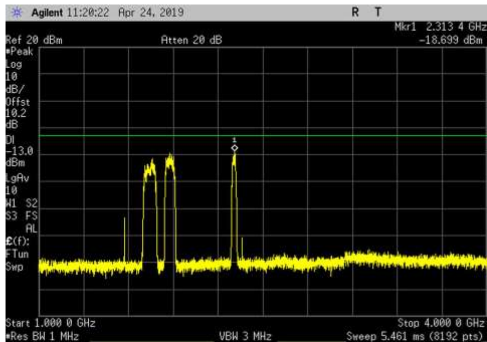
UL_776-787_GSM_1000- 4000MHz_HC
