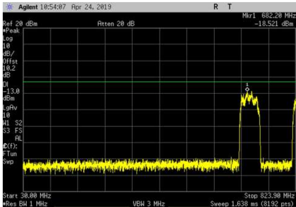
UL_824-849_GSM_30- 823.9MHz_MC
