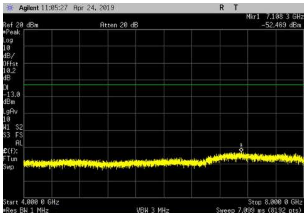
UL_698-716_GSM_4000-8000MHz_HC
