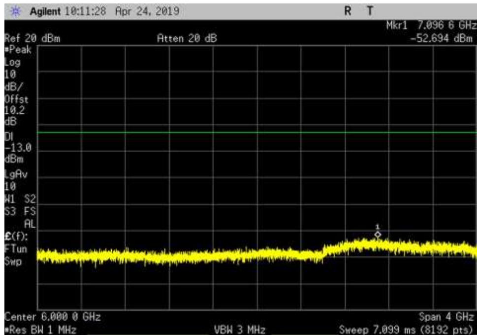
UL_663-698_GSM_4000- 8000MHz_LC
