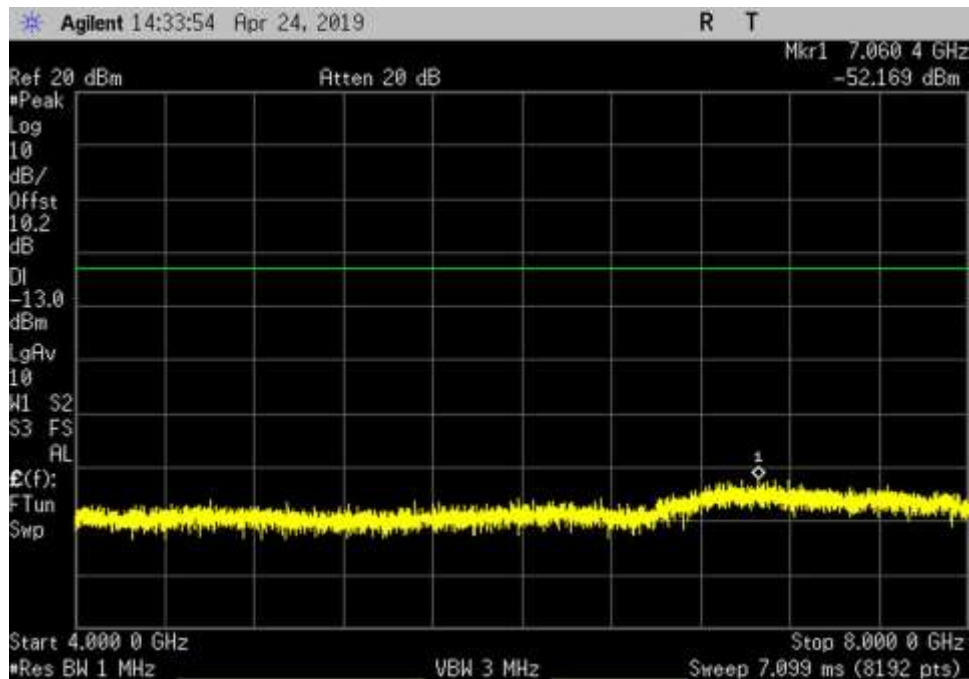
DL_869-894_GSM_4000- 8000MHz_HC
