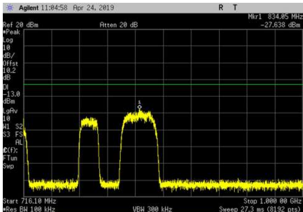
UL_698-716_GSM_716.1- 1000MHz_HC
