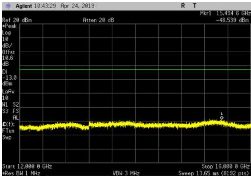
UL_1850-1915_GSM_12000- 16000MHz_LC
