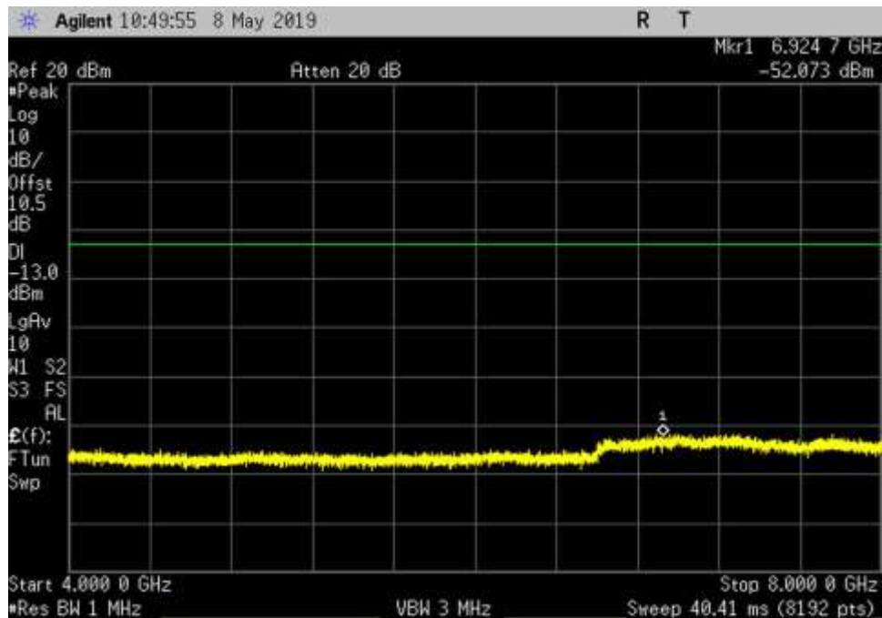
UL_2305-2315_GSM_4000-8000MHz_LC
