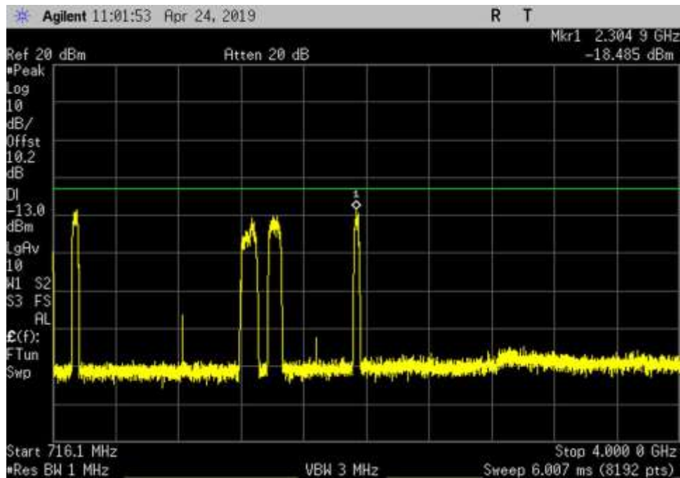
UL_698-716_GSM_716.1- 4000MHz_LC
