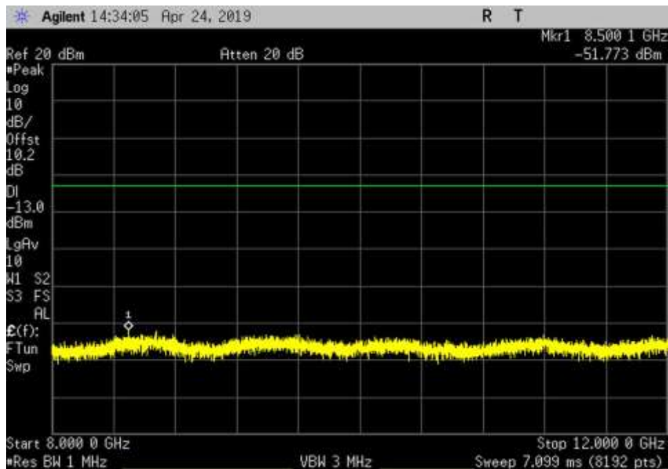
DL_869-894_GSM_8000-12000MHz_HC
