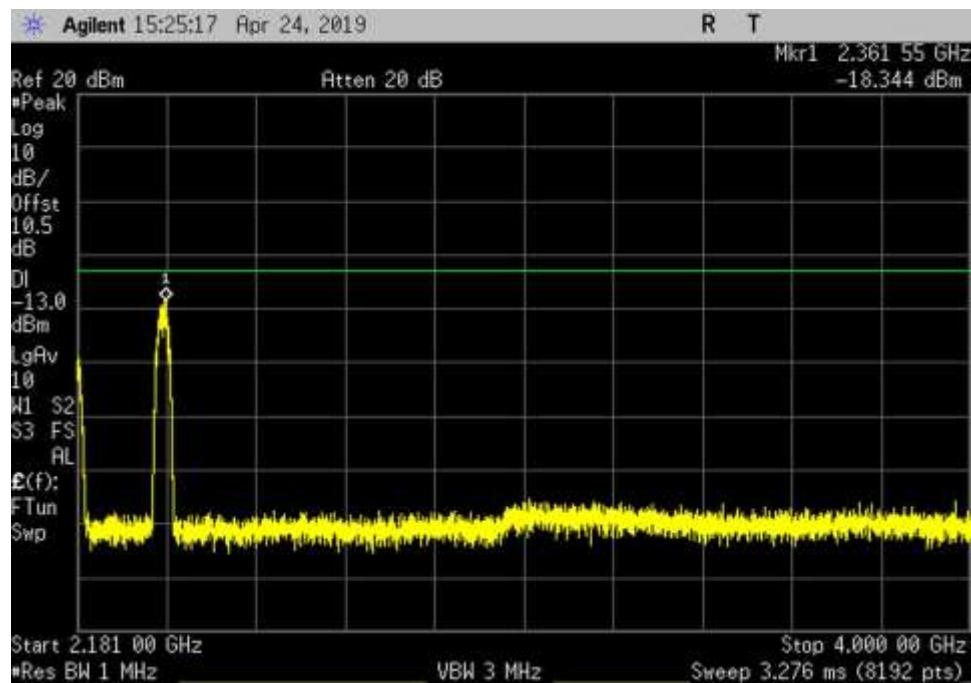
DL_2110-2155_AWGN_2181- 4000MHz_LC
