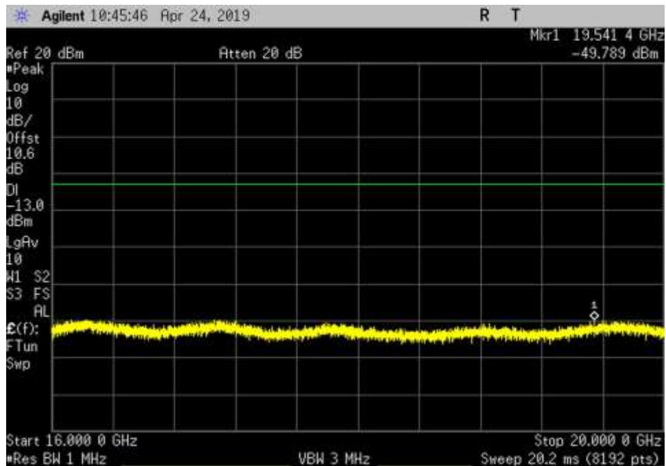
UL_1850-1915_GSM_16000-20000MHz_MC
