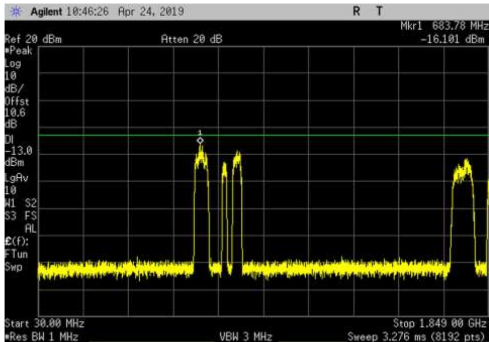
UL_1850-1915_GSM_30-1849MHz_HC
