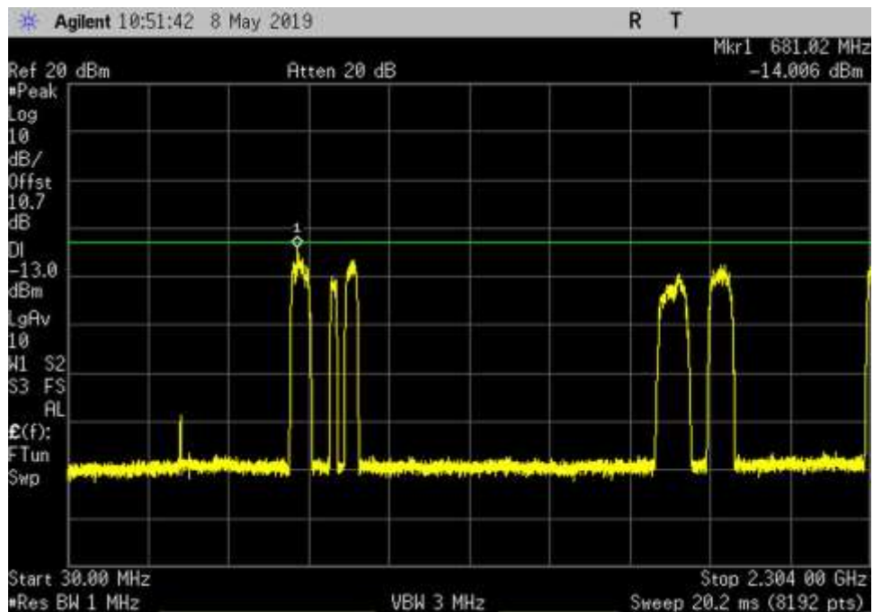
UL_2305-2315_GSM_30- 2304MHz_MC
