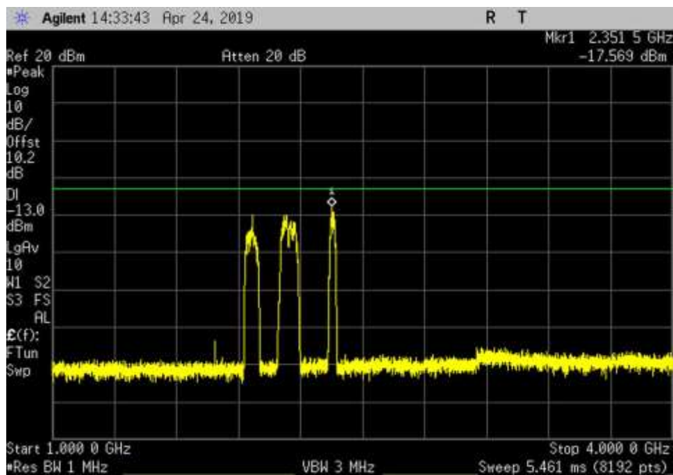
DL_869-894_GSM_1000- 4000MHz_HC
