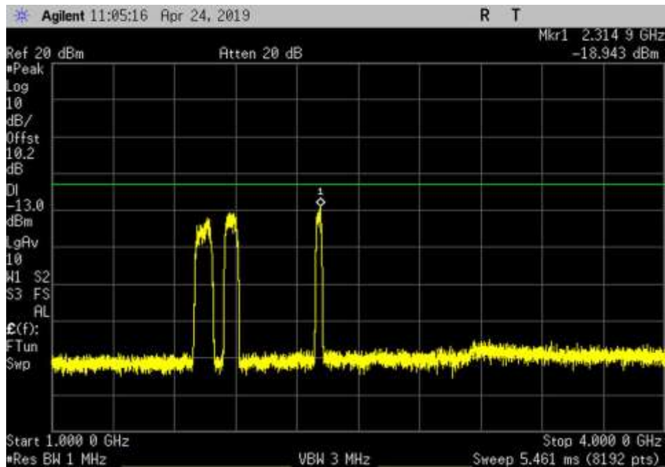
UL_698-716_GSM_1000- 4000MHz_HC
