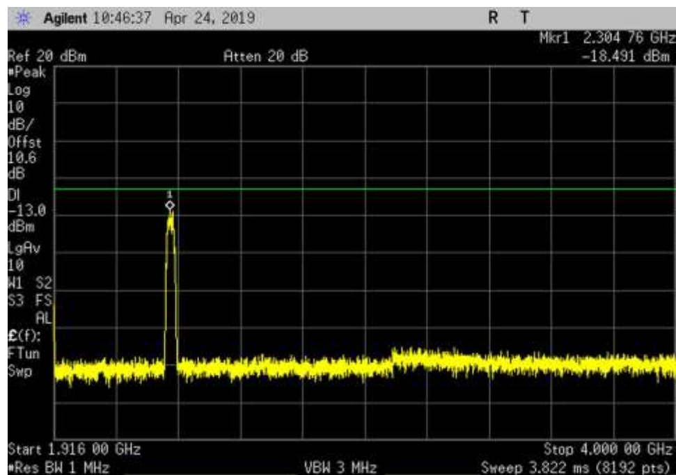
UL_1850-1915_GSM_1916- 4000MHz_HC
