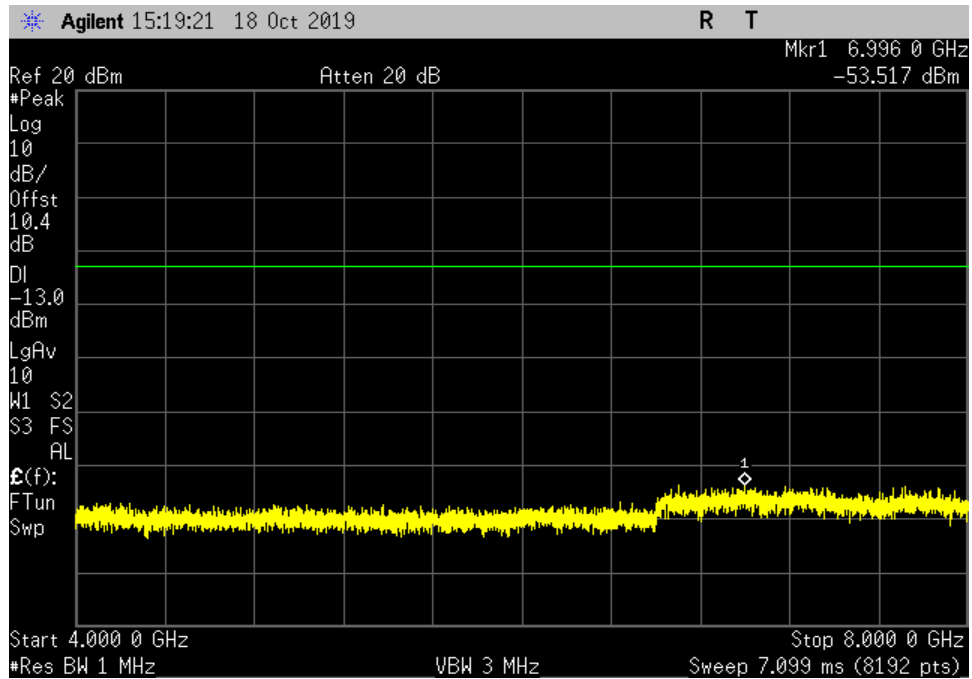
UL_1710-1755_GSM_4000- 8000MHz_LC
