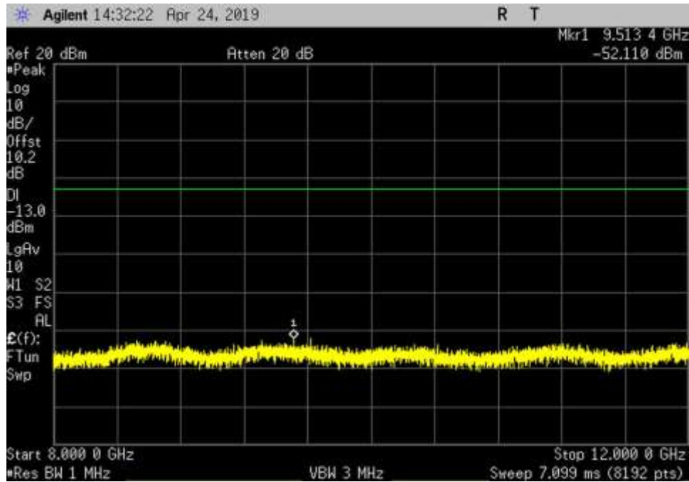
DL_869-894_GSM_8000-12000MHz_MC
