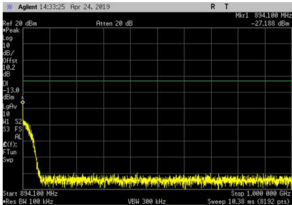
DL_869-894_GSM_ 894.1- 1000MHz_HC
