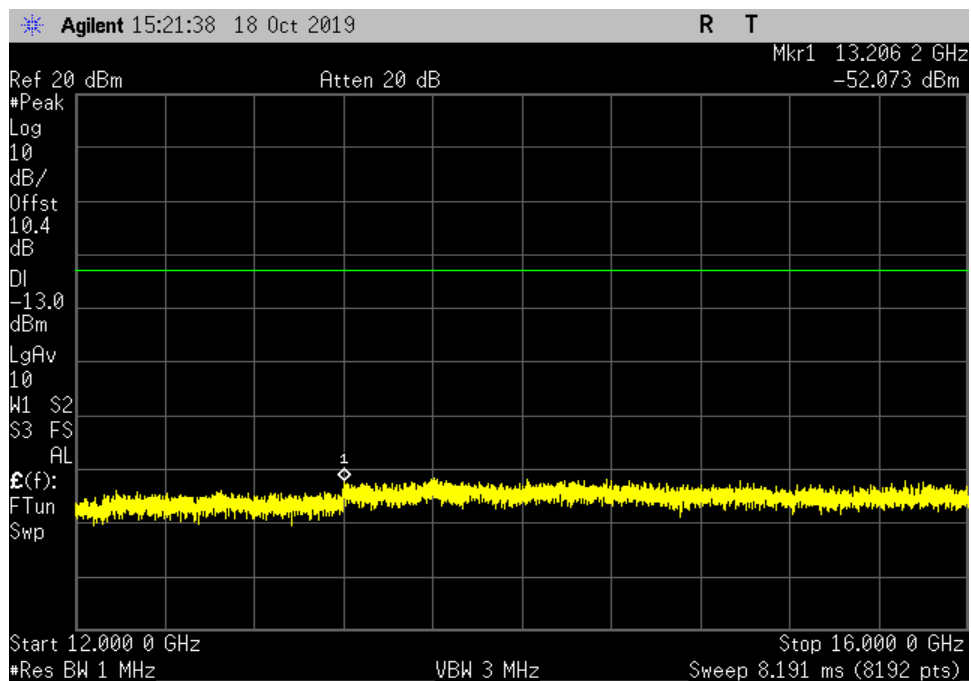
UL_1710-1755_GSM_12000- 16000MHz_MC
