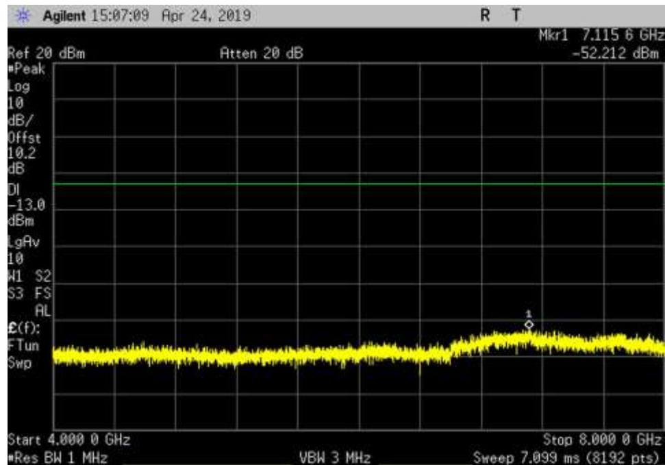
DL_617-652_GSM_4000- 8000MHz_HC
