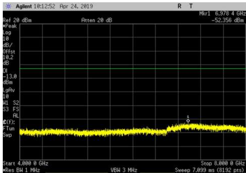
UL_663-698_GSM_4000-8000MHz_MC
