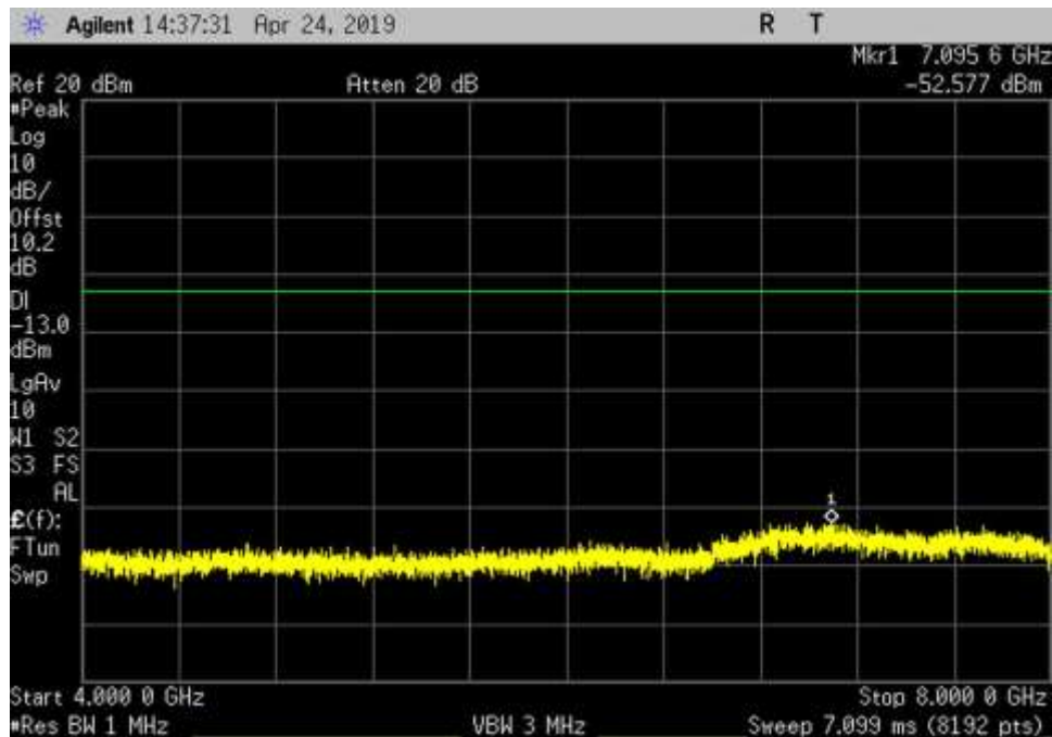
DL_728-746_GSM_4000-8000MHz_LC
