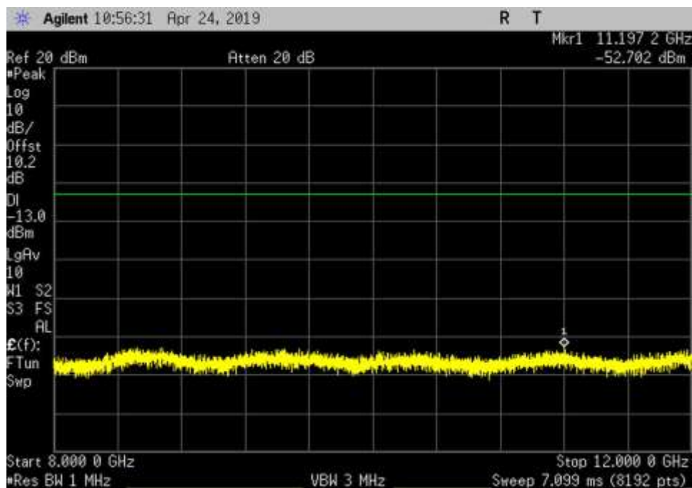
UL_824-849_GSM_8000-12000MHz_HC
