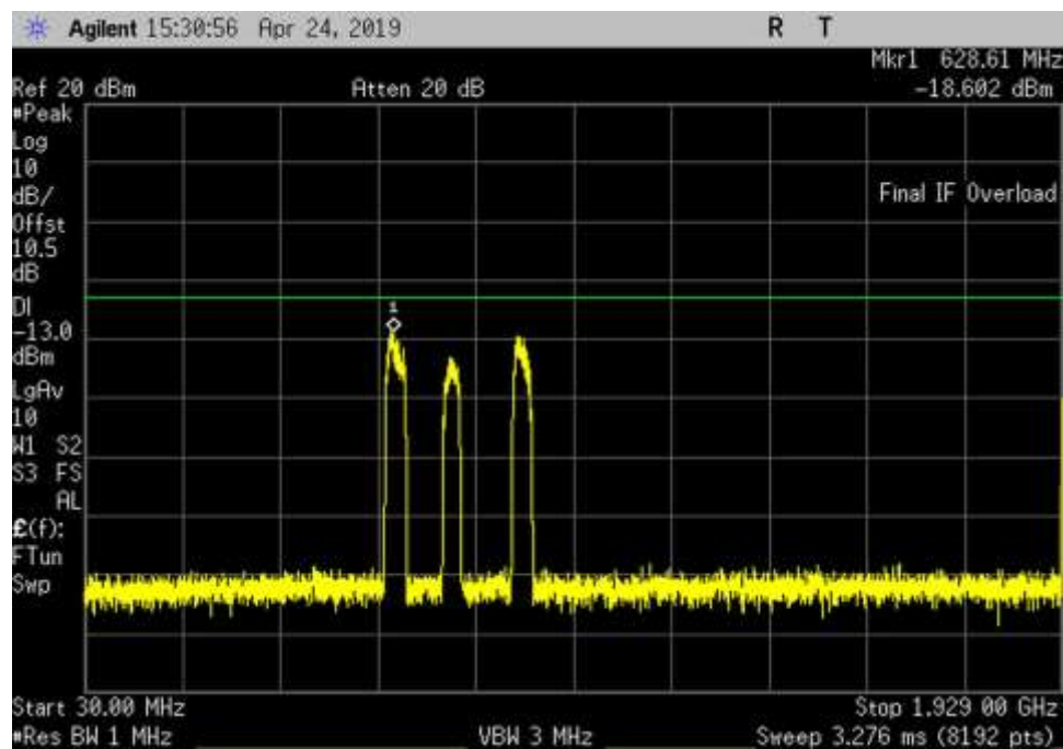
DL_1930-1995_AWGN_30-1929MHz_LC
