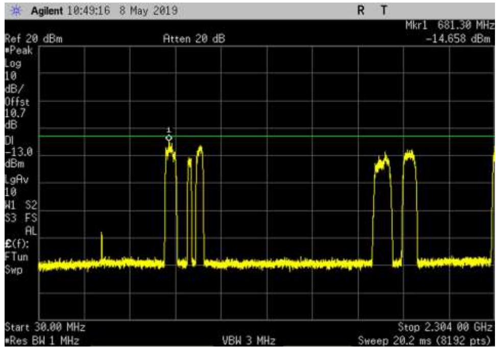
UL_2305-2315_GSM_30- 2304MHz_LC
