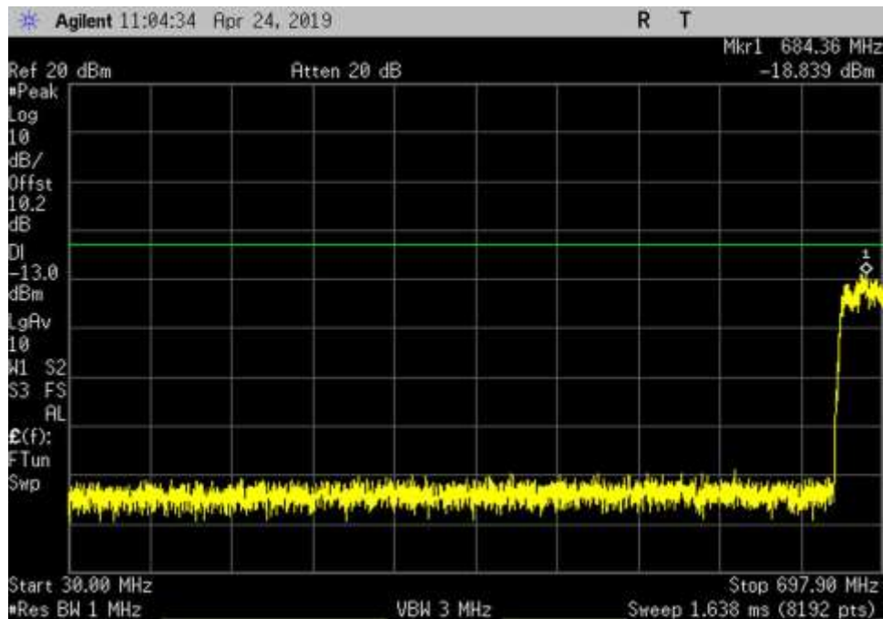
UL_698-716_GSM_30- 697.9MHz_HC
