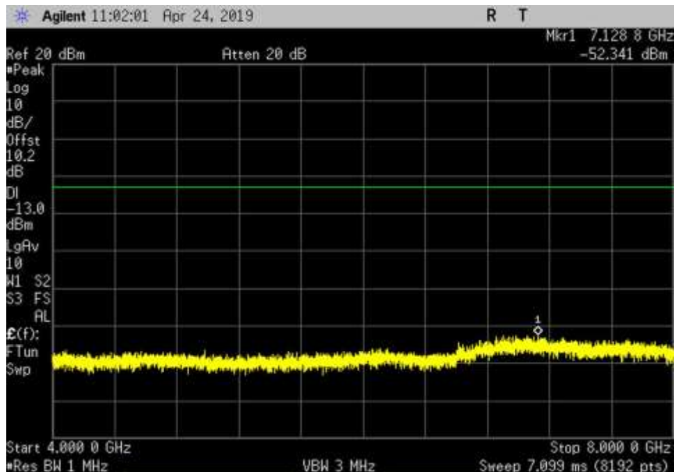
UL_698-716_GSM_4000- 8000MHz_LC
