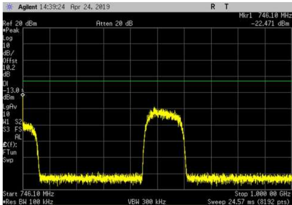
DL_728-746_GSM_746.1- 1000MHz_HC
