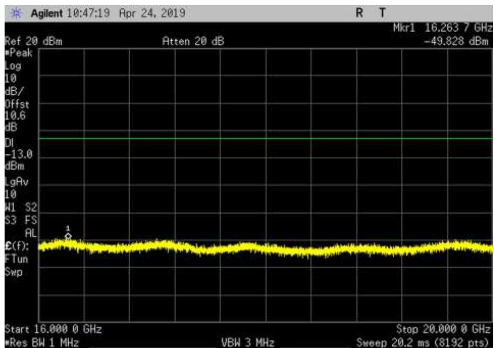
UL_1850-1915_GSM_16000-20000MHz_HC
