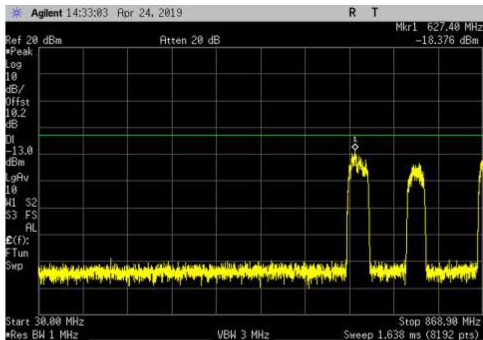
DL_869-894_GSM_30- 868.9MHz_HC
