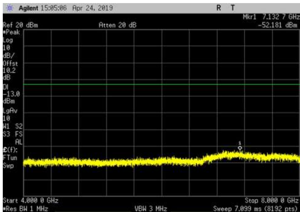
DL_617-652_GSM_4000- 8000MHz_MC
