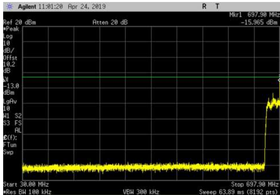
UL_698-716_GSM_30- 697.9MHz_LC
