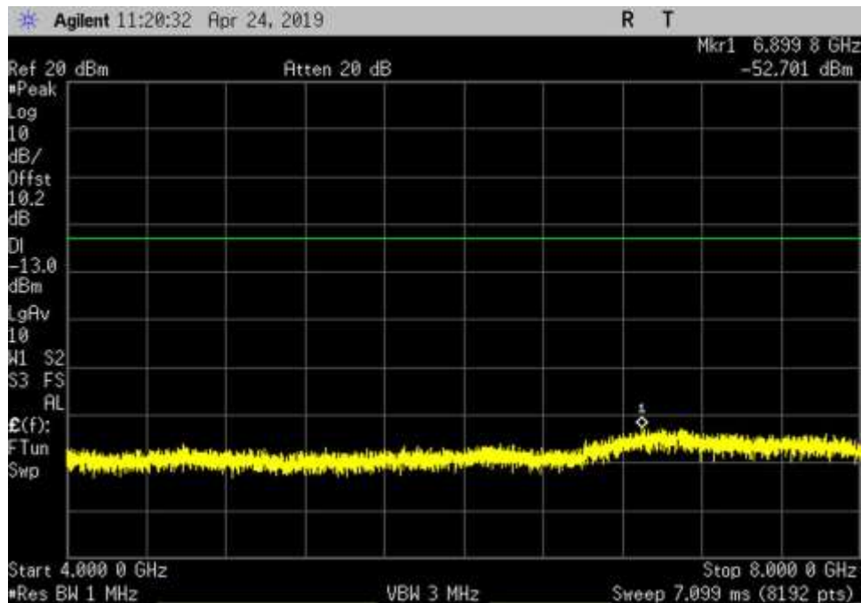
UL_776-787_GSM_4000- 8000MHz_HC
