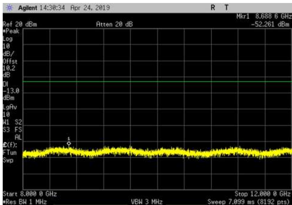
DL_869-894_GSM_8000- 12000MHz_LC
