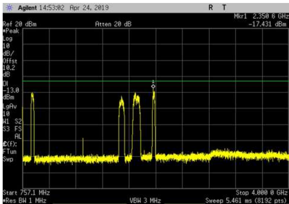
DL_746-757_GSM_757.1- 4000MHz_LC
