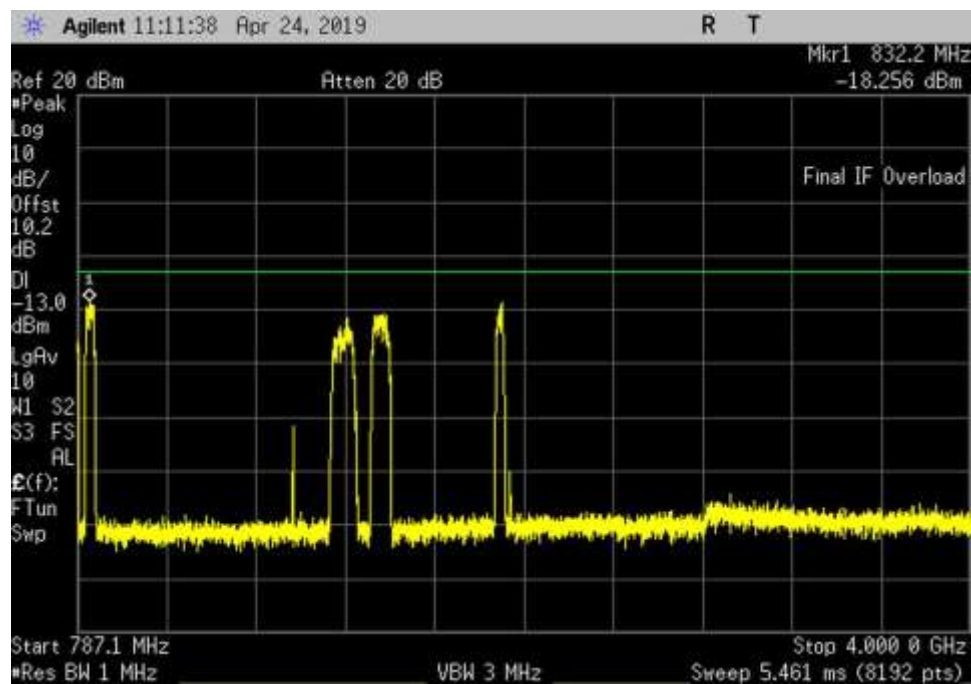
UL_776-787_GSM_787.1- 4000MHz_MC
