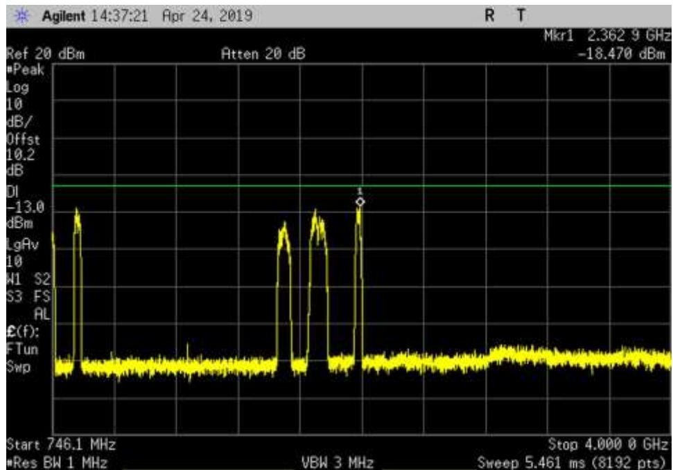
DL_728-746_GSM_746.1- 4000MHz_LC
