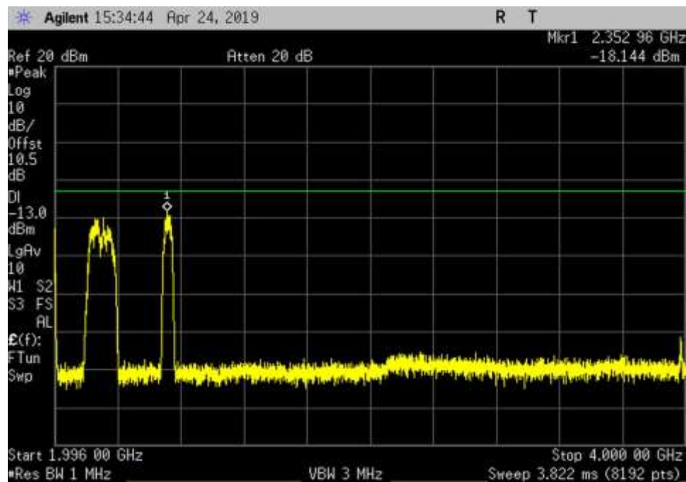
DL_1930-1995_AWGN_1996- 4000MHz_HC
