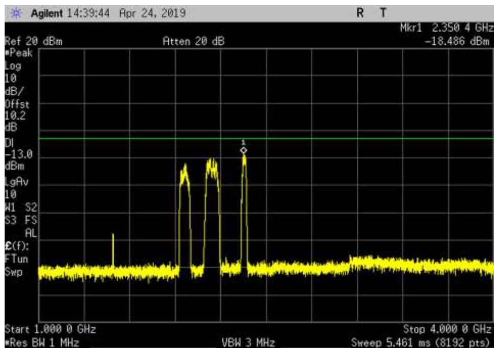
DL_728-746_GSM_1000- 4000MHz_HC
