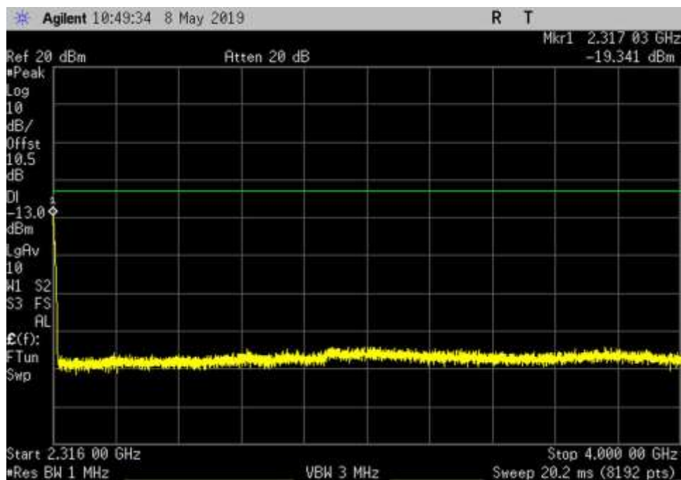
UL_2305-2315_GSM_2316- 4000MHz_LC
