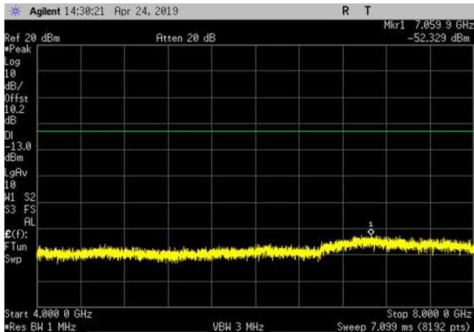
DL_869-894_GSM_4000-8000MHz_LC
