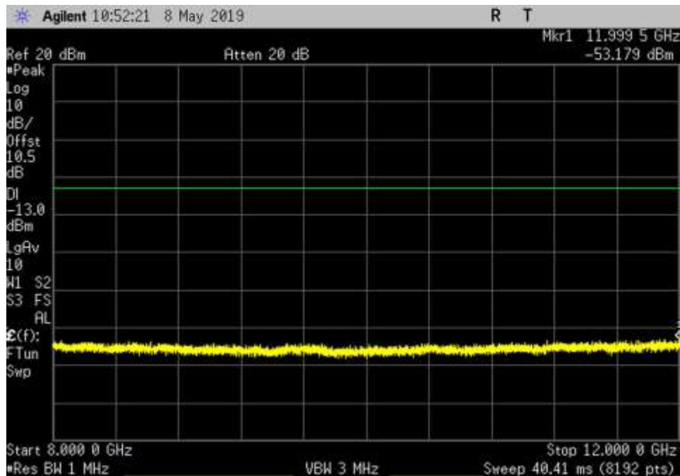
UL_2305-2315_GSM_8000-12000MHz_MC
