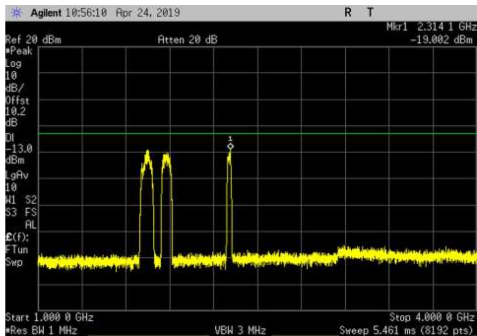
UL_824-849_GSM_1000- 4000MHz_HC
