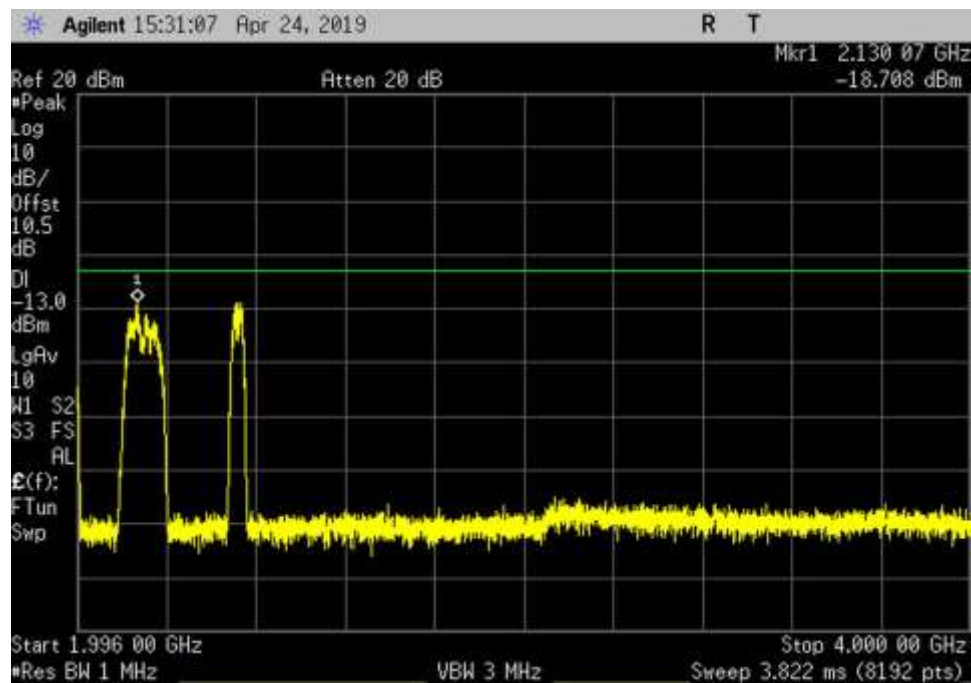
DL_1930-1995_AWGN_1996- 4000MHz_LC
