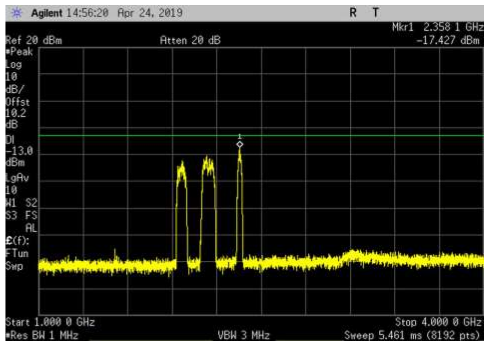
DL_746-757_GSM_1000- 4000MHz_HC
