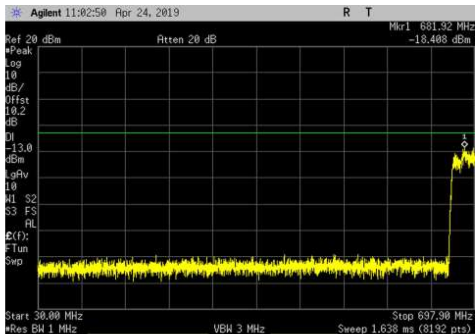
UL_698-716_GSM_30- 697.9MHz_MC
