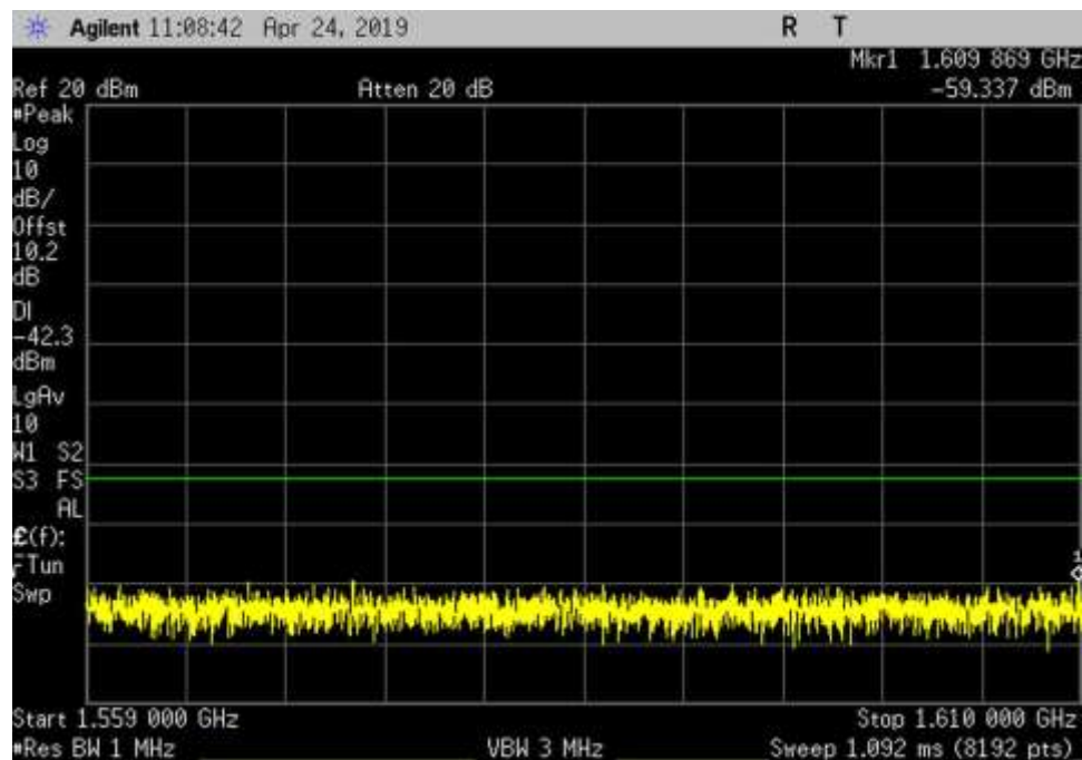
UL_776-787_GSM_1559- 1610MHz_LC
