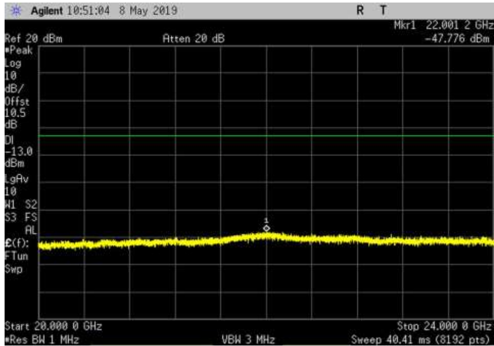
UL_2305-2315_GSM_20000-24000MHz_LC
