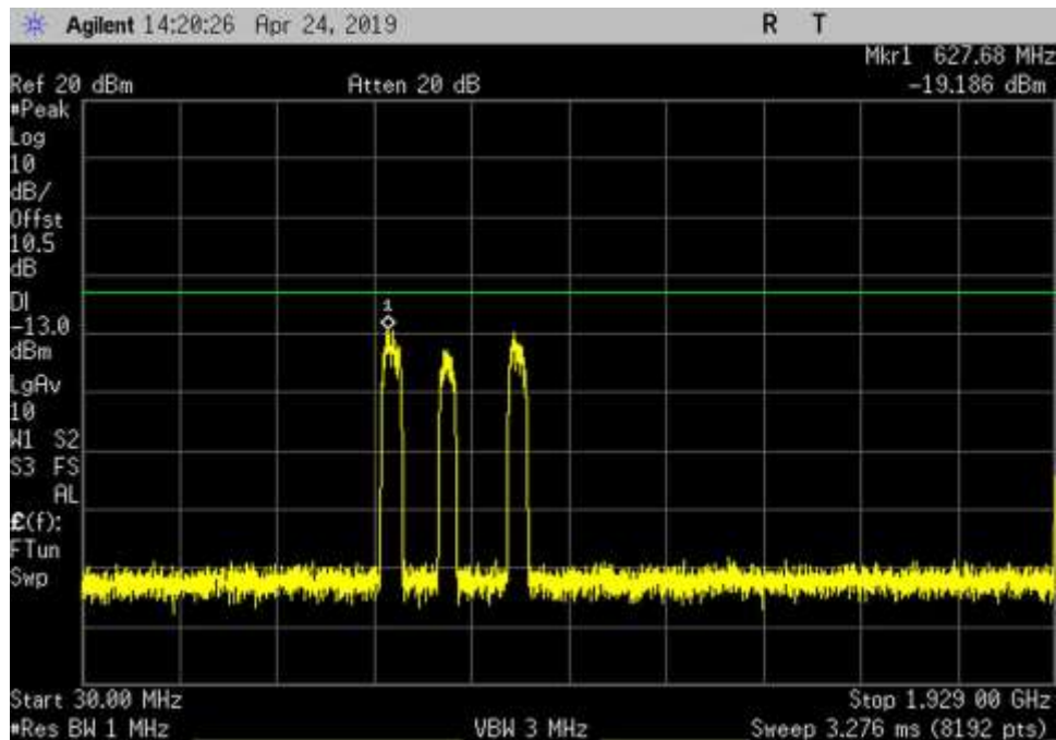
DL_1930-1995_GSM_30-1929MHz_LC
