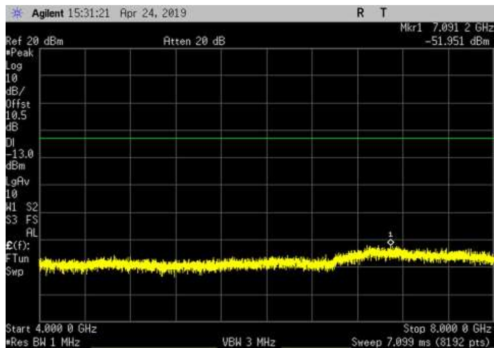
DL_1930-1995_AWGN_ 4000- 8000MHz_LC
