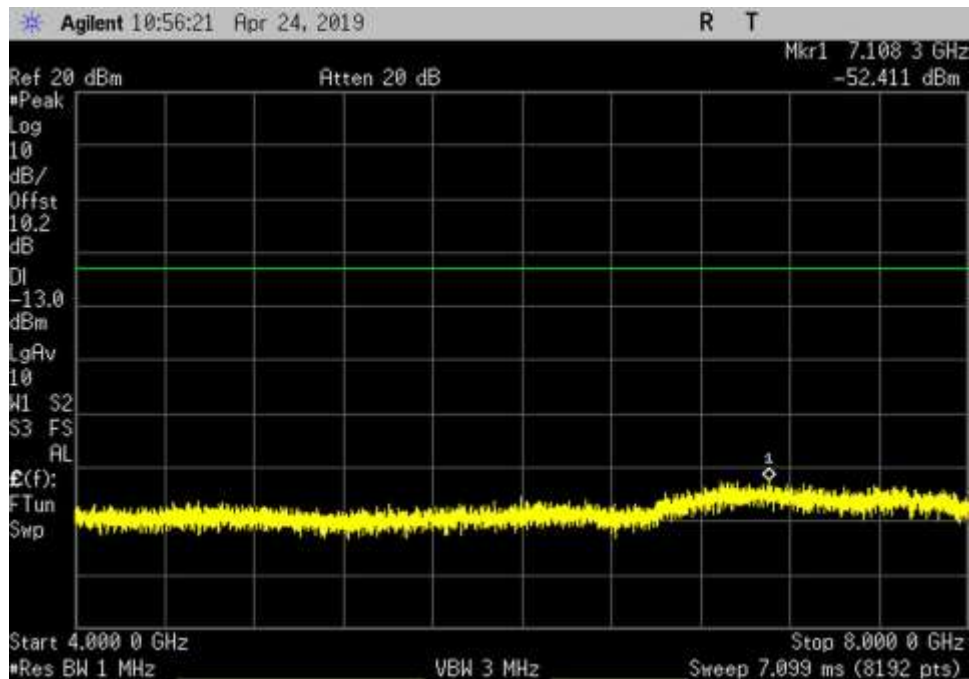
UL_824-849_GSM_4000- 8000MHz_HC
