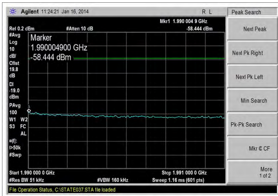
DL_1930-1995MHz_CDMA_H_-57dBm
