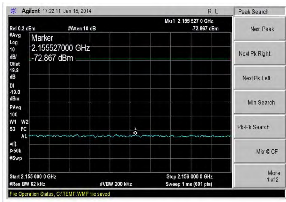
DL_2110-2155MHz_LTE_H_-20dBm
