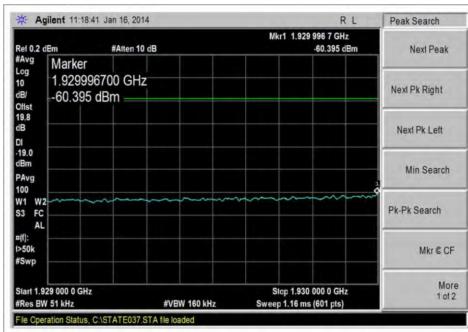
DL_1930-1995MHz_CDMA_L_-60dBm
