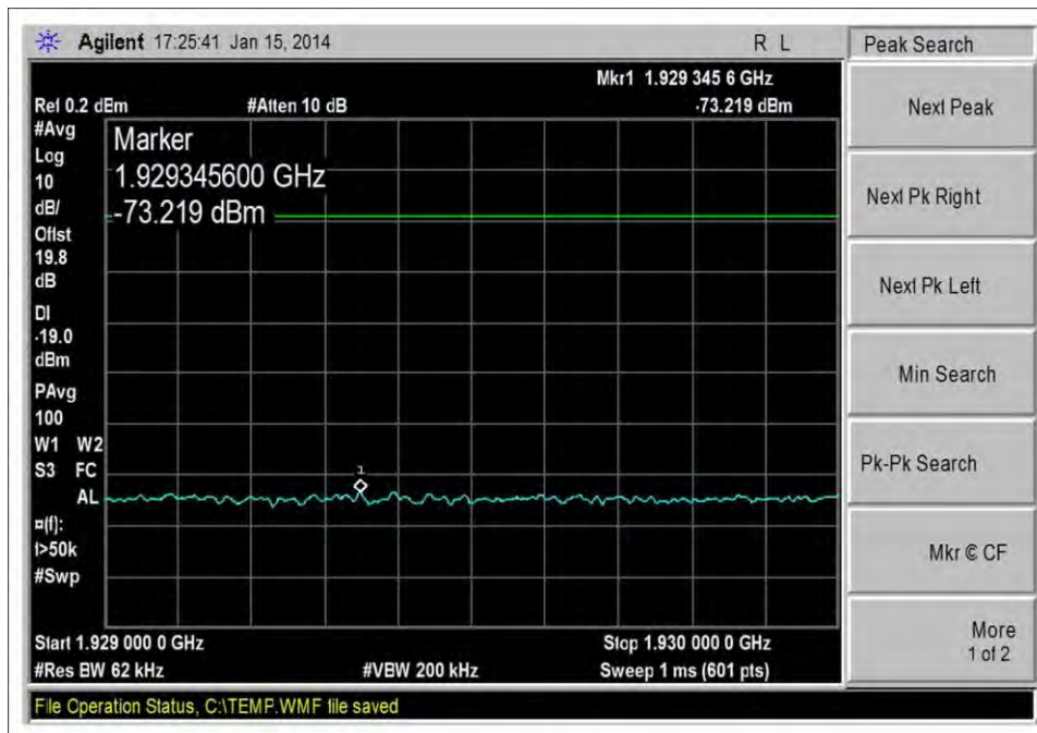
DL_1930-1995MHz_LTE_L_-20dBm
