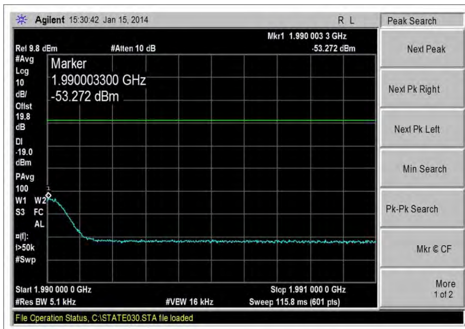
DL_1930-1995MHz_GSM_H_-58dBm
