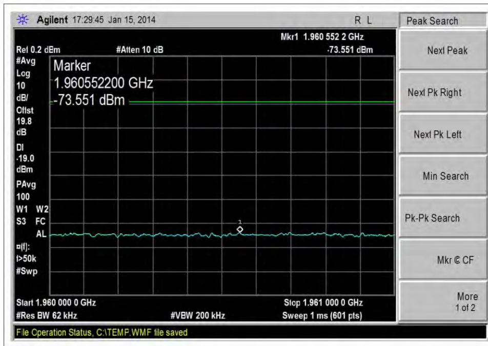
DL_1930-1995MHz_LTE_H_-20dBm
