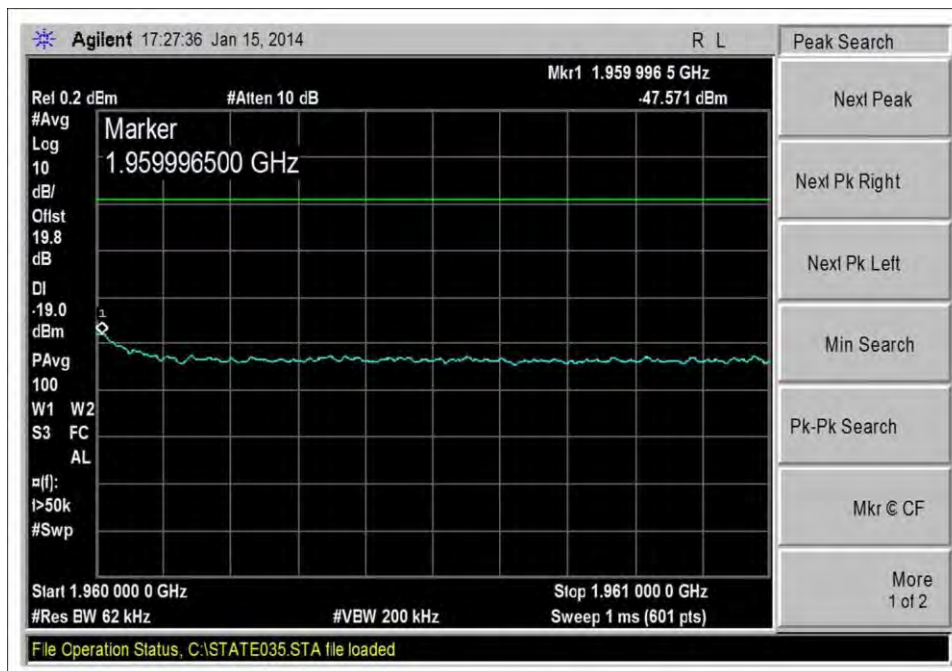
DL_1930-1995MHz_LTE_H_-64dBm
