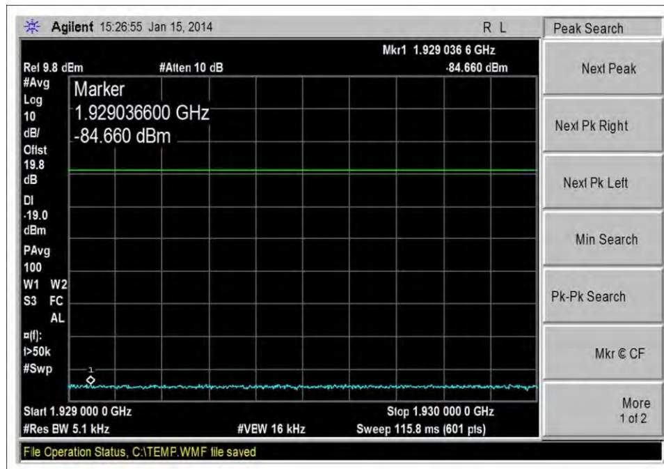
DL_1930-1995MHz_GSM_L_-20dBm
