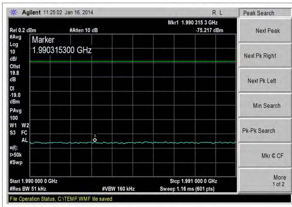
DL_1930-1995MHz_CDMA_H_-20dBm
