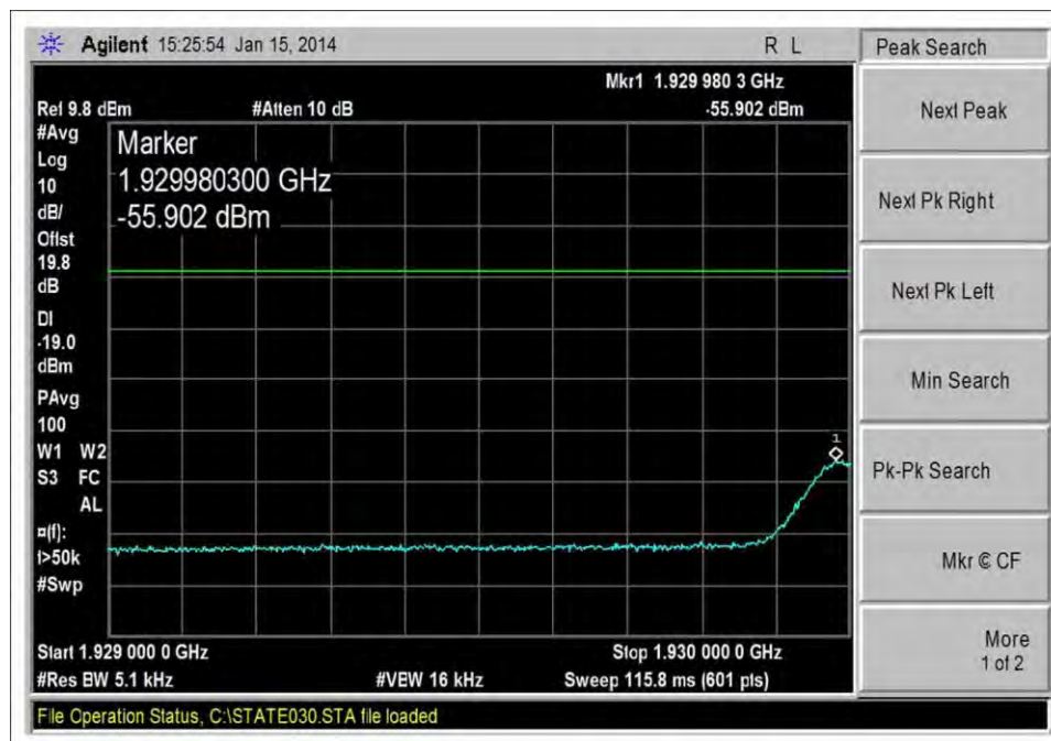
DL_1930-1995MHz_GSM_L_-60dBm
