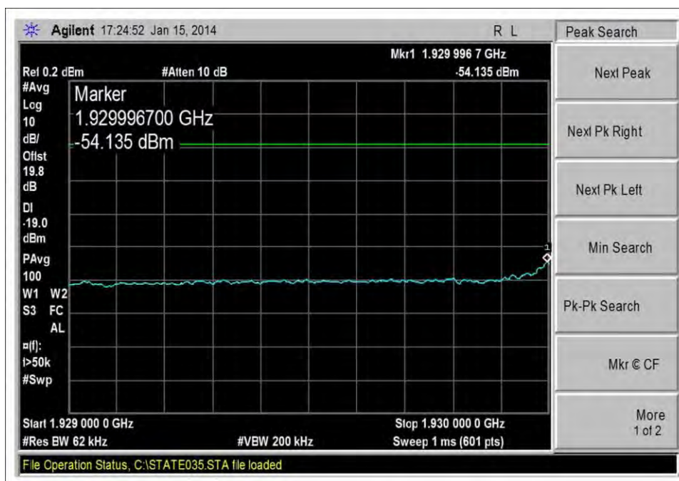
DL_1930-1995MHz_LTE_L_-60dBm
