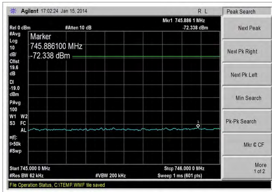
DL_746-757MHz_LTE_L_-20dBm
