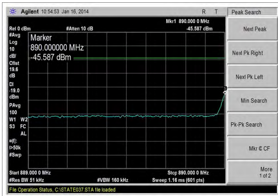
DL_890-891.5MHz_CDMA_L_-62dBm
