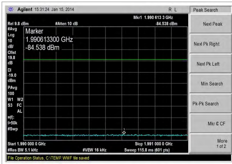
DL_1930-1995MHz_GSM_H_-20dBm
