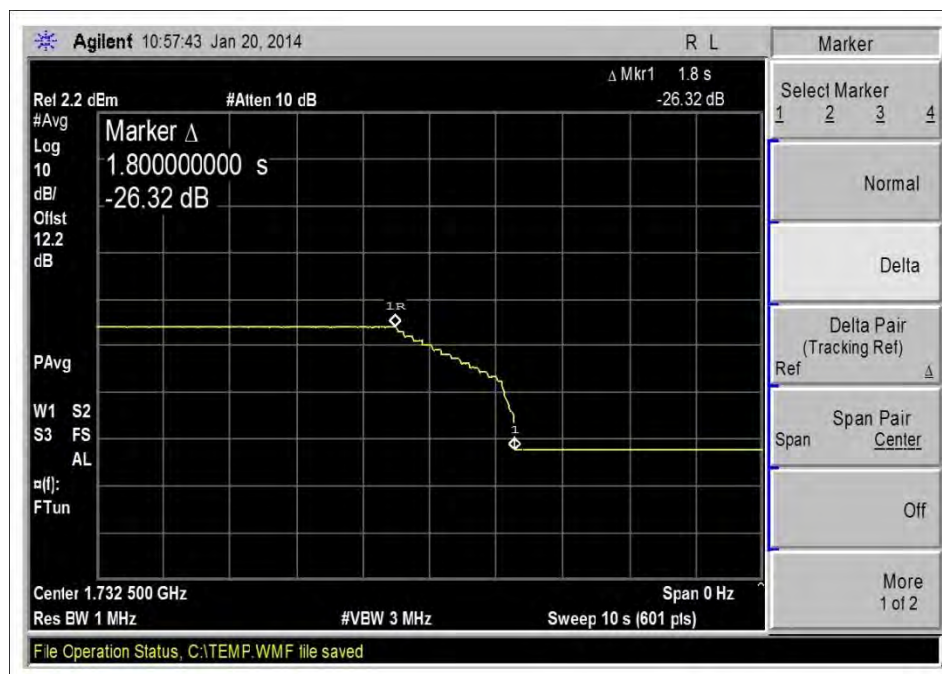
VariableNoiseTiming_UL_1710-1755MHz
