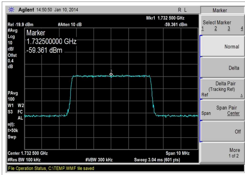
1710-1755MHz UL, LTE-Input
