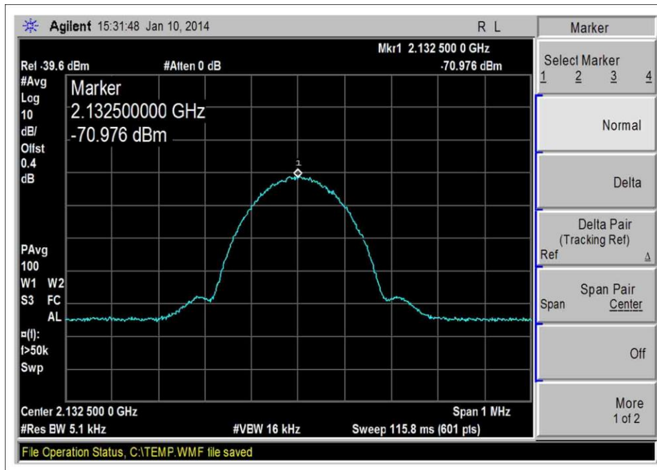
2110-2135MHz DL, GSM-Input
