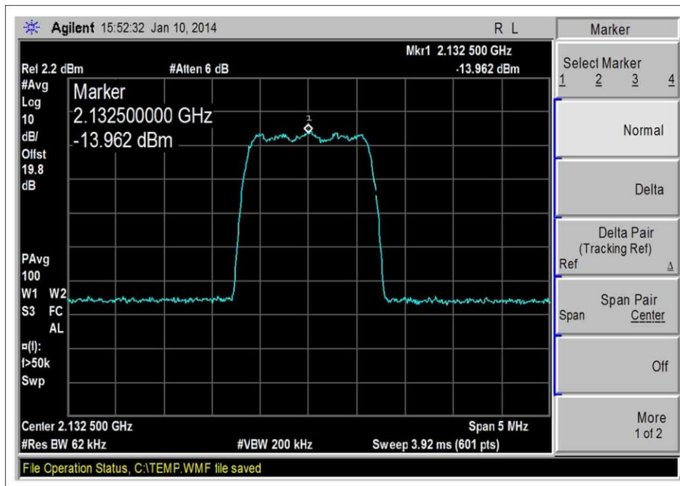
2110-2135MHz DL, CDMA-Output
