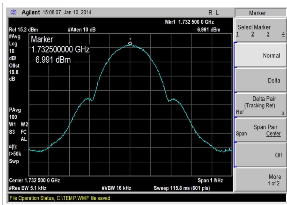
1710-1755MHz UL, GSM-Output
