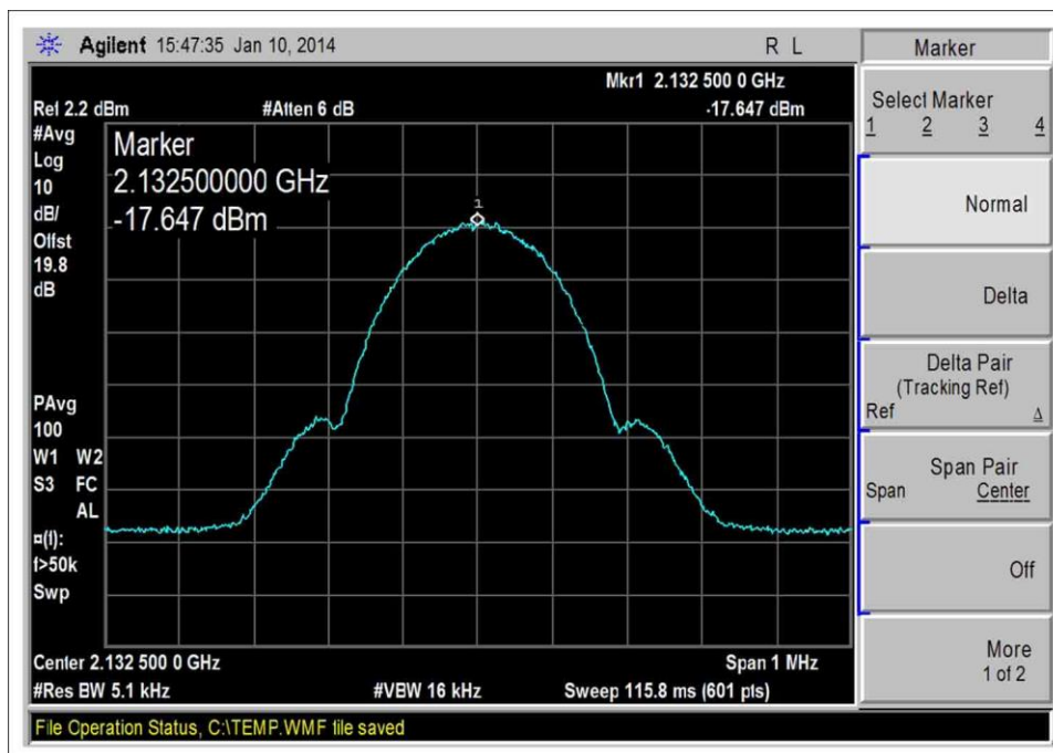
2110-2135MHz DL, GSM-Output
