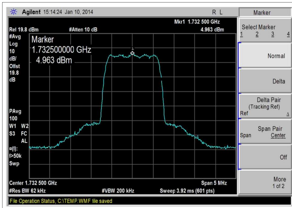
1710-1755MHz UL, CDMA-Output
