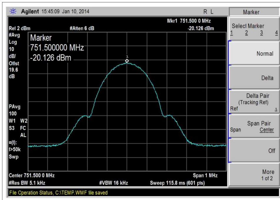
746-757MHz DL, GSM-Output
