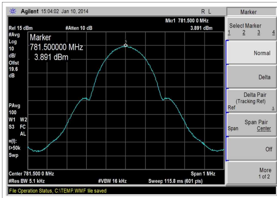
776-787MHz UL, GSM-Output
