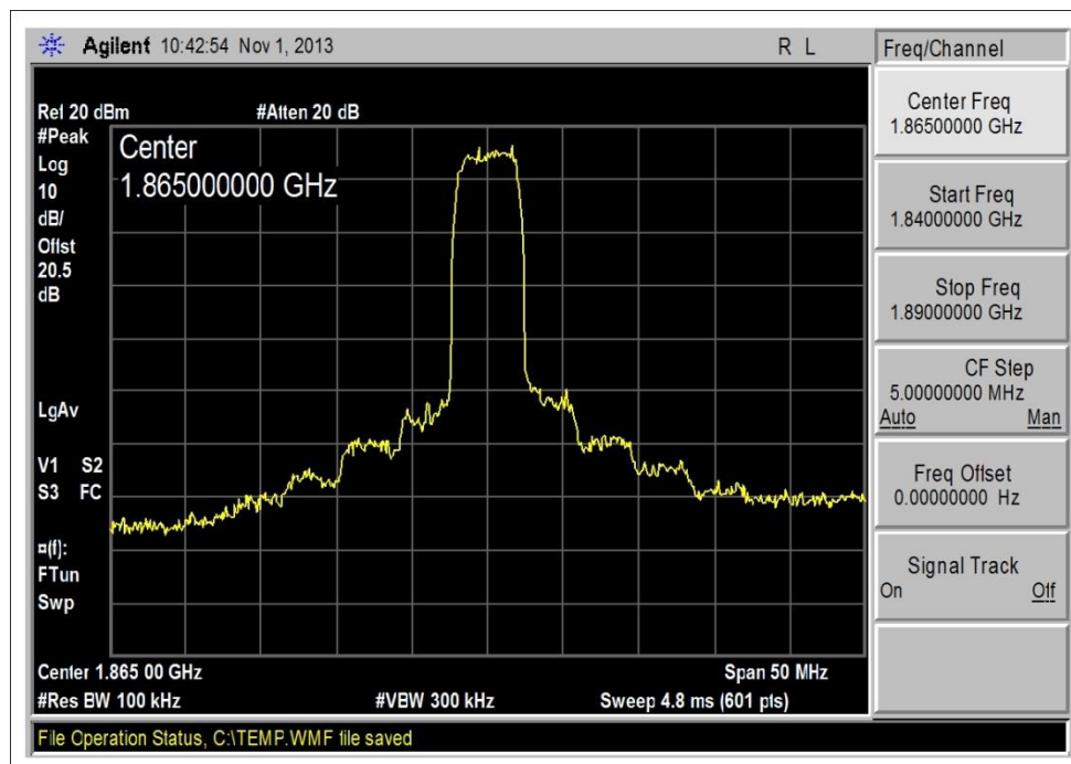
1850-1910MHz UL_WCDMA_Output
