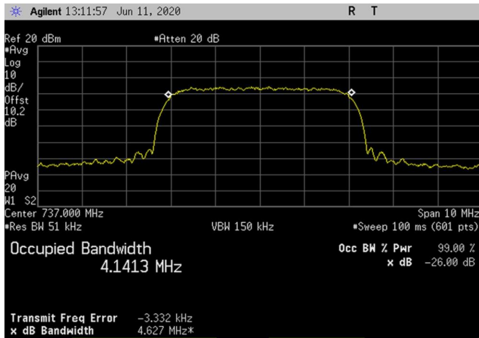
DL_728-746_WCDMA_737MHz
