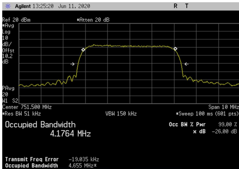
DL_746-757_WCDMA_751.5MHz
