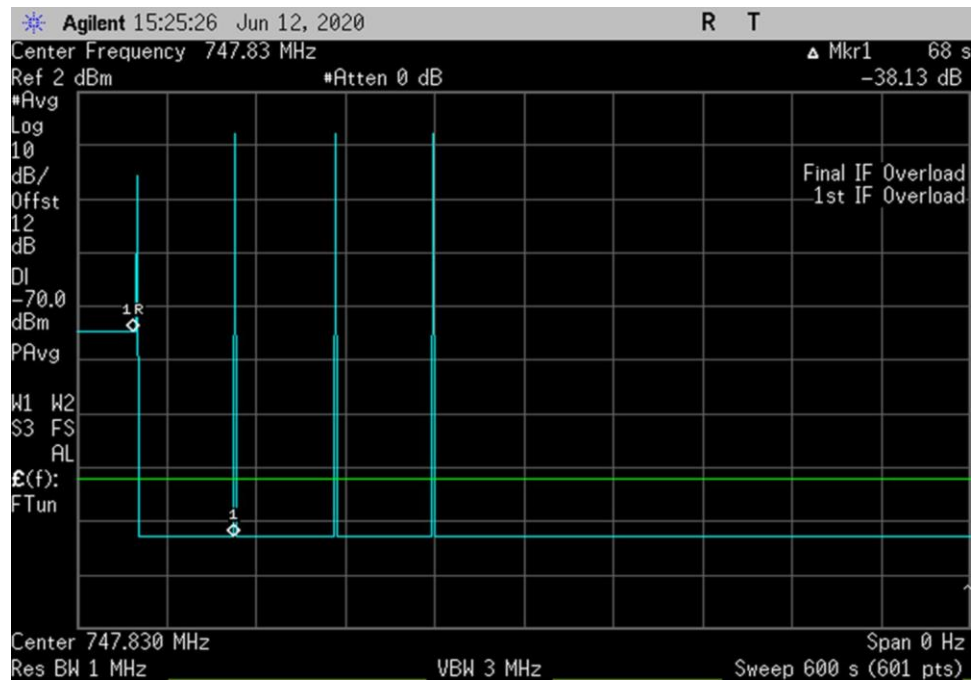
DL_746-757_600sec_747.83MHz
