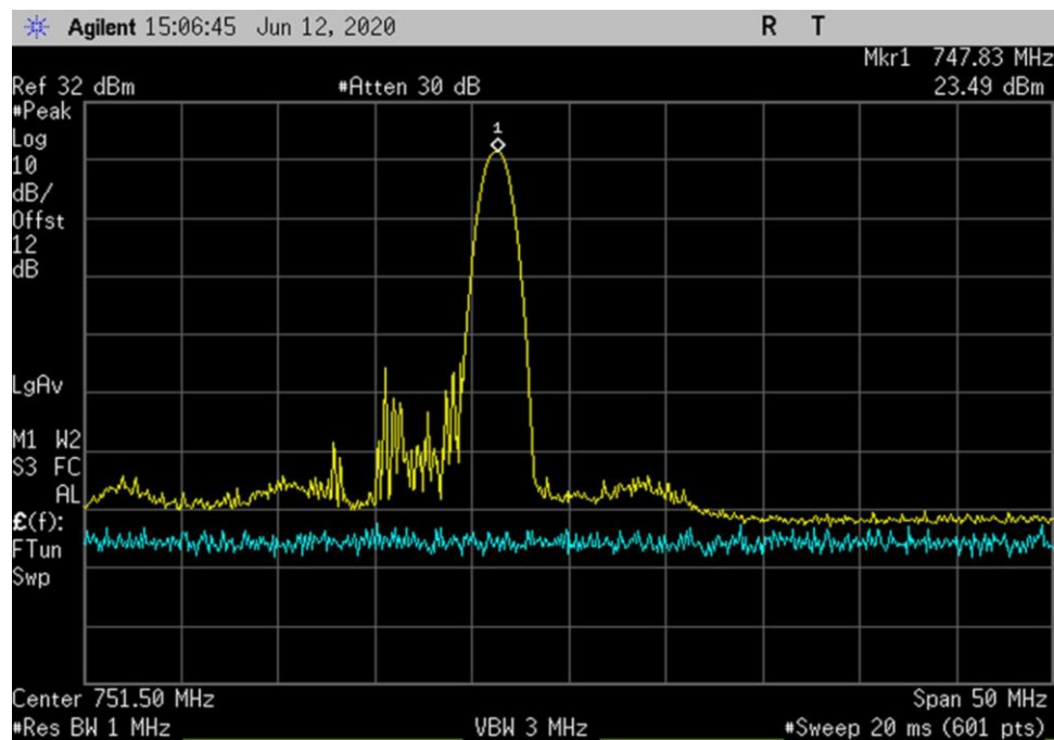
DL_746-757_Pk_751.5MHz
