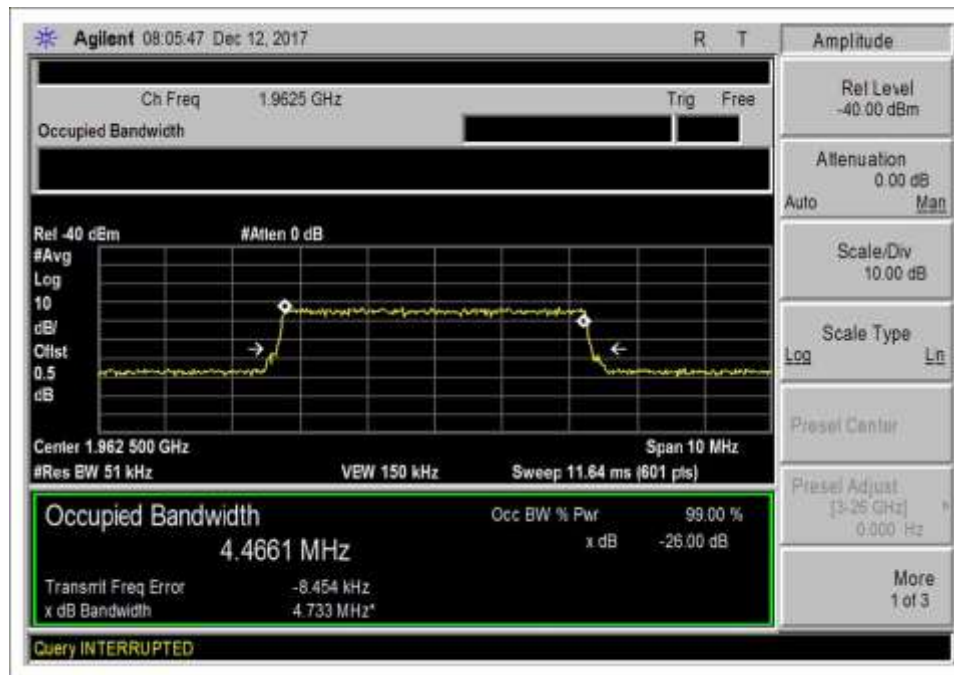
7.10 DL 1930-1995_LTE_IN
