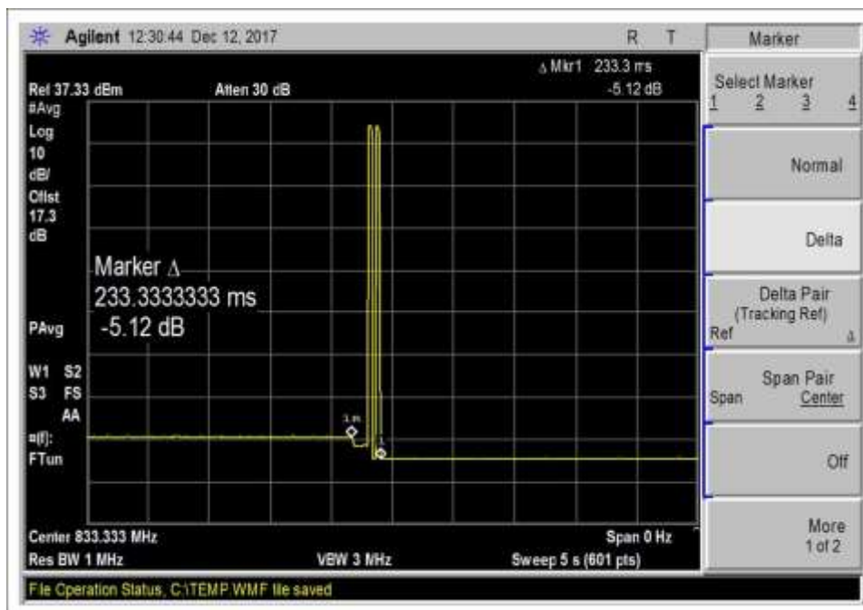
7.11.2 UL 824-849 time
