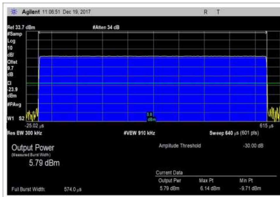
7.2 DL 869-864 pulse_max
