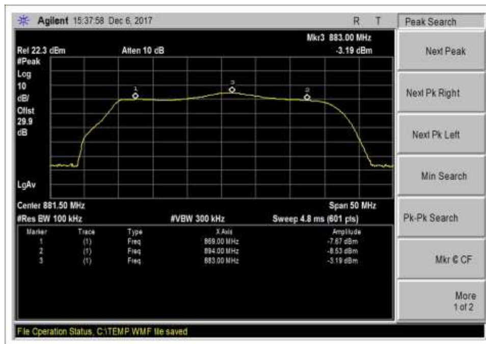
7.1 DL 869-894M
