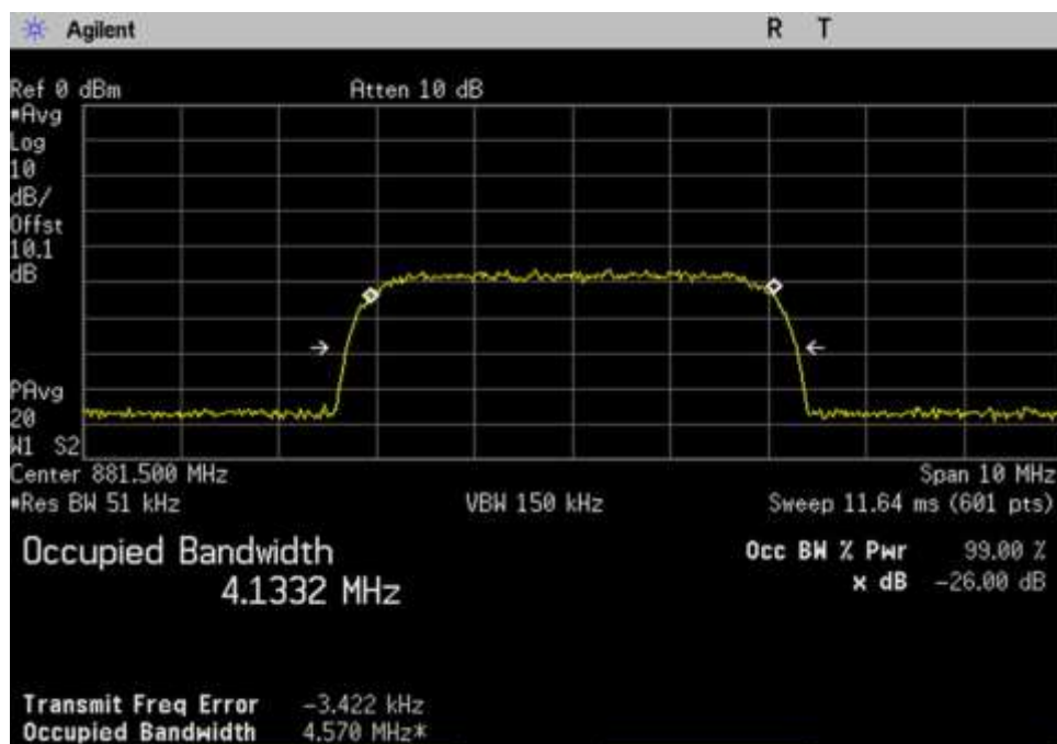
DL_869-894_WCDMA_881.5MHz
