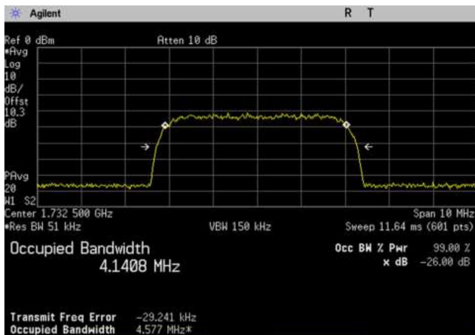
UL_1710-1755_WCDMA_1732.5MHz
