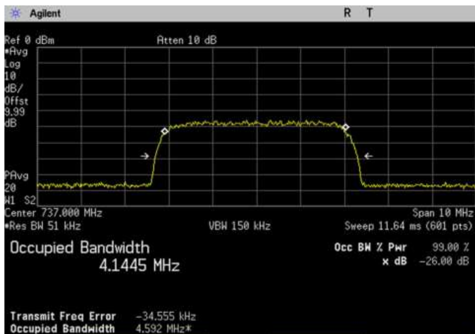
DL_728-746_WCDMA_737MHz
