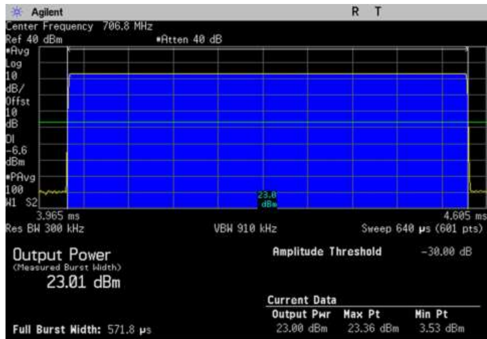
UL_698-716_GSM_706.8MHz
