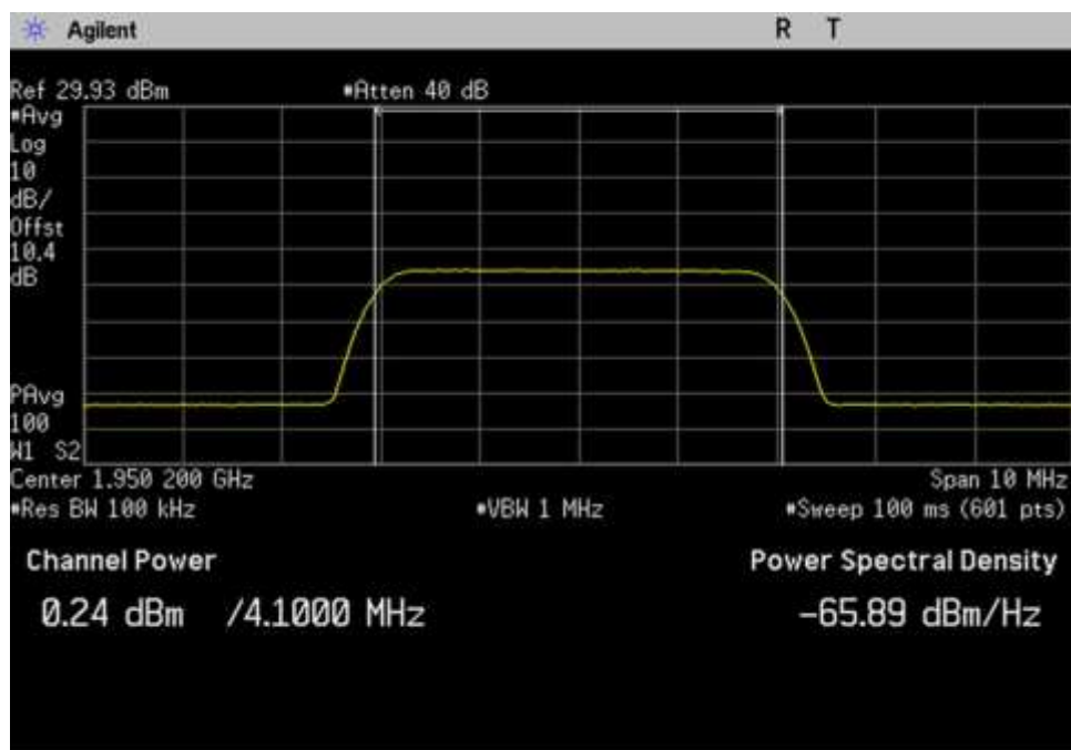
DL_1930-1995_AWGN_ 1950.2MHz
