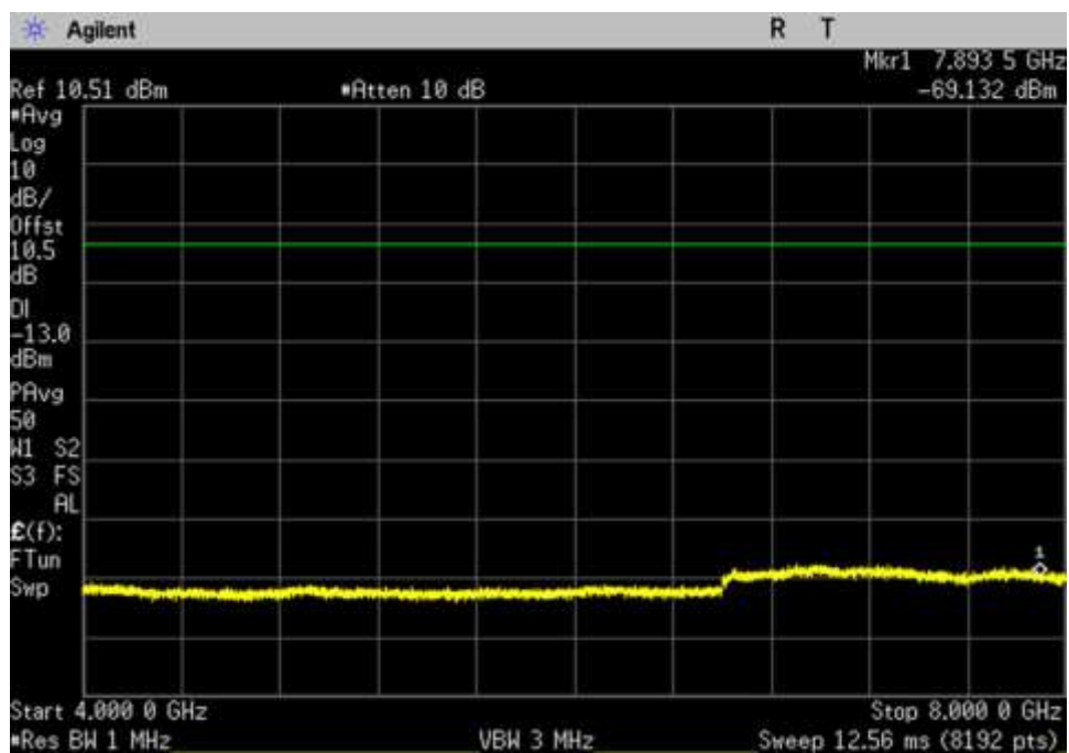
DL_2110-2155_ 4000- 8000MHz
