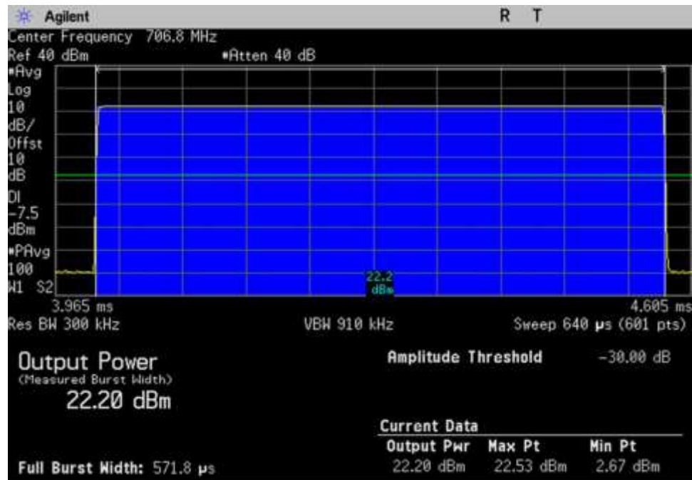
UL_698-716_GSM_Max_706.8MHz
