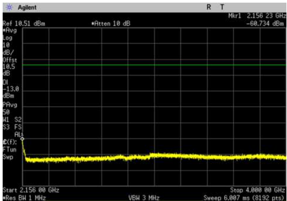
DL_2110-2155_ 2156- 4000MHz
