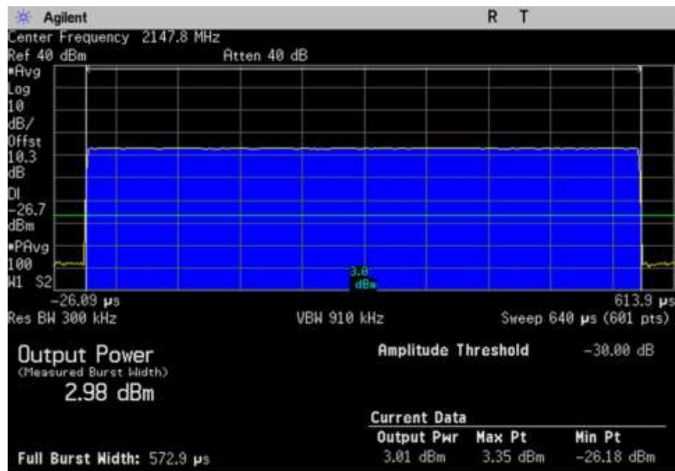
DL_2110-2155_GSM_ 2147.8MHz
