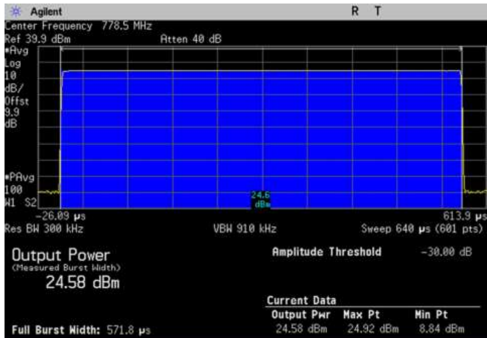
UL_776-787_GSM_Max_ 778.5MHz
