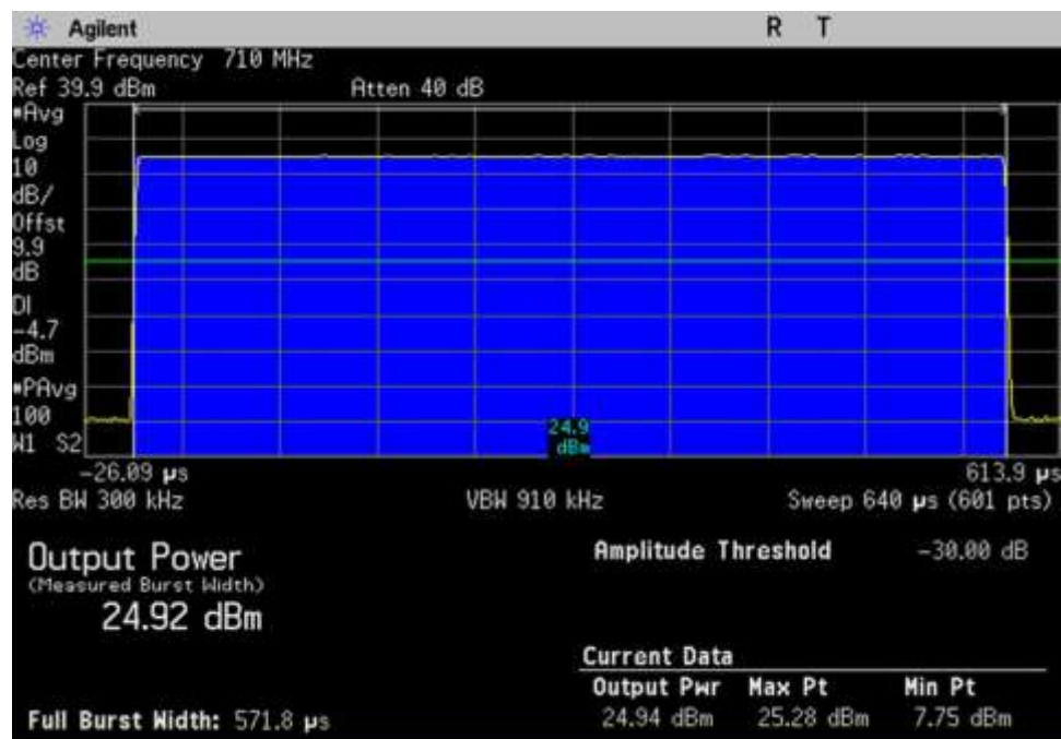
UL_698-716_GSM_710MHz
