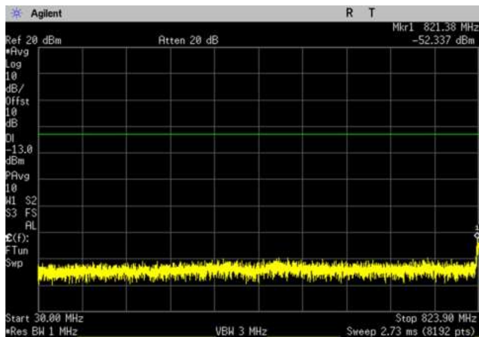
UL_824-849_ 30- 823.9MHz
