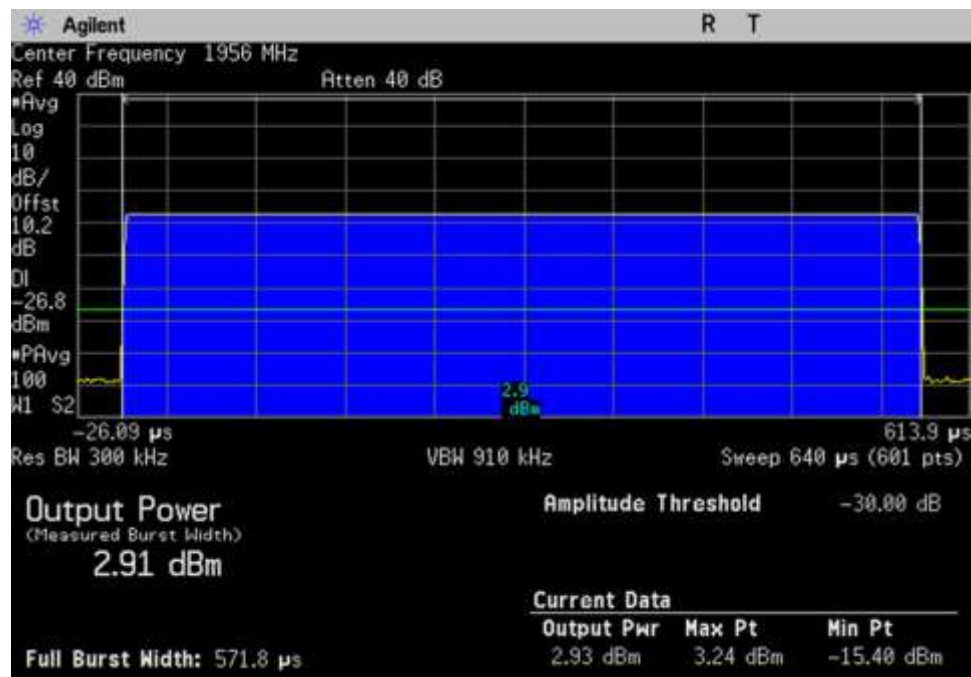
DL_1930-1995_GSM_1956MHz
