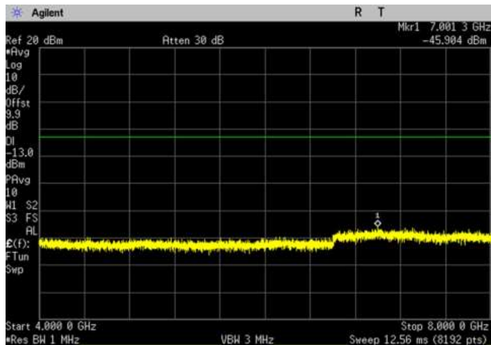
UL_776-787_ 4000- 8000MHz
