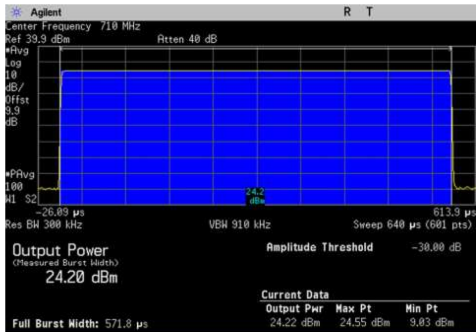
UL_698-716_GSM_Max_710MHz
