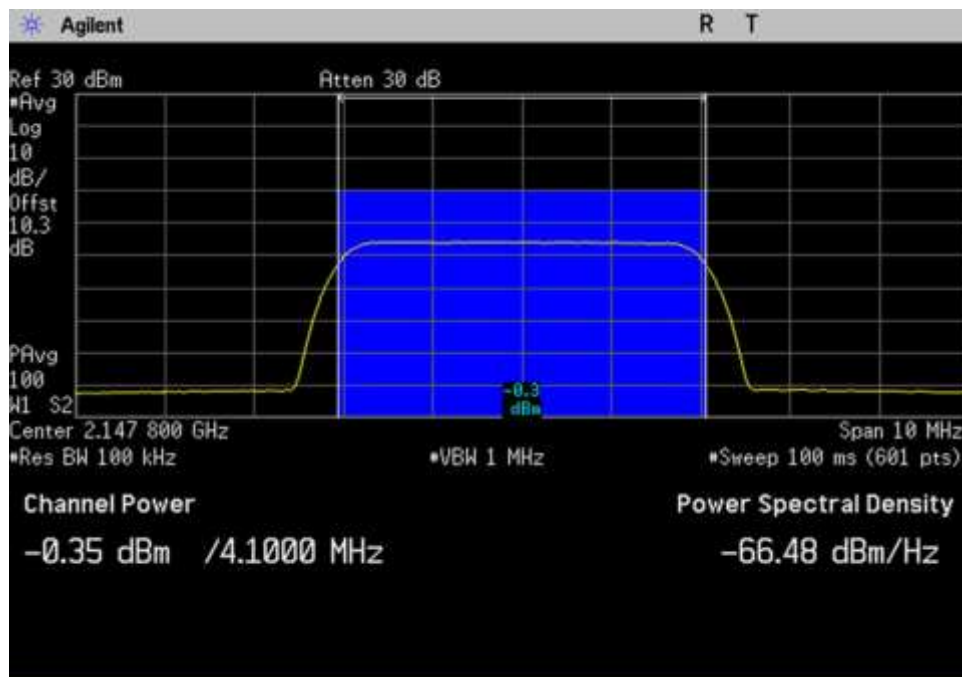
DL_2110-2155_AWGN_2147.8MHz
