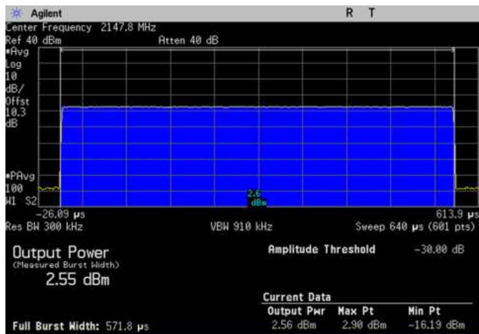
DL_2110-2155_GSM_Max_ 2147.8MHz
