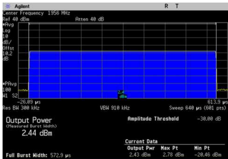
DL_1930-1995_GSM_Max_1956MHz
