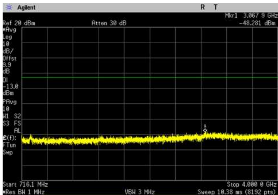
UL_698-716_716.1- 4000MHz
