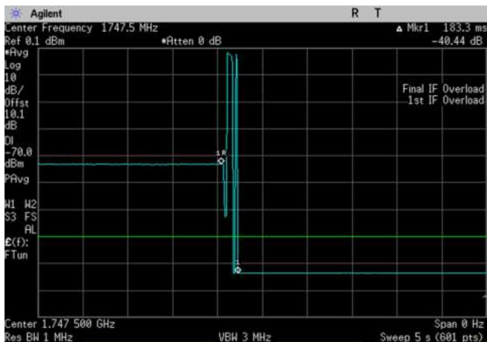
UL_1710-1755_ 1747.5MHz
