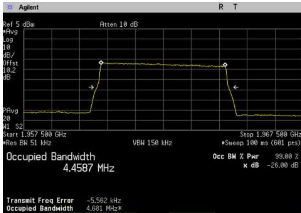
DL_1930-1995_LTE_ 1962.5MHz
