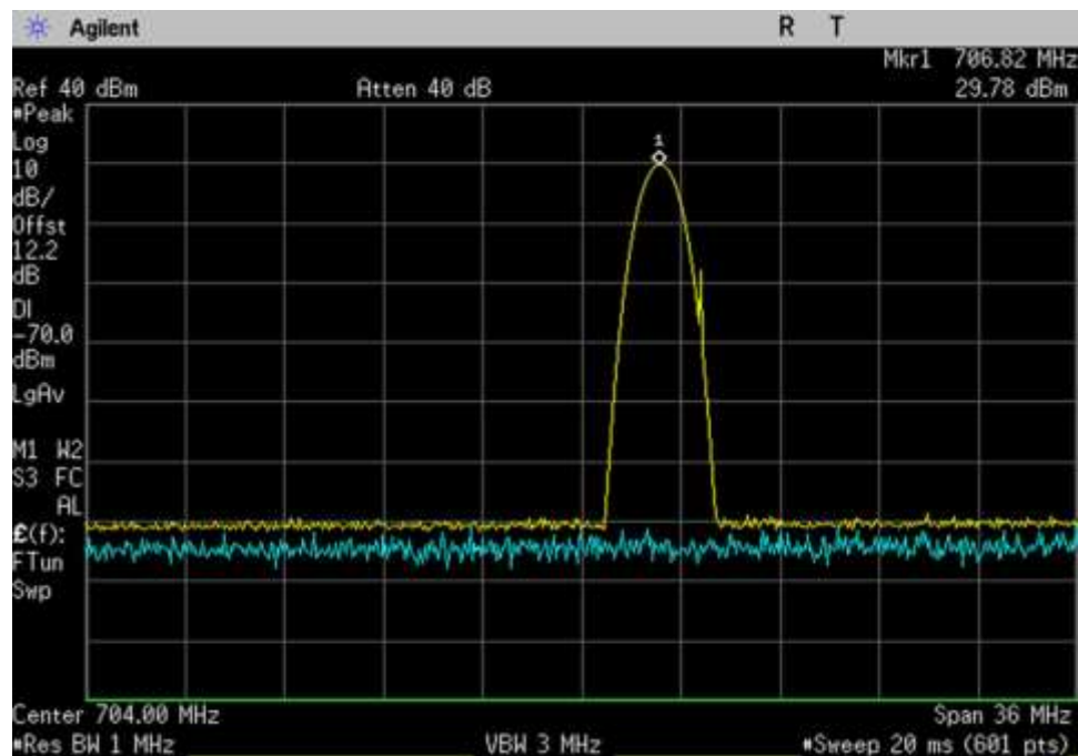
UL_698-716_Pk_ 704MHz
