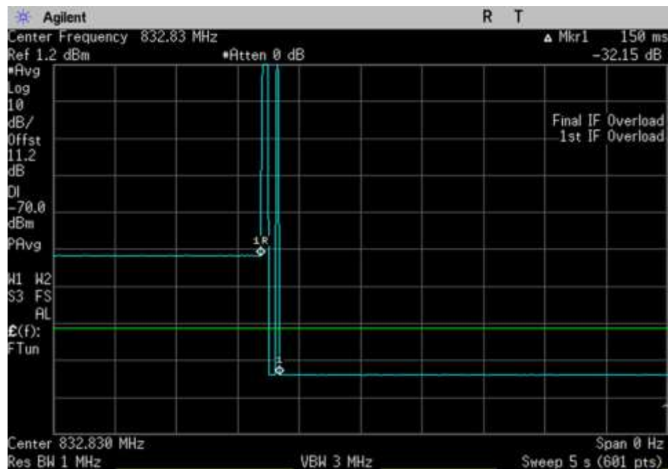
UL_824-849_ 832.83MHz
