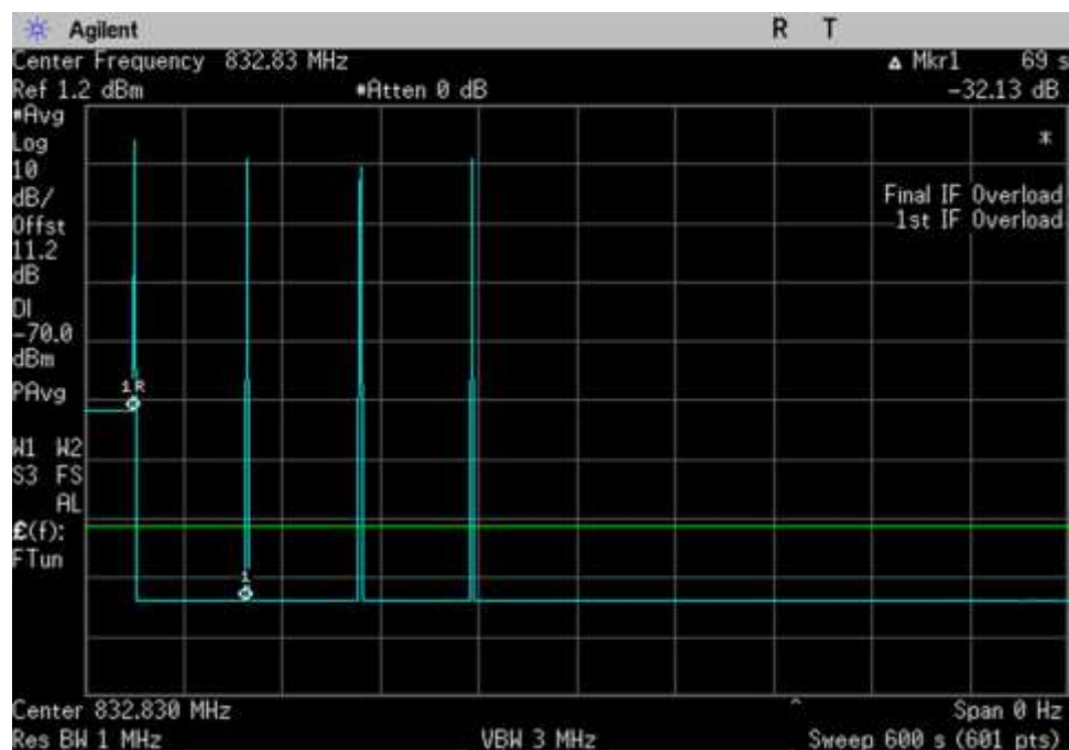
UL_824-849_600sec_ 832.83MHz
