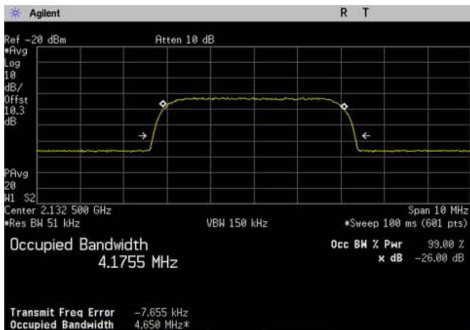
DL_2110-2155_WCDMA_2132.5MHz
