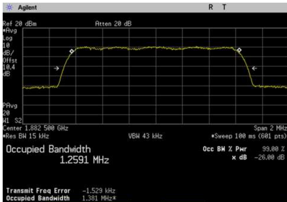
UL_1850-1915_CDMA_1882.5MHz
