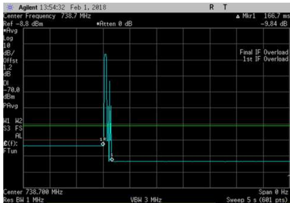
DL_728-746_ 738.7MHz
