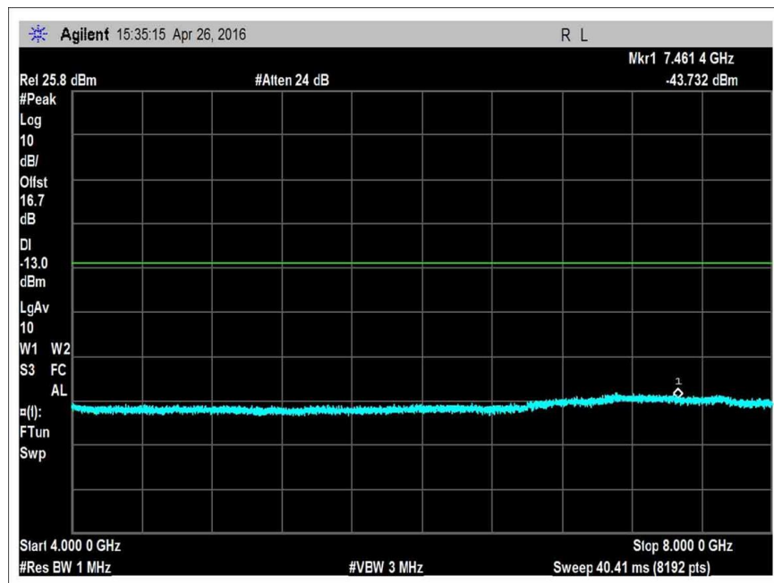
2.1051_DL_869-894R2
