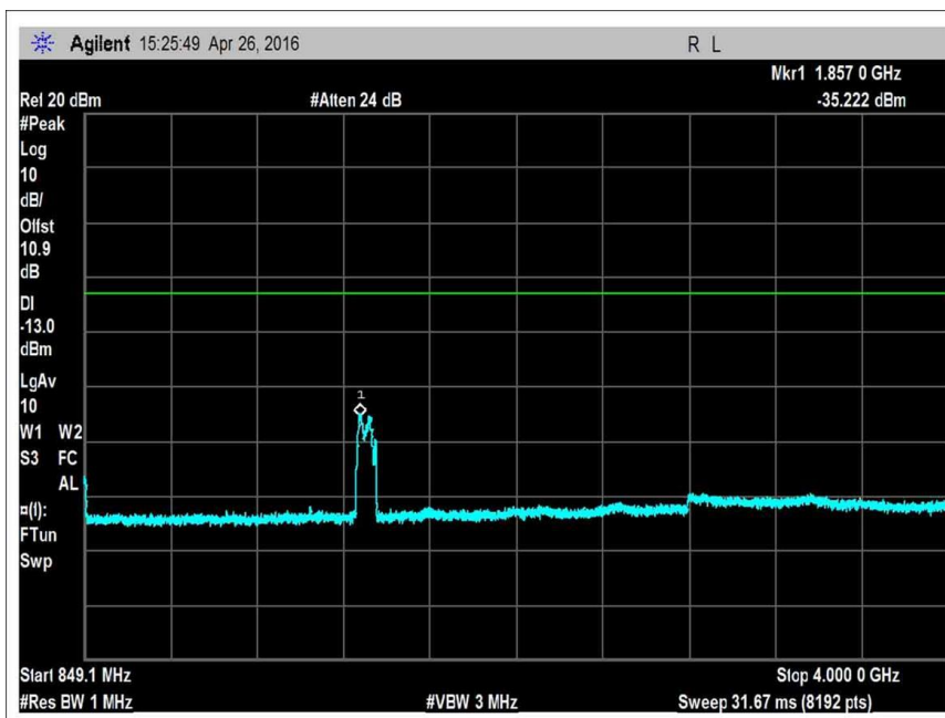
2.1051_UL_824-849R1
