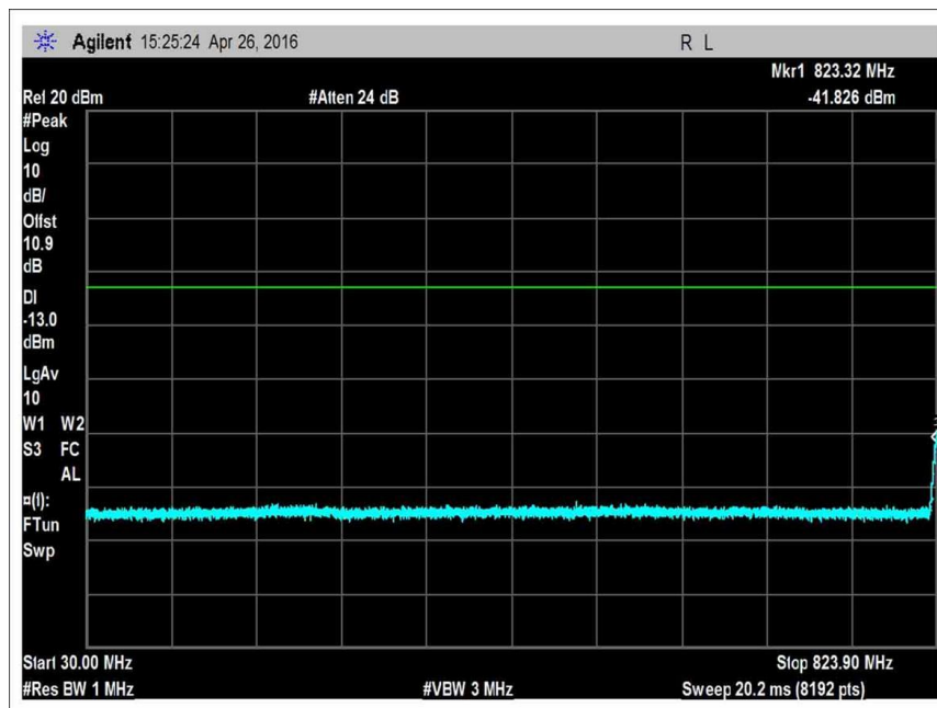
2.1051_UL_824-849L
