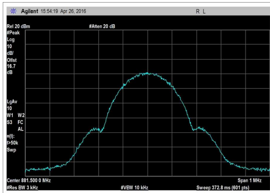
OBW_DL_869-894MHz_GSM
