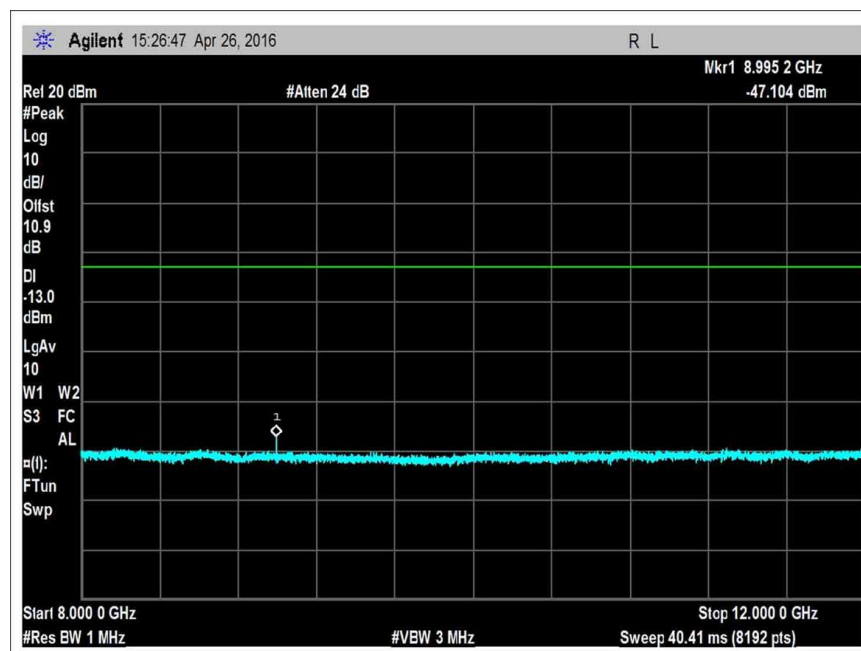
2.1051_UL_824-849R3
