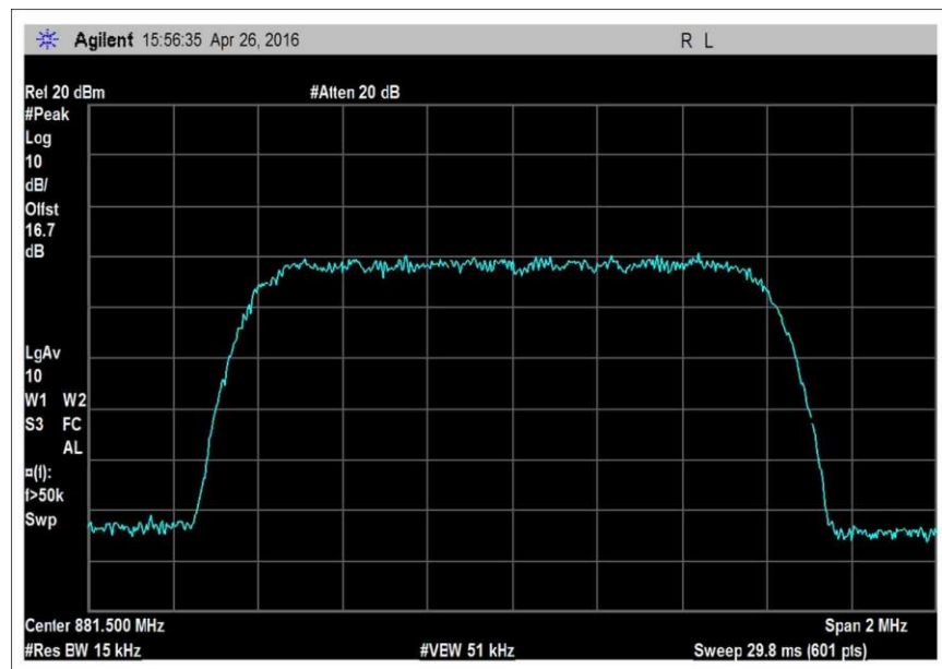
OBW_DL_869-894MHz_CDMA
