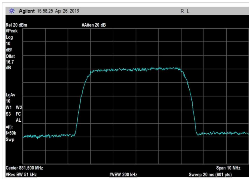
OBW_DL_869-894MHz_WCDMA
