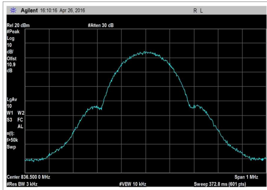
OBW_UL_824-849MHz_GSM
