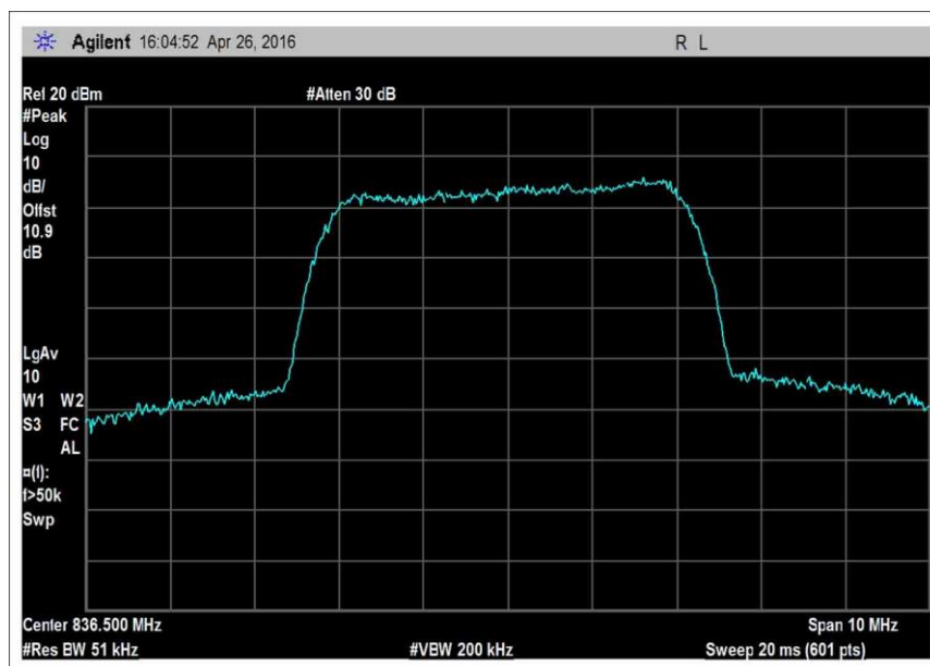
OBW_UL_824-849MHz_WCDMA
