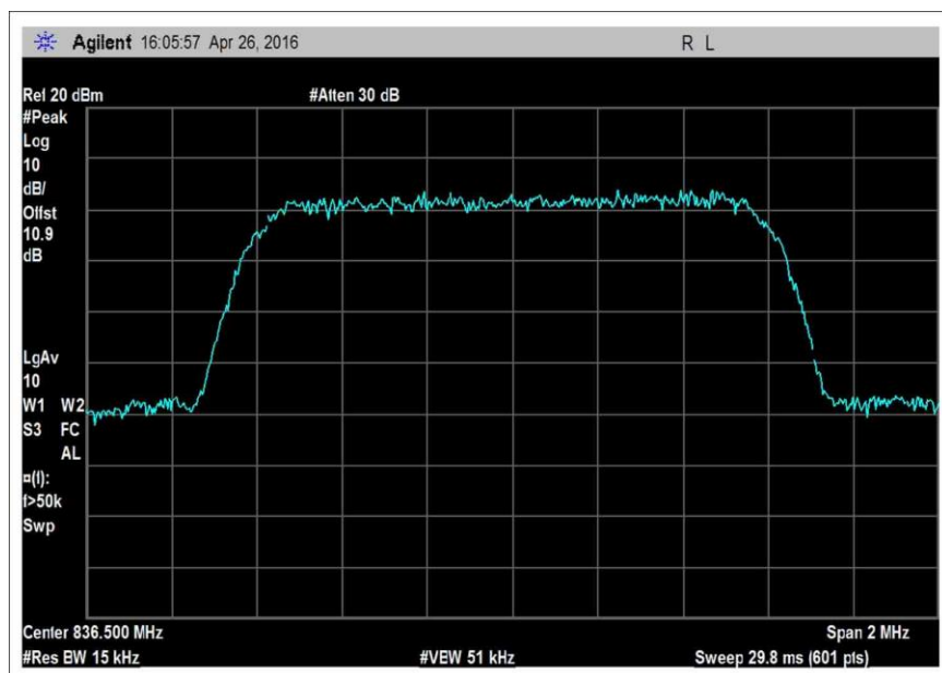
OBW_UL_824-849MHz_CDMA
