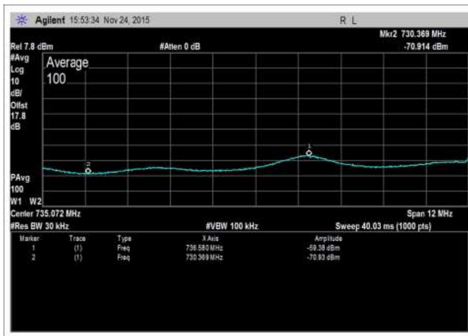
DL-728-746-AWGNR+4
