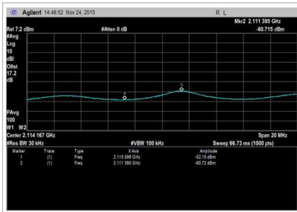
DL-2110-2155-AWG NR+5
