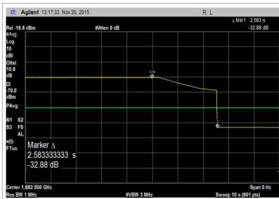
7.7_VarNoise_UL_1850-1915MHz
