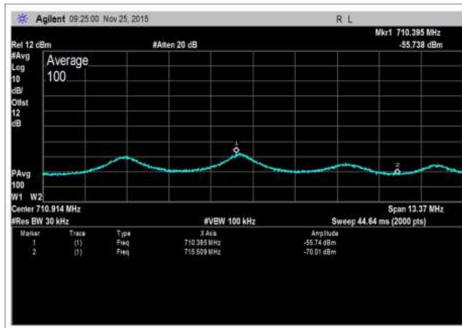
UL-698-716-AWGNL+1
