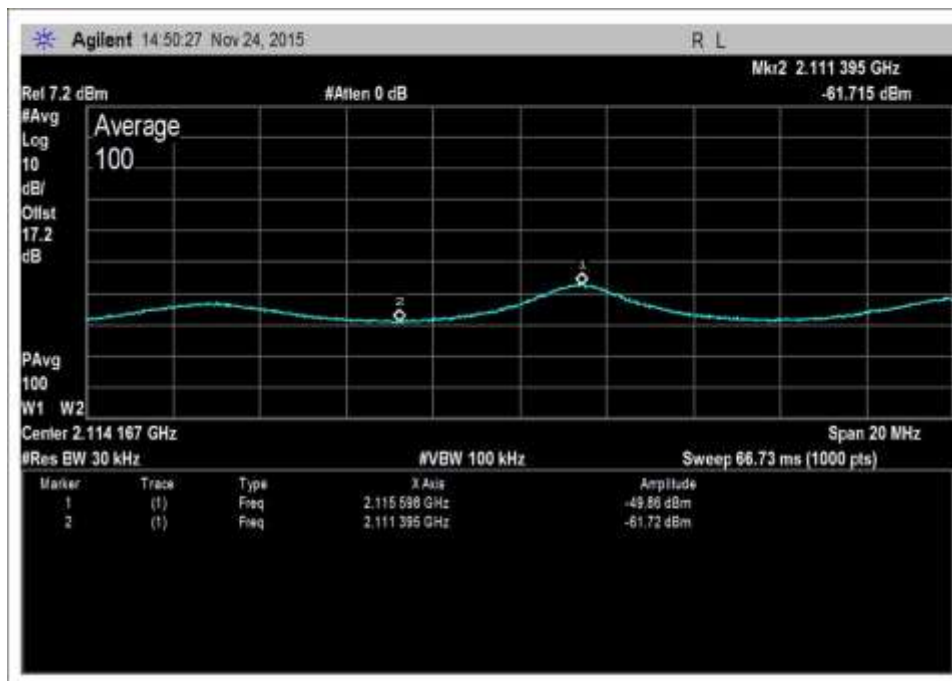
DL-2110-2155-AWG NR+3
