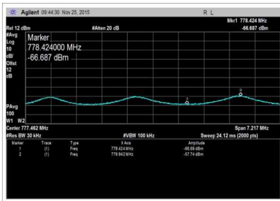
UL-776-787-AWGNL+5
