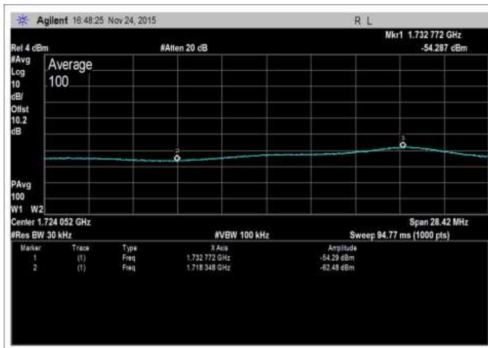
UL-1710-1755-AWGNR+2
