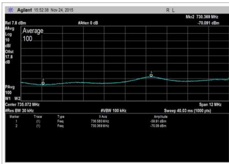
DL-728-746-AWGNR+5
