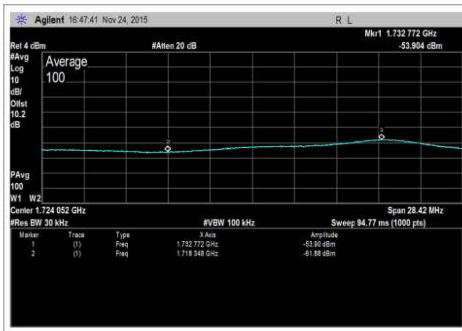
UL-1710-1755-AWGNR+3
