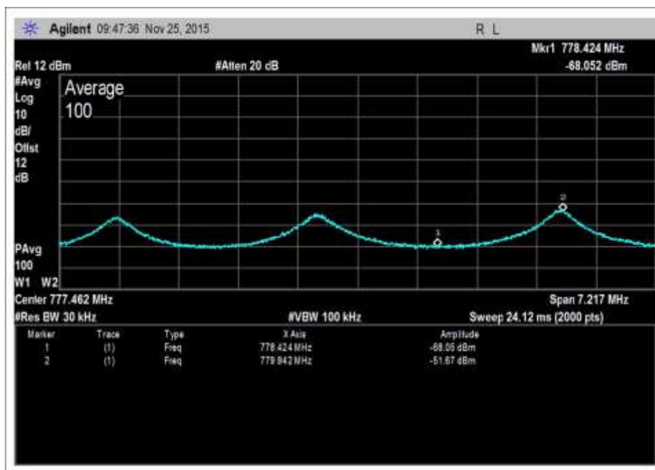
UL-776-787-AWGNL+1
