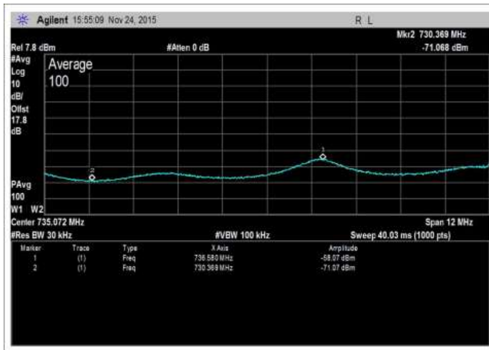
DL-728-746-AWGNR+2
