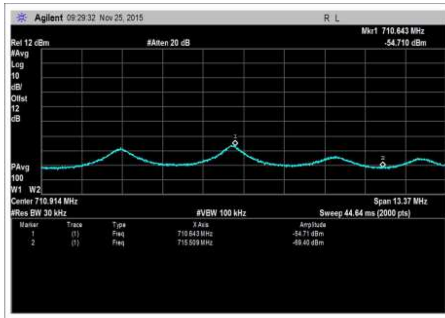
UL-698-716-AWGNL+0
