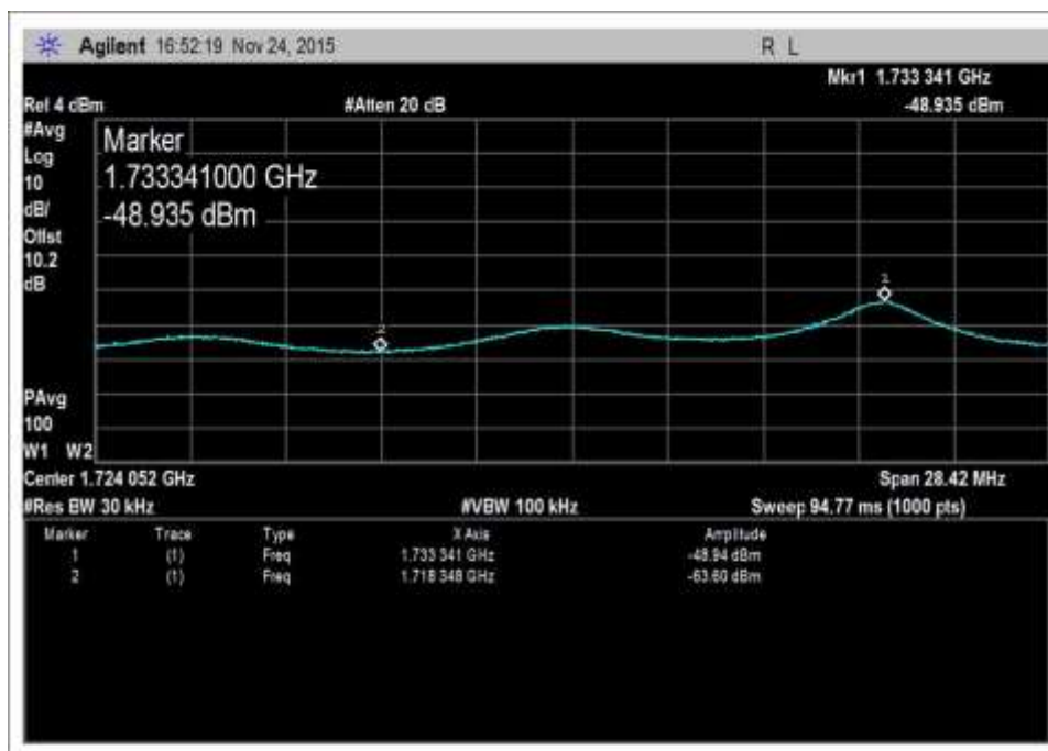
UL-1710-1755-AWGNR+0
