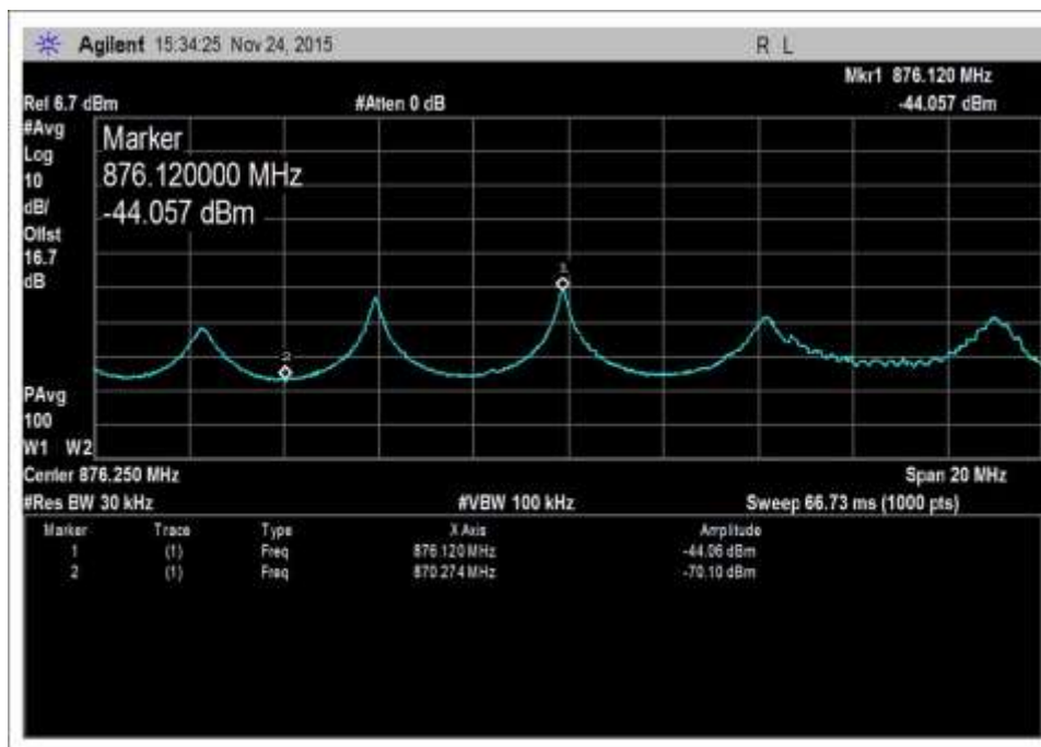
DL-869-894-AWG NR-2
