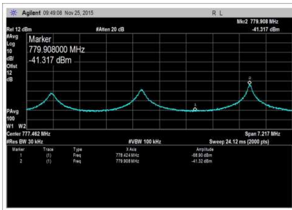
UL-776-787-AWGNL-2
