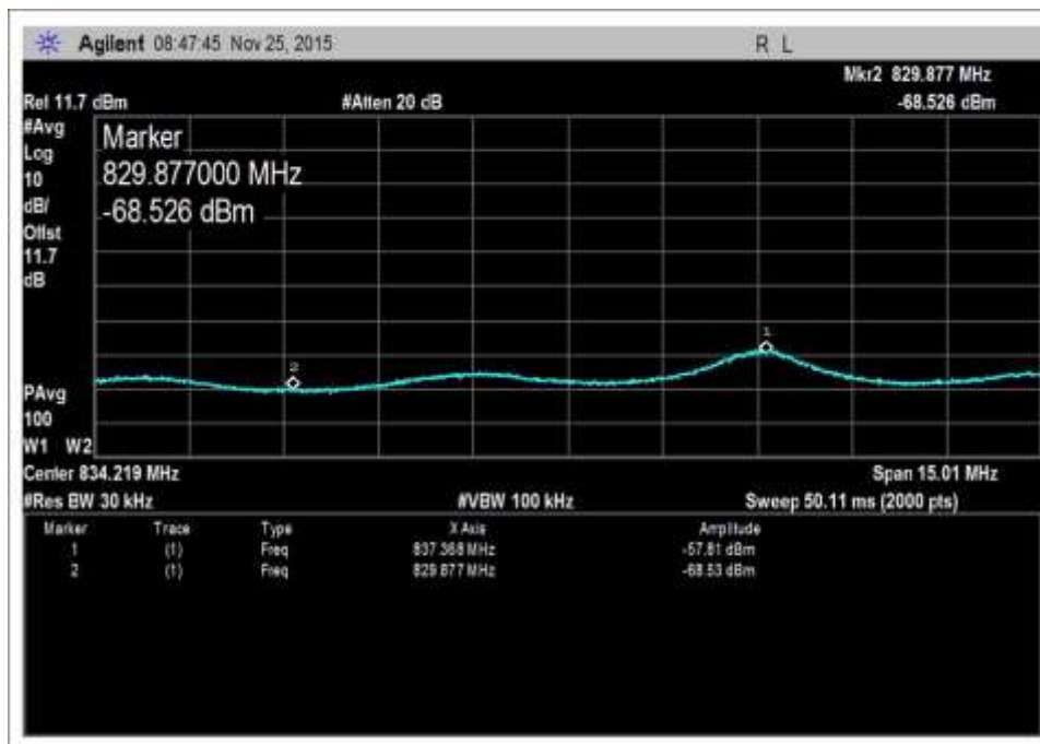
UL-824-849-AWGNR+3
