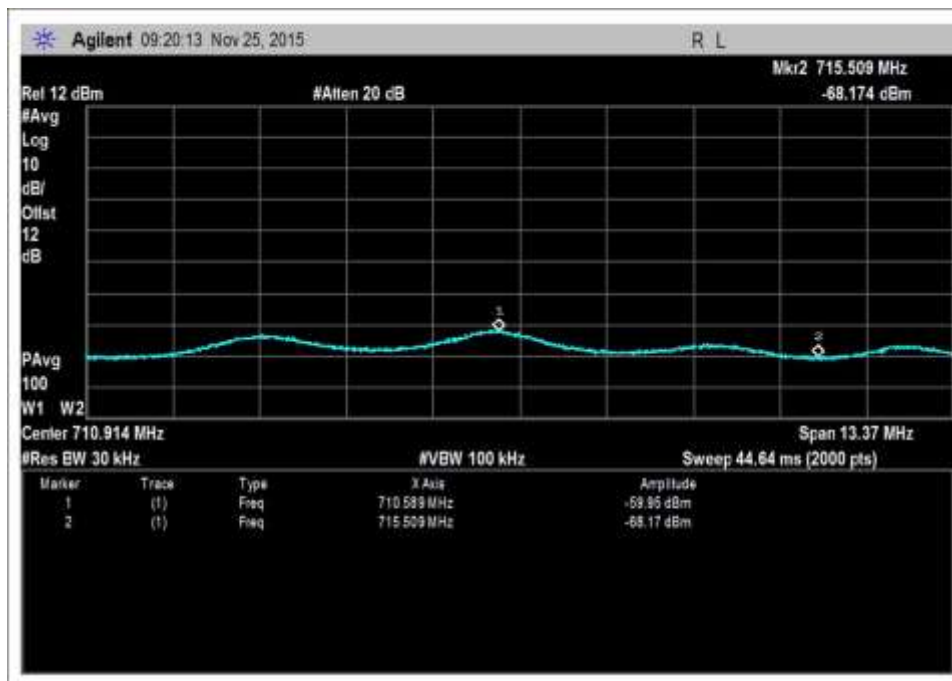
UL-698-716-AWGNL+5
