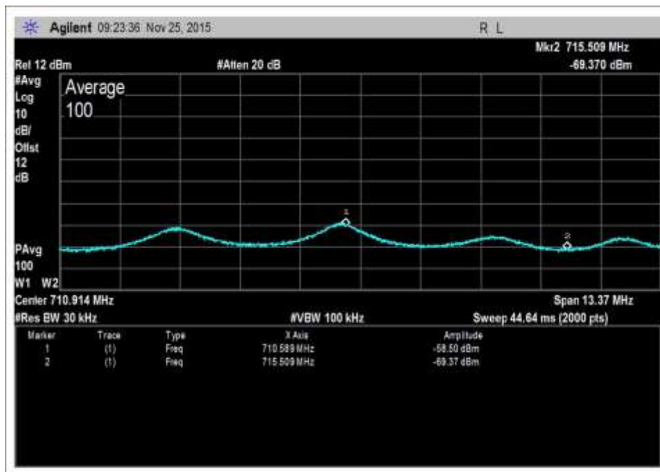
UL-698-716-AWGNL+2
