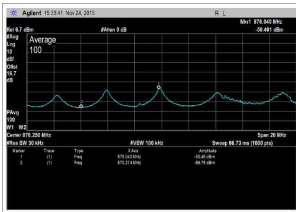
DL-869-894-AWGNR-1
