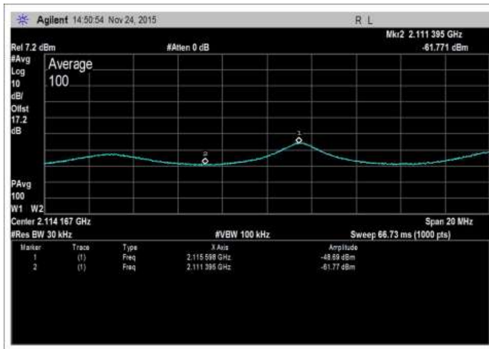
DL-2110-2155-AWG NR+2
