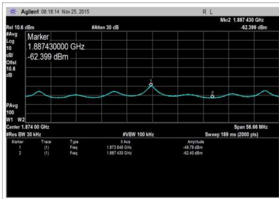
UL-1850-1915-AWGNR+3
