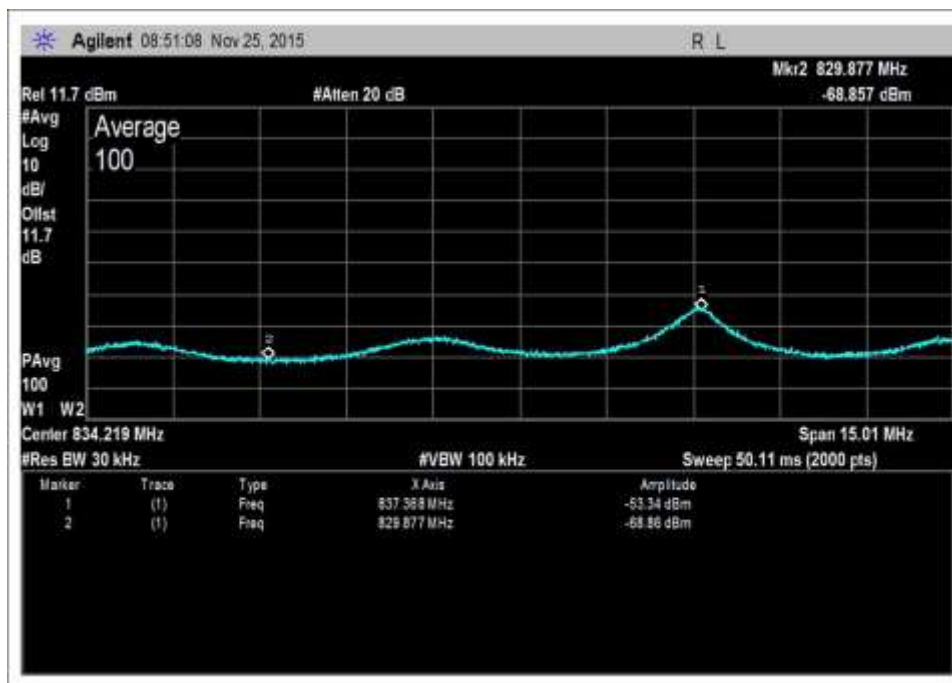
UL-824-849-AWGNR-1
