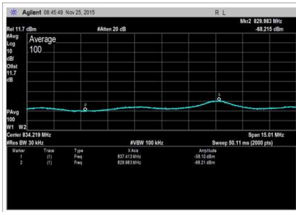
UL-824-849-AWGNR+5
