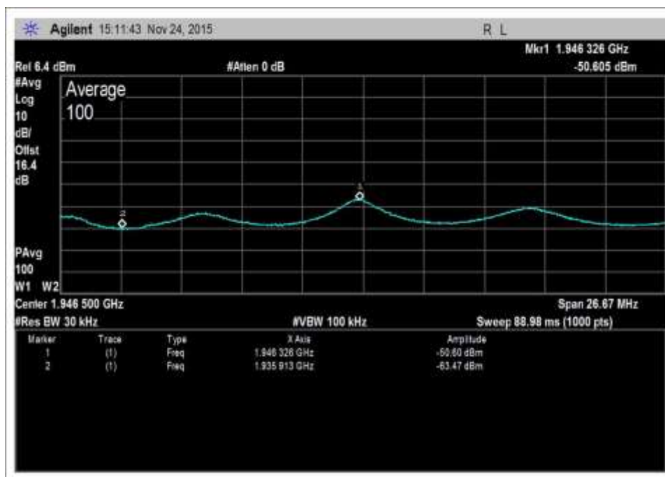
DL-1930-1995-AWG NR+1
