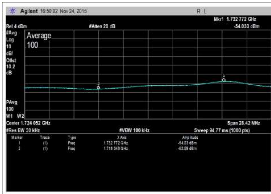
UL-1710-1755-AWGNR+1
