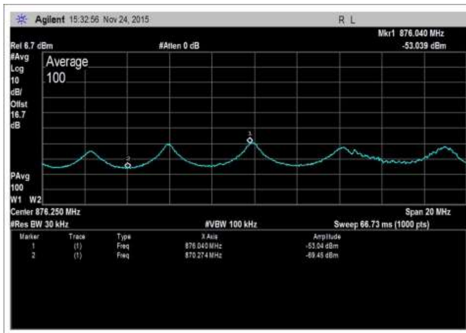
DL-869-894-AWGNR+0
