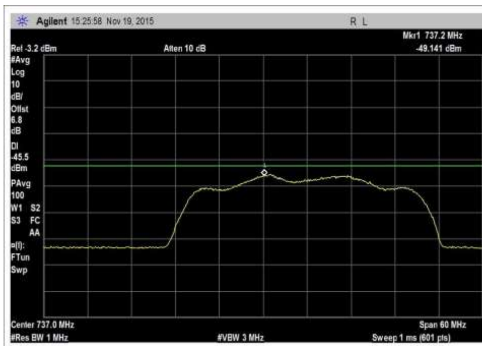
7.7_Noise_DL_728-746MHz-Zoom
