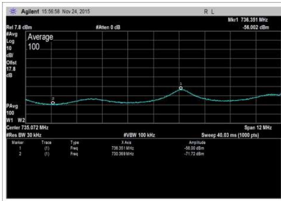
DL-728-746-AWGNR+0
