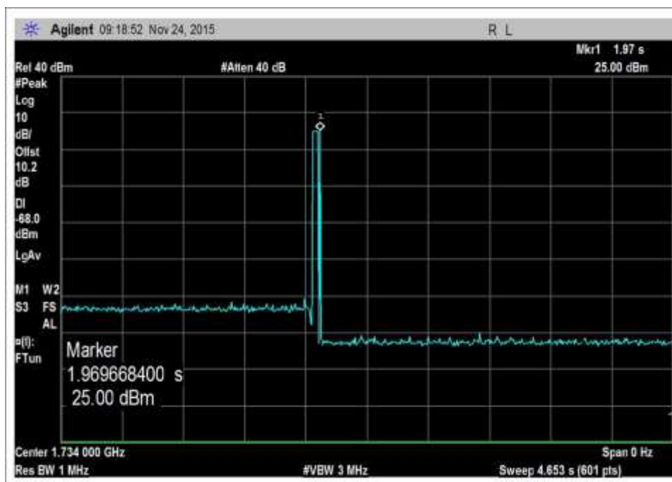
7.11_osc_UL-1710-1755MHz-Pk
