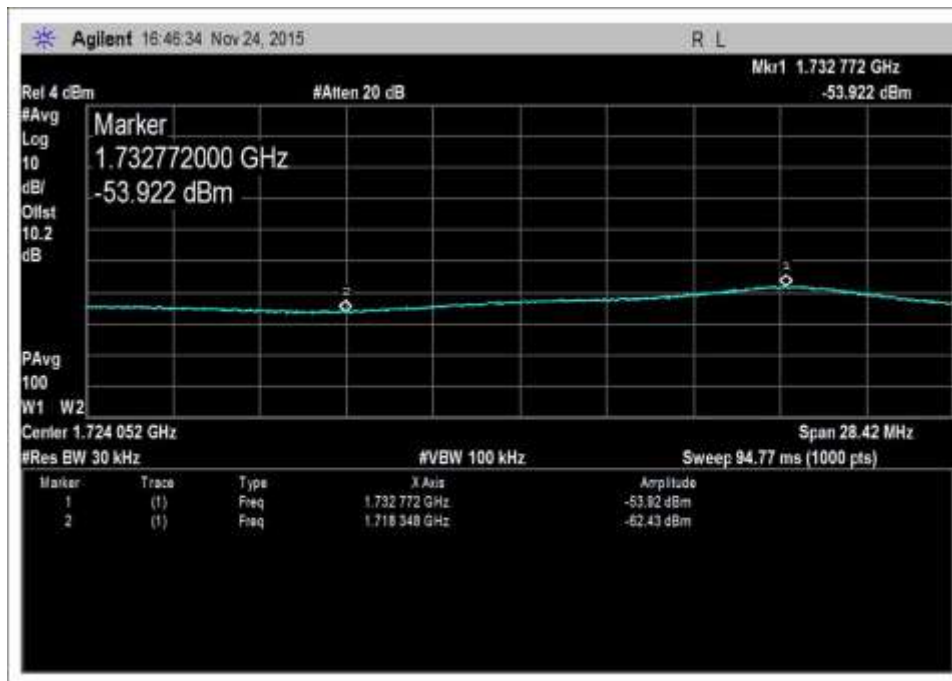
UL-1710-1755-AWG NR+5
