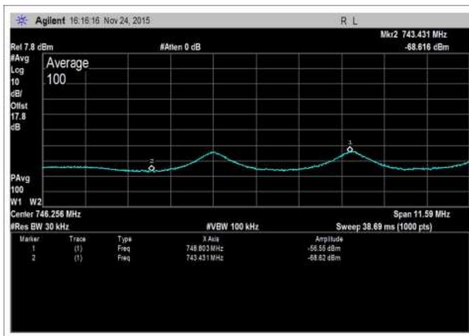
DL-746-757-AWGNR+3
