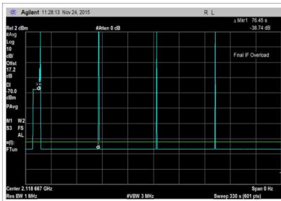
7.11_osc_DL-2110-2155MHz-330sec
