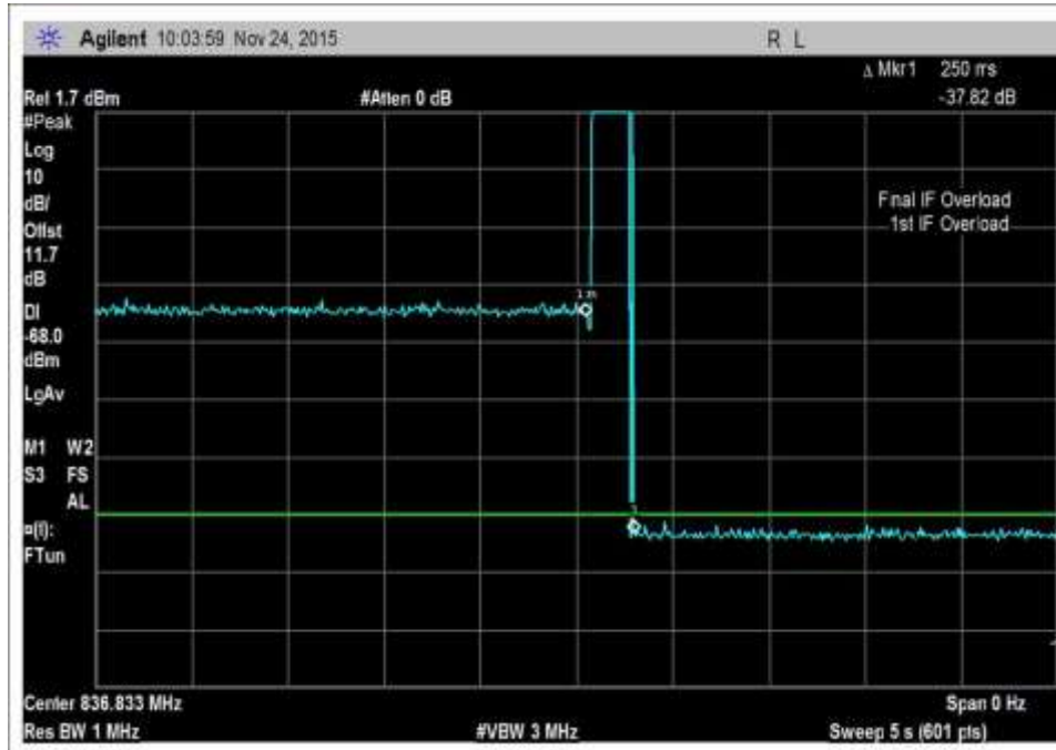
7.11_osc_UL-824-849MHz
