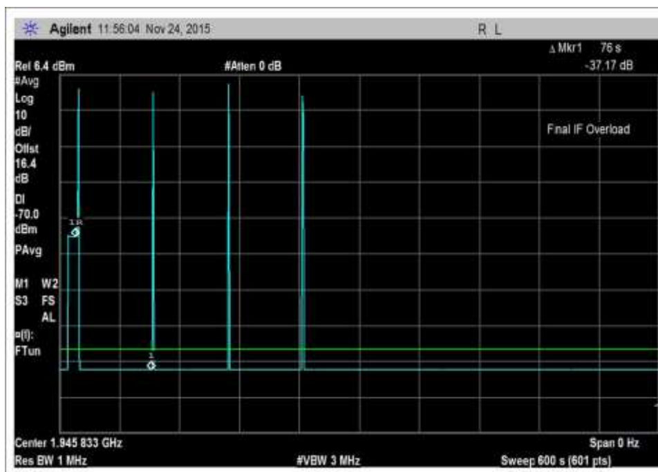
7.11_osc_DL-1930-1995MHz-600sec
