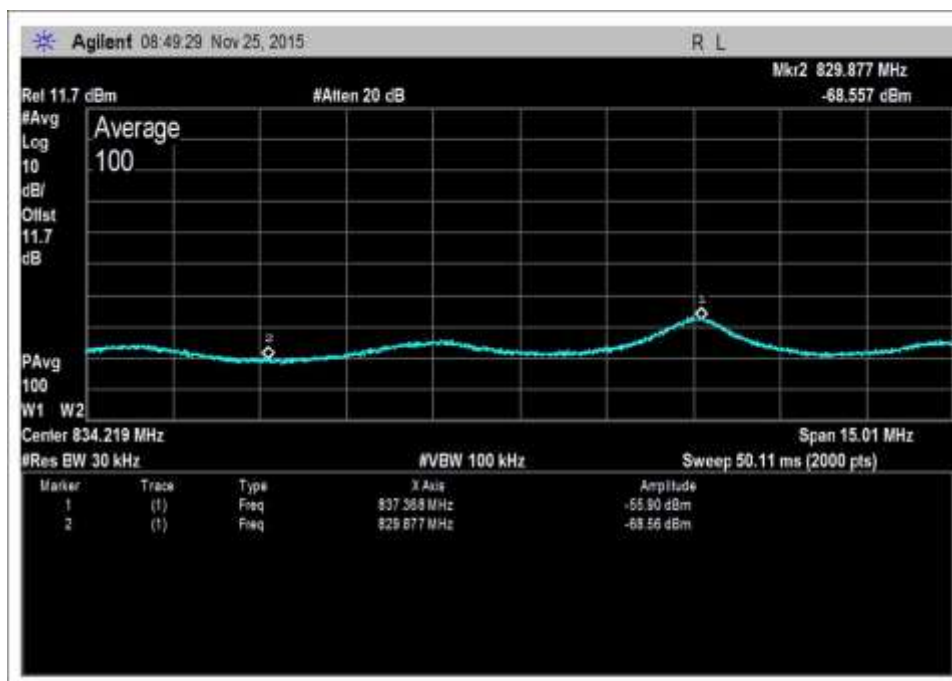
UL-824-849-AWGNR+1
