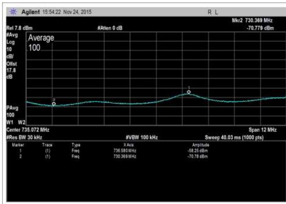
DL-728-746-AWGNR+3
