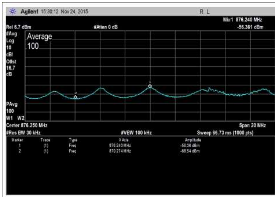
DL-869-894-AWGNR+2
