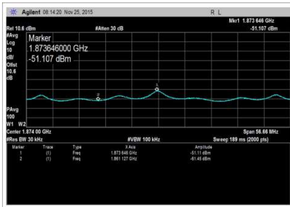
UL-1850-1915-AWGNR+5
