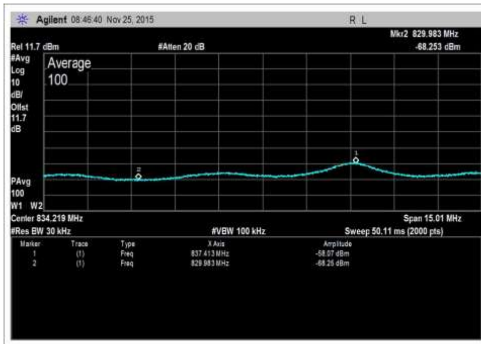
UL-824-849-AWGNR+4
