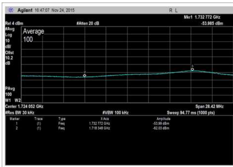
UL-1710-1755-AWGNR+4
