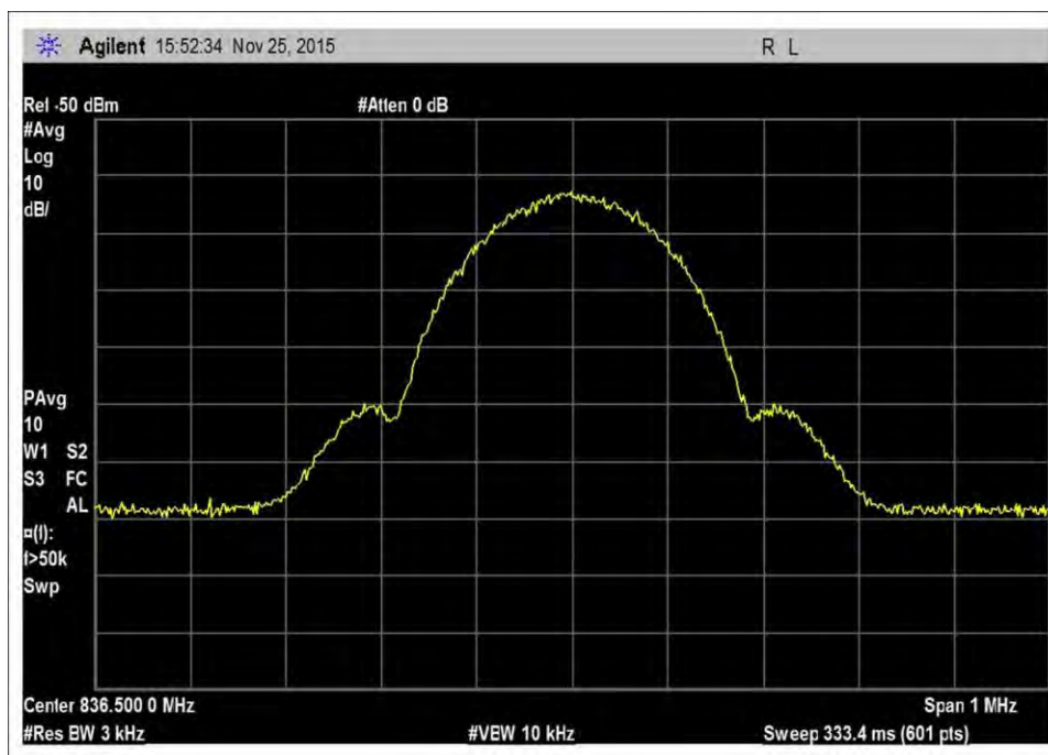
7.10_OBW_UL_824-849MHz_GSM
