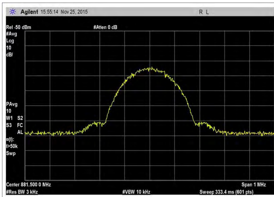
7.10_OBW_DL_869-894MHz_GSM
