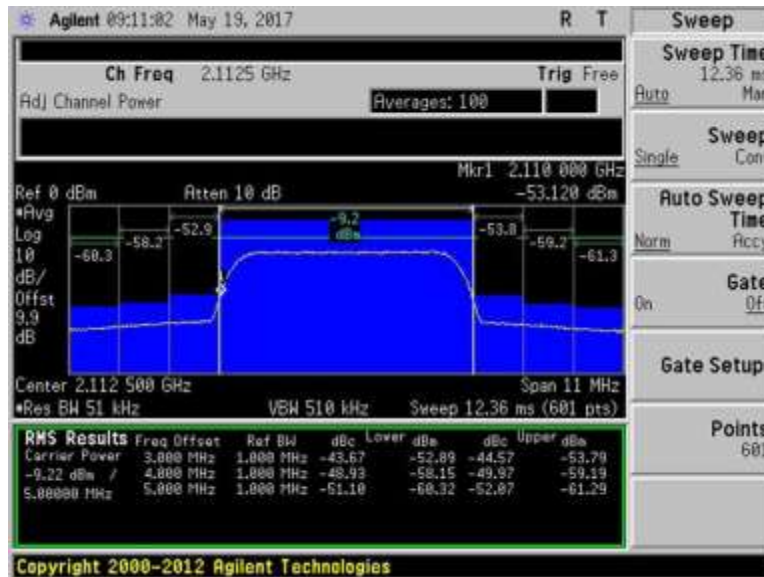
7.5_OBE_DL_2110-2155MHz_L_PreAGC_WCDMA
