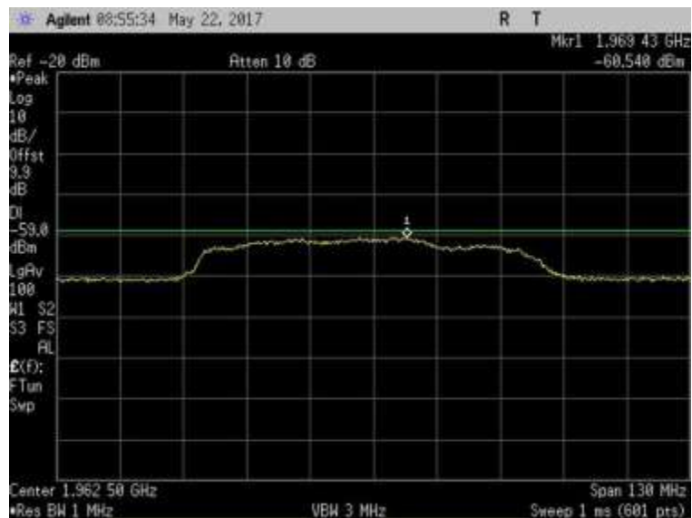
7.7.1_Noise_DL_1930-1995MHz
