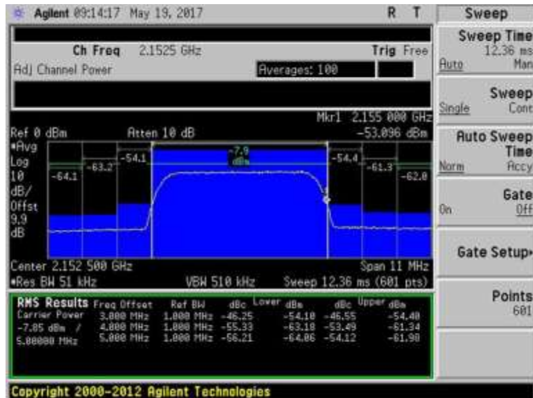
7.5_OBE_DL_2110-2155MHz_H_PreAGC_WCDMA
