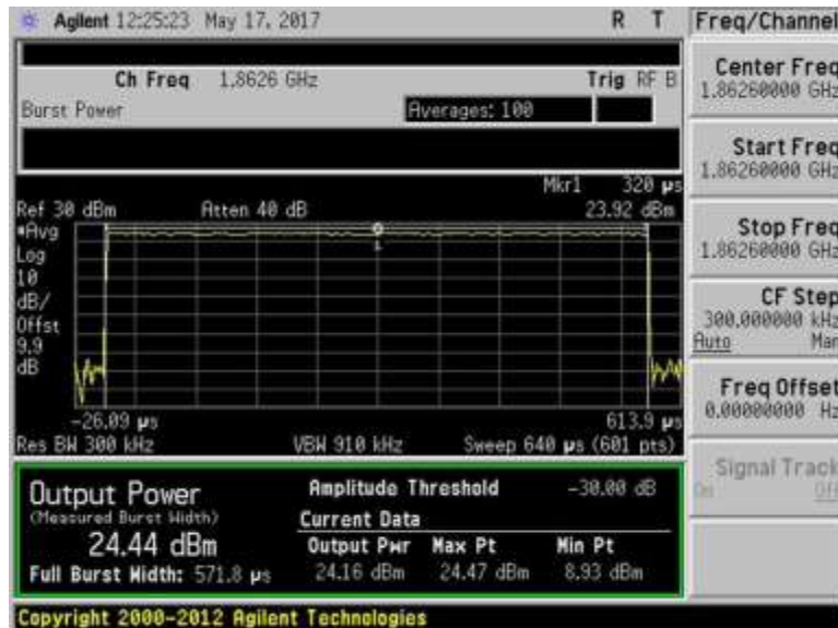
7.2_Power_UL_1850-1915MHz_GSM_Max
