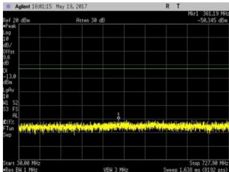
7.6_CSE_DL_728-746MHz_L
