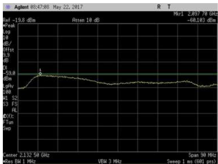
7.7.1_Noise_DL_2110-2155MHz
