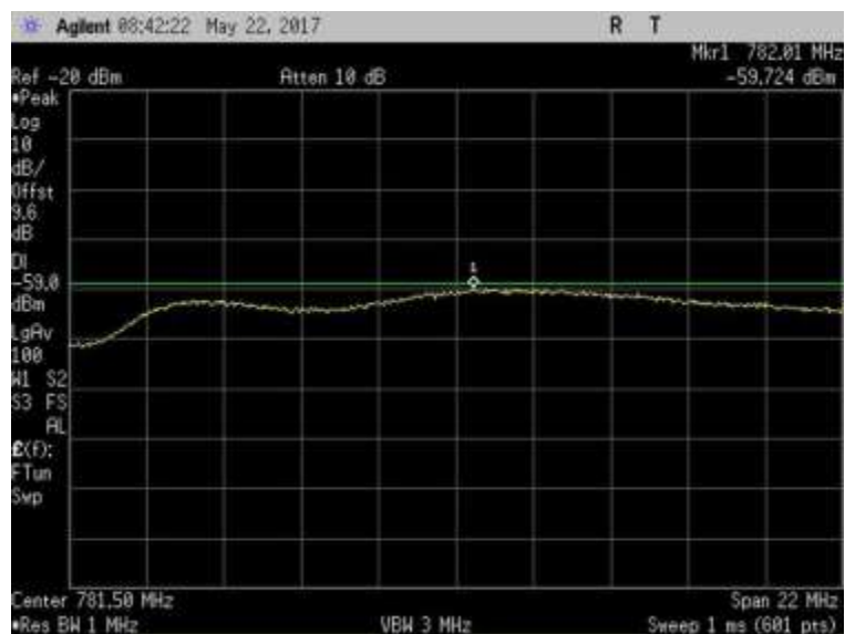
7.7.1_Noise_UL_776-787MHz
