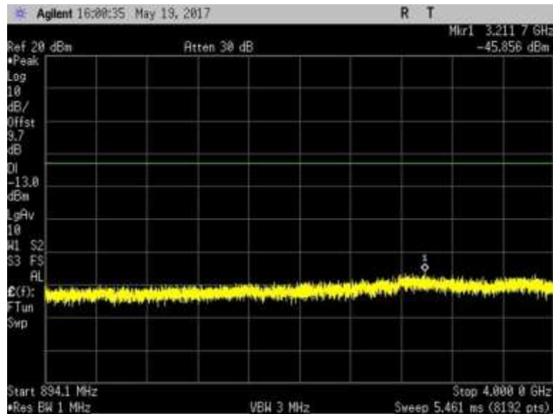
7.6_CSE_DL_869-894MHz_R1
