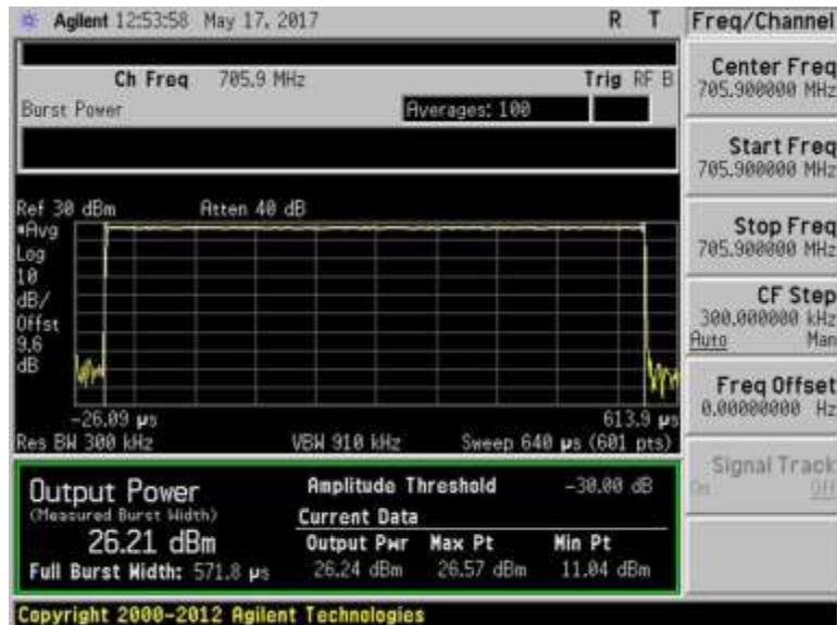
7.2_Power_UL_698-716MHz_GSM_Max
