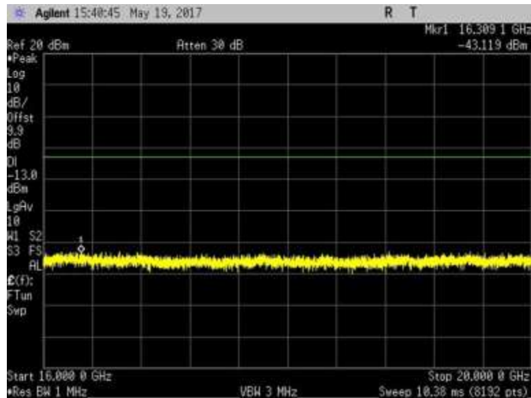
7.6_CSE_UL_1850-1915MHz_R5
