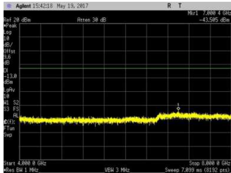
7.6_CSE_UL_698-716MHz_R2
