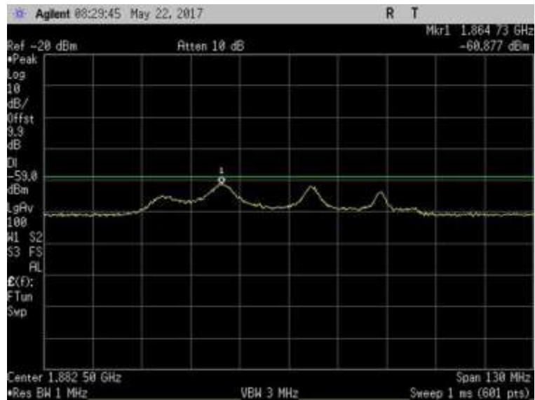
7.7.1_Noise_UL_1850-1915MHz
