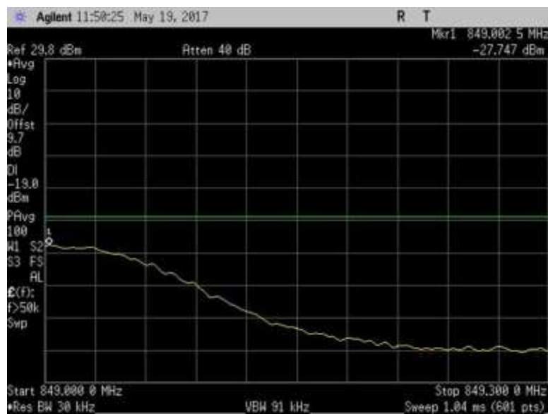
7.5_OBE_UL_824-849MHz_H_PreAGC_GSM
