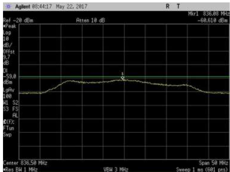
7.7.1_Noise_UL_824-849MHz
