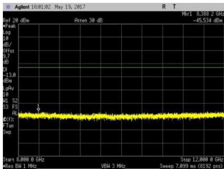
7.6_CSE_DL_869-894MHz_R3
