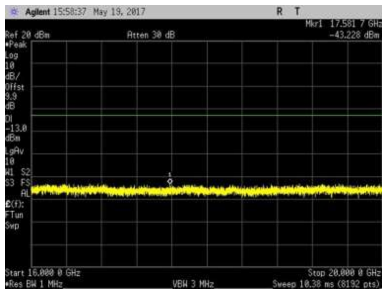
7.6_CSE_DL_2110-2155MHz_R5
