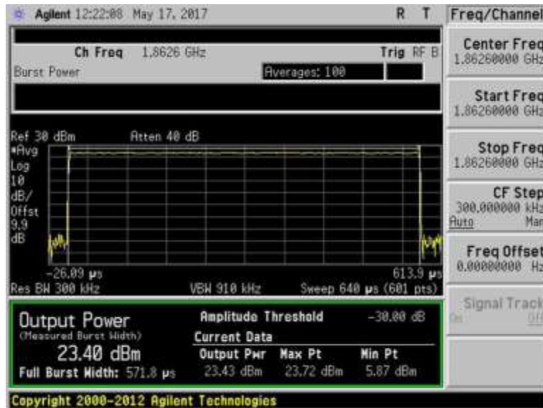
7.2_Power_UL_1850-1915MHz_GSM
