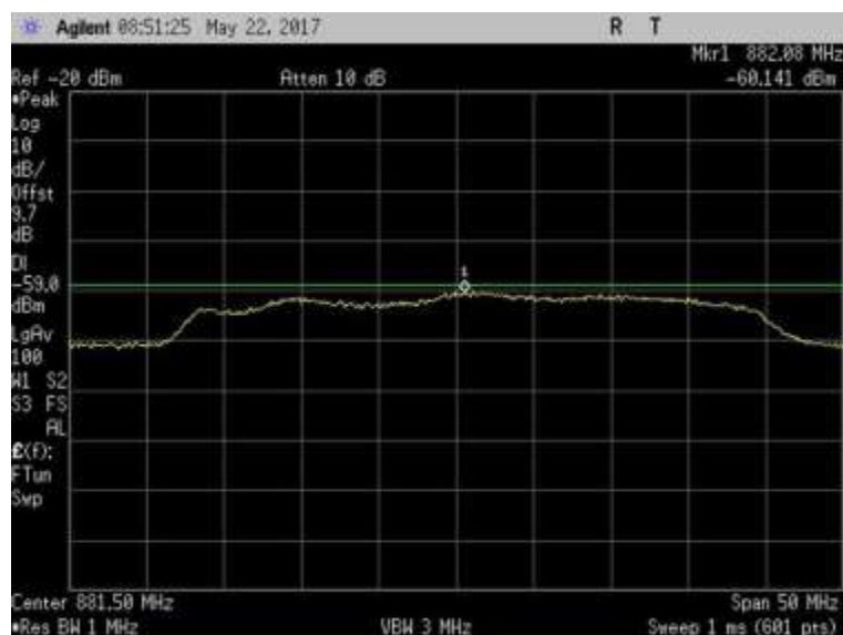
7.7.1_Noise_DL_869-894MHz
