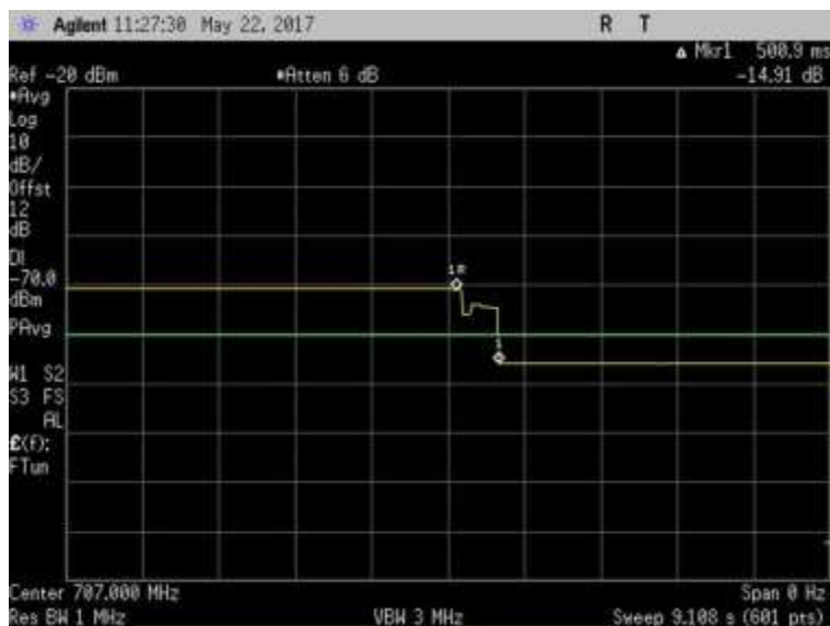
7.7.2_VarNoise_UL_698-716MHz
