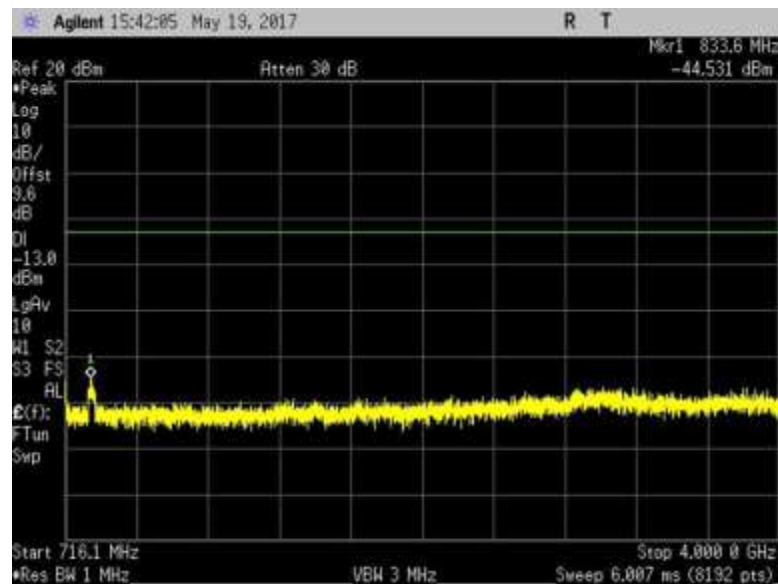
7.6_CSE_UL_698-716MHz_R1
