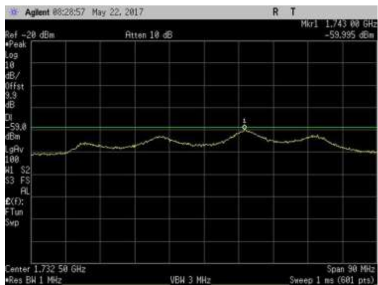
7.7.1_Noise_UL_1710-1755MHz
