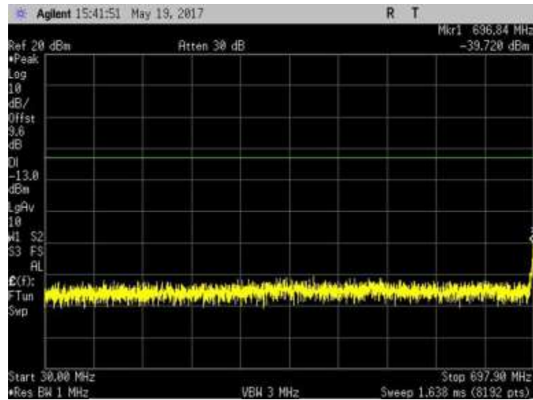
7.6_CSE_UL_698-716MHz_L
