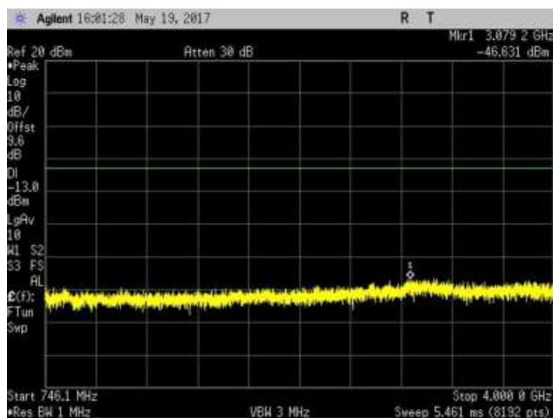
7.6_CSE_DL_728-746MHz_R1
