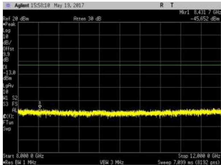
7.6_CSE_DL_2110-2155MHz_R3
