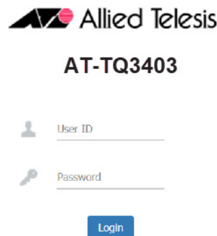
Figure 24. Login Prompt
