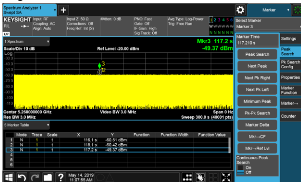
Signal 1, 5260MHz, 802.11ac VHT80
