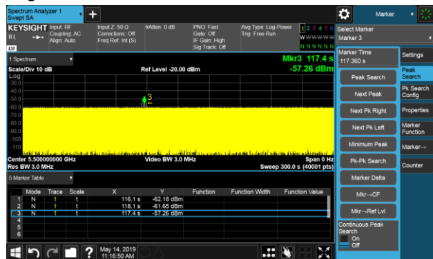
Signal 1, 5500MHz, 802.11ac VHT80
