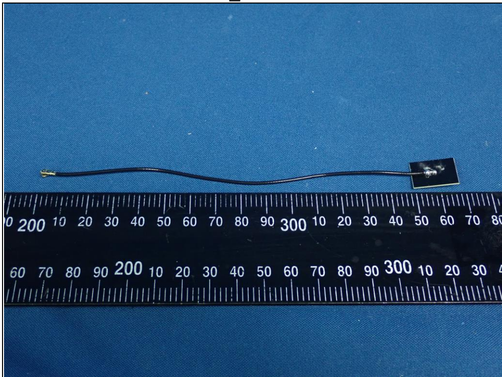
5GHz_Antenna 2
