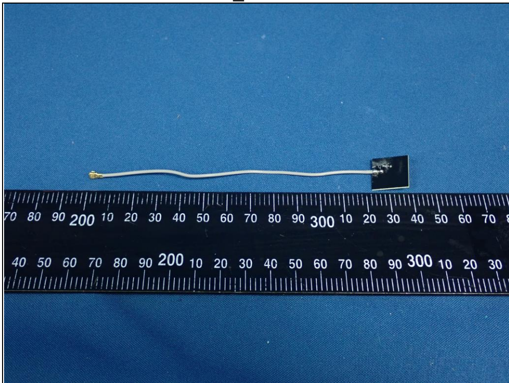
5GHz_Antenna 1
