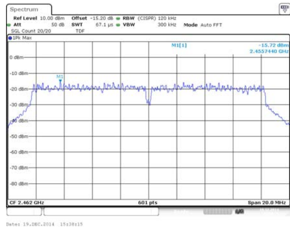
2462 MHz / Ant. 2
