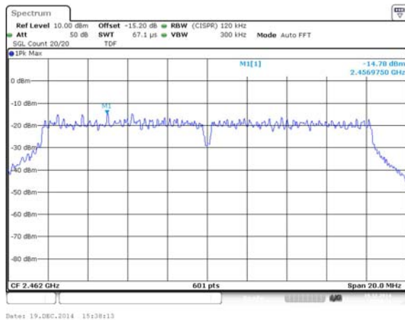
2462 MHz / Ant. 1
