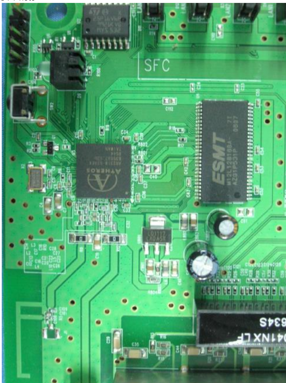
(9) EUT Photo
