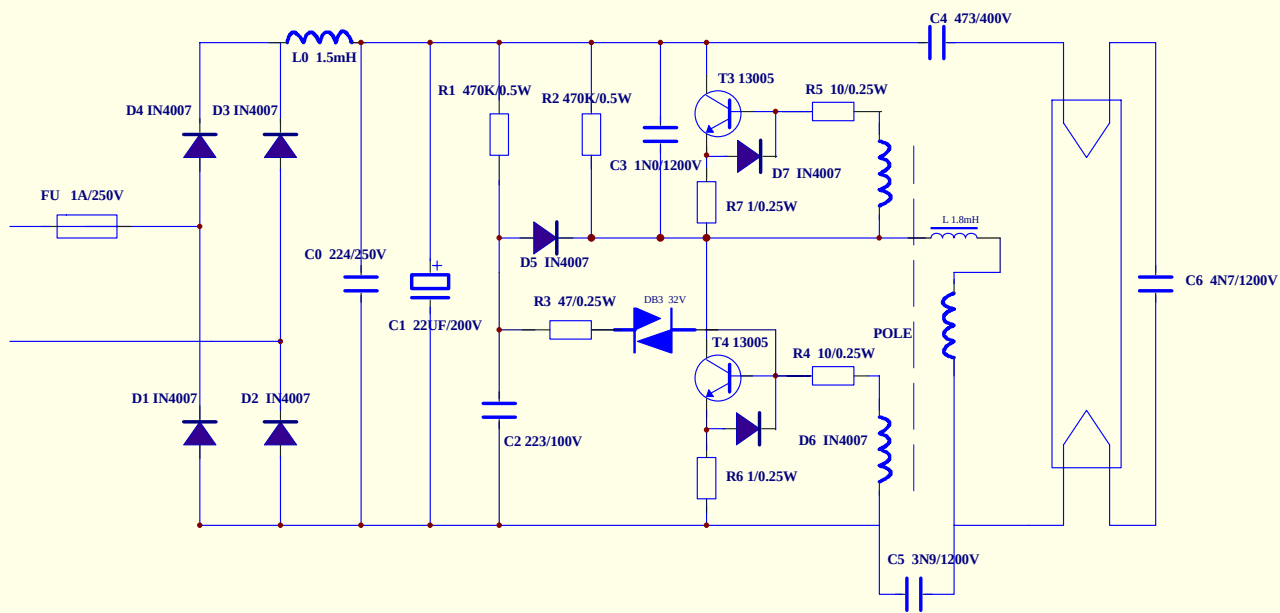
SFU-201线路原理图
