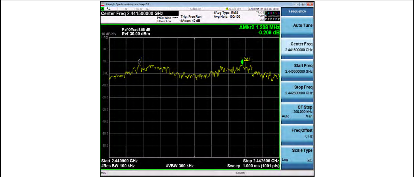
π/4DQPSK
