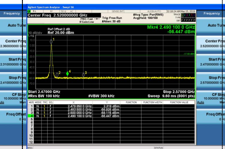
Right Band edge hoping off
