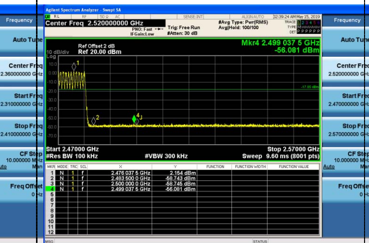
Right Band edge hoping on
