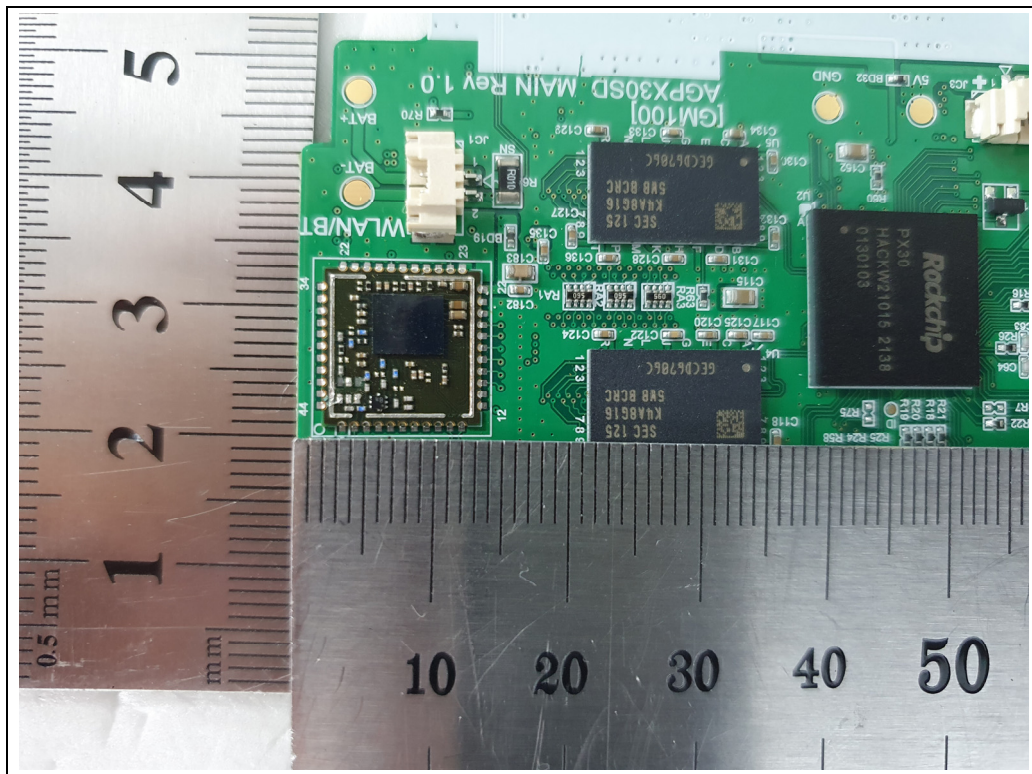
&lt;BT, WLAN Module&gt;
