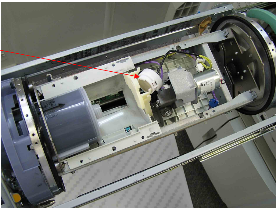
RF Module-2
