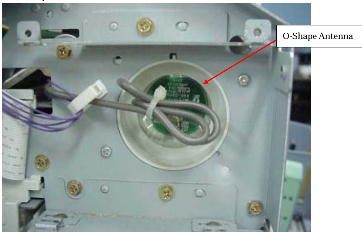
写真4 O-Shape Antenna 取り付け状態 (上部写真の左から撮影)
