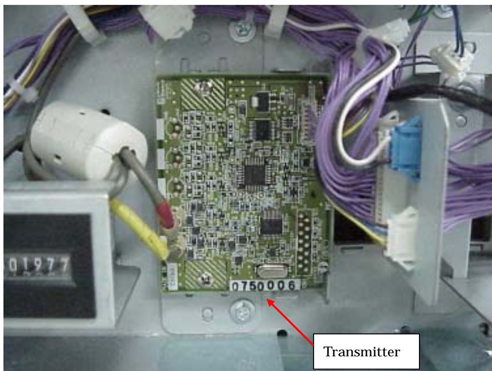
写真2 無線器取り付け状態
