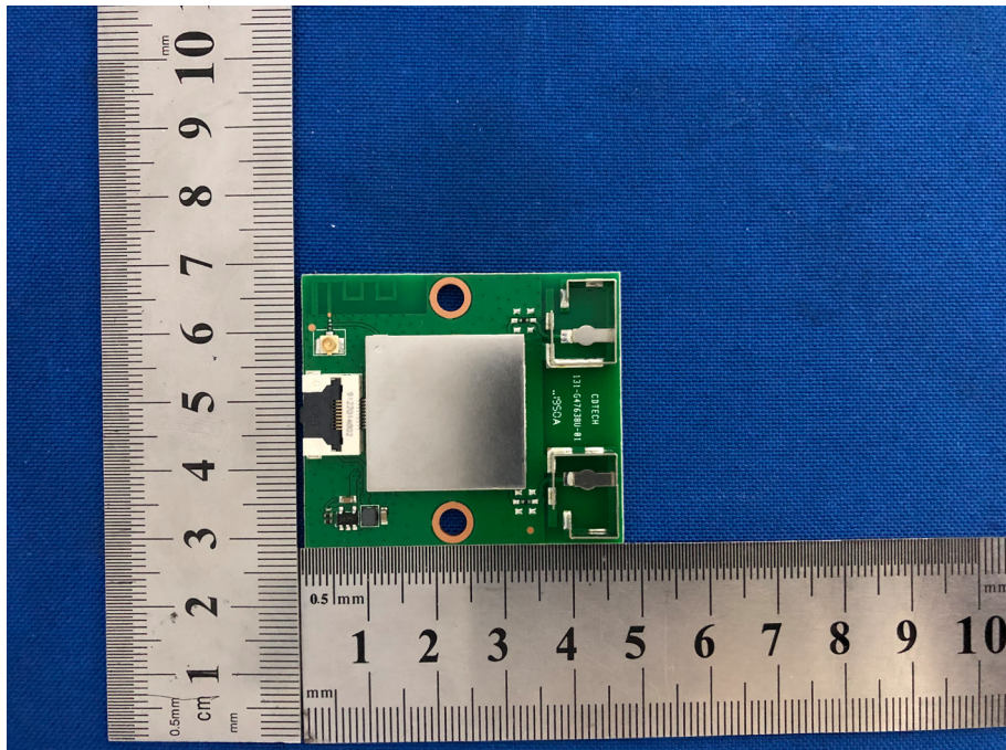
EUT Photo 2
