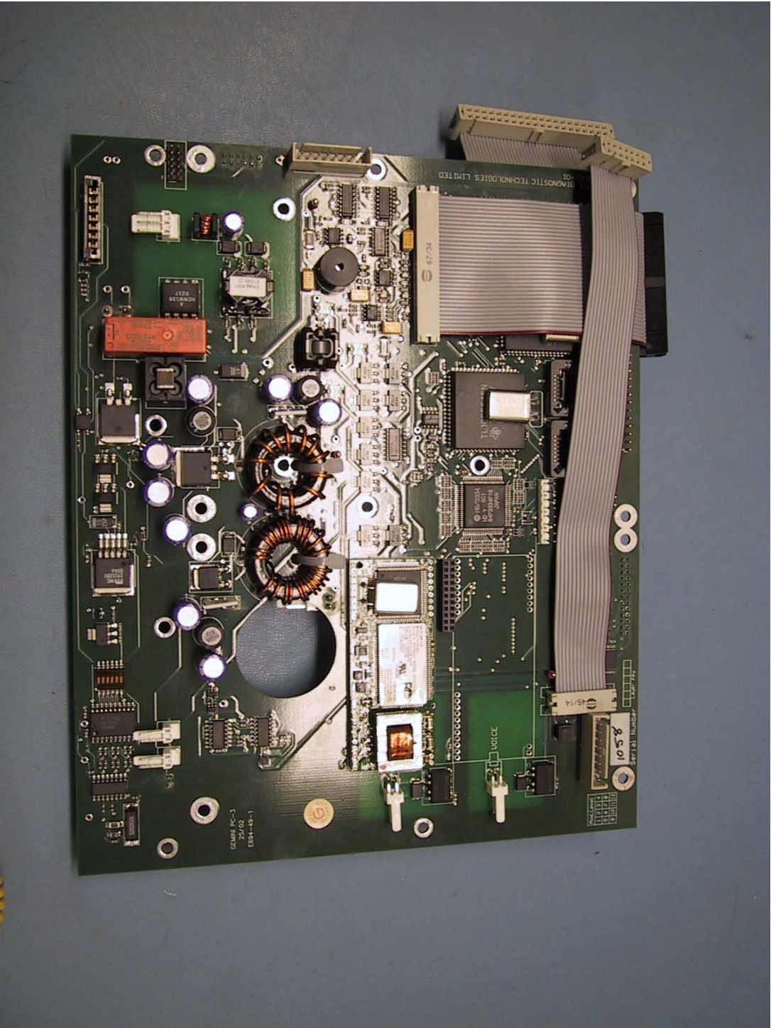
Tempus PCB 1
