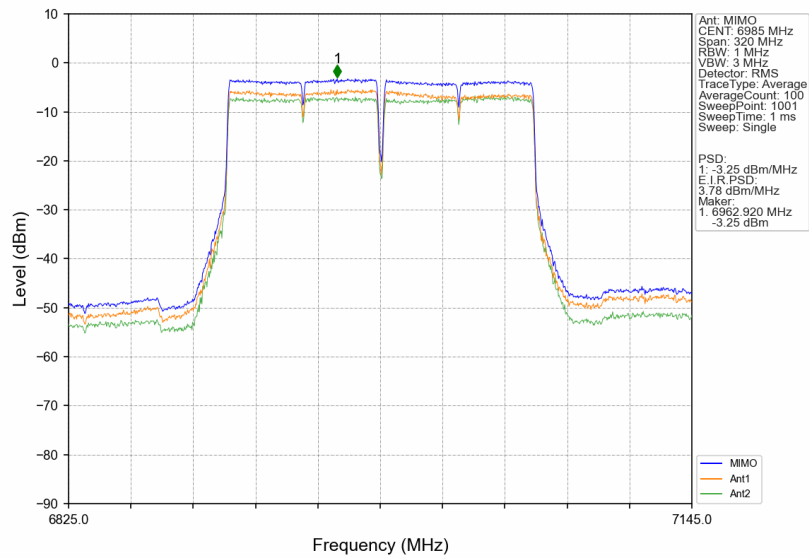
802.11ax(VHT160)_MCH_6985MHz_MIMO_NTNV
