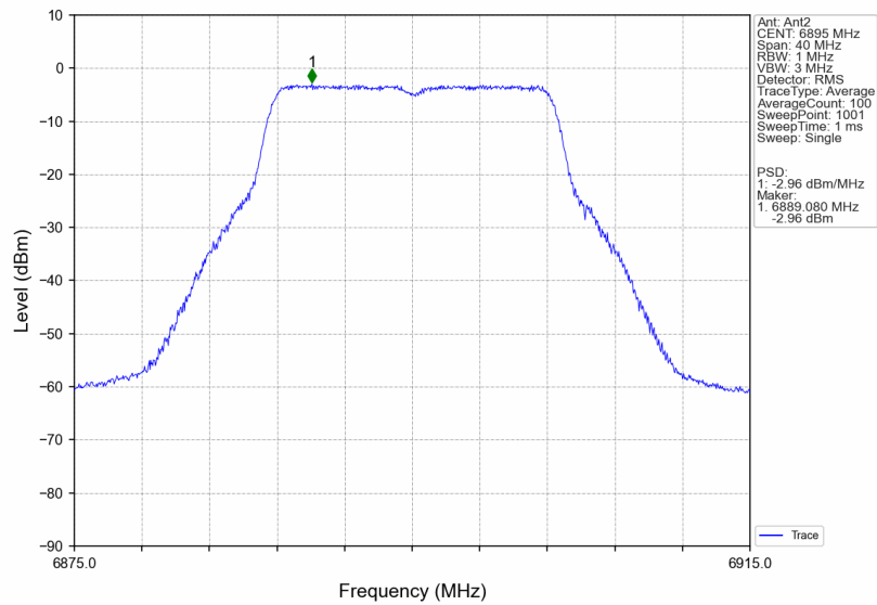
802.11a_LCH_6895MHz_Ant2_NTNV
