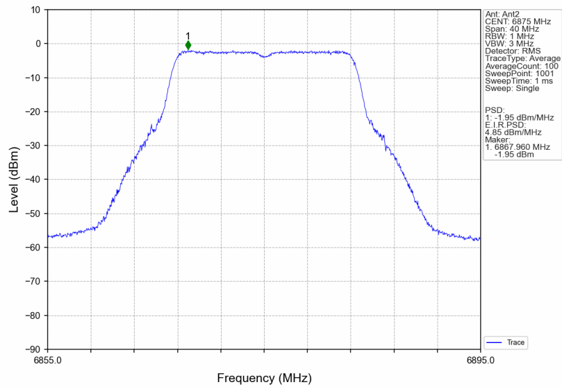
802.11a_HCH_6875MHz_Ant2_NTNV
