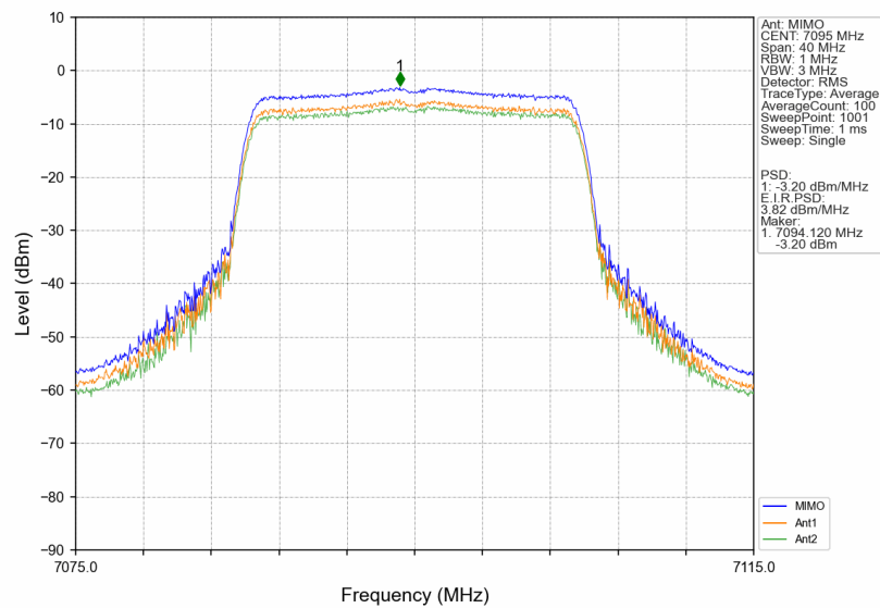
802.11ax(VHT20) HCH 7095MHz_MIMO_NTNV
