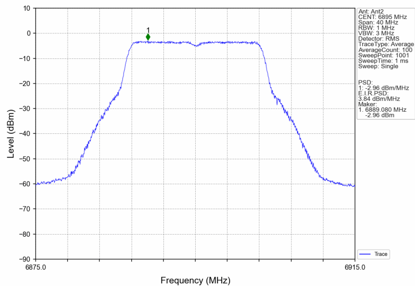
802.11a_LCH_6895MHz_Ant2_NTNV
