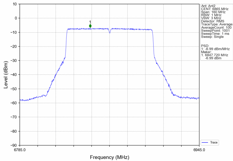
802.11ax(VHT80)_HCH_6865MHz_Ant2_NTNV
