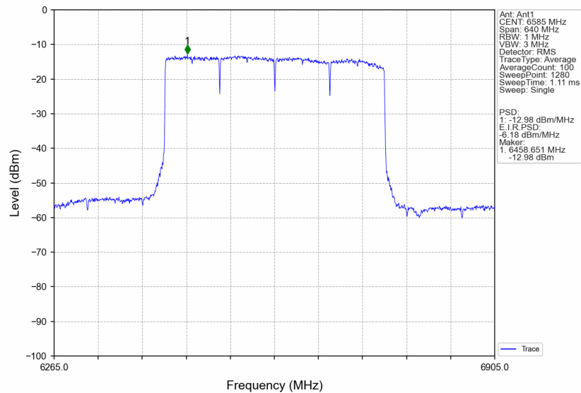
802.11be(EHT320)_MCH_6585MHz_4xRU996_Left_Ant1_NTNV
