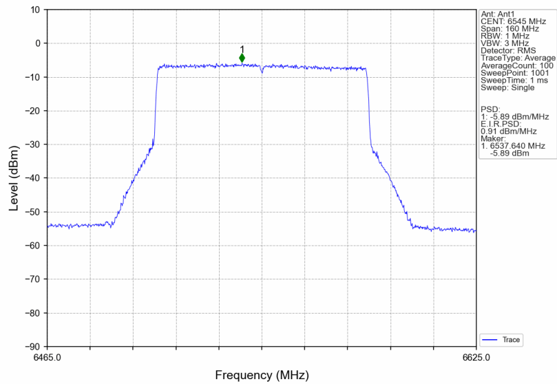
802.11be(EHT80)_HCH_6545MHz_RU996_Left_Ant1_NTNV
