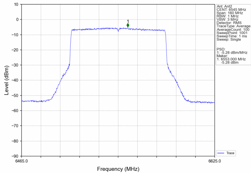
802.11be(EHT80)_HCH_6545MHz_RU996_Left_MIMO_NTNV
