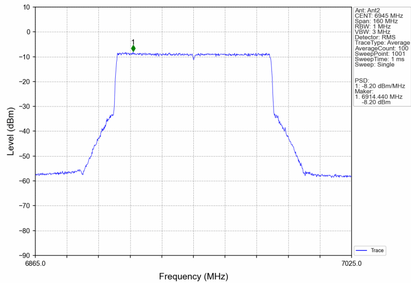
802.11be(EHT80)_LCH_6945MHz_RU996_Left_MIMO_NTNV
