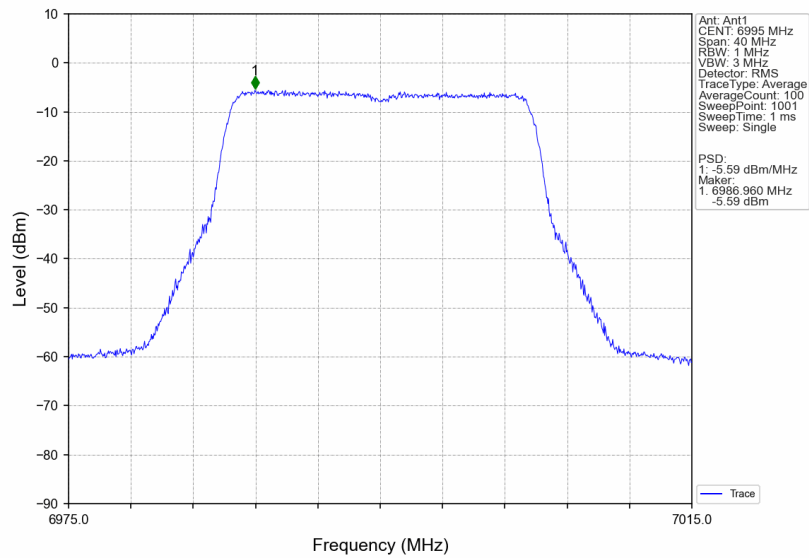
802.11be(EHT20)_MCH_6995MHz_RU242_Left_Ant1_NTNV
