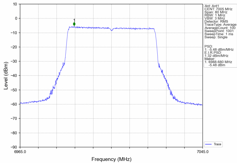
802.11be(EHT40)_MCH_7005MHz_RU484_Left_Ant1_NTNV
