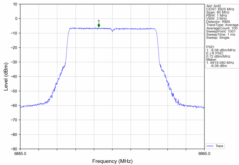
802.11be(EHT40)_LCH_6925MHz_RU484_Left_Ant2_NTNV
