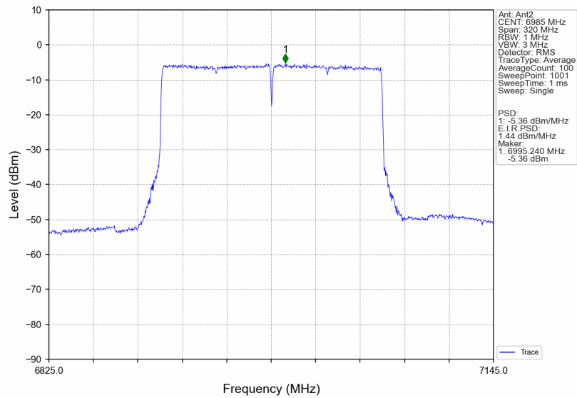
802.11be(EHT160)_MCH_6985MHz_2xRU996_Left_MIMO_NTNV
