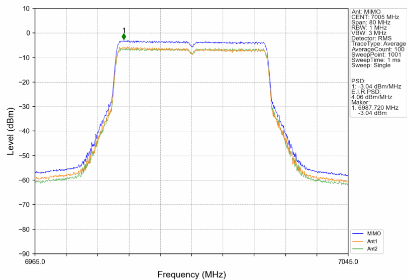
802.11be(EHT40)_MCH_7005MHz_RU484_Left_MIMO_NTNV
