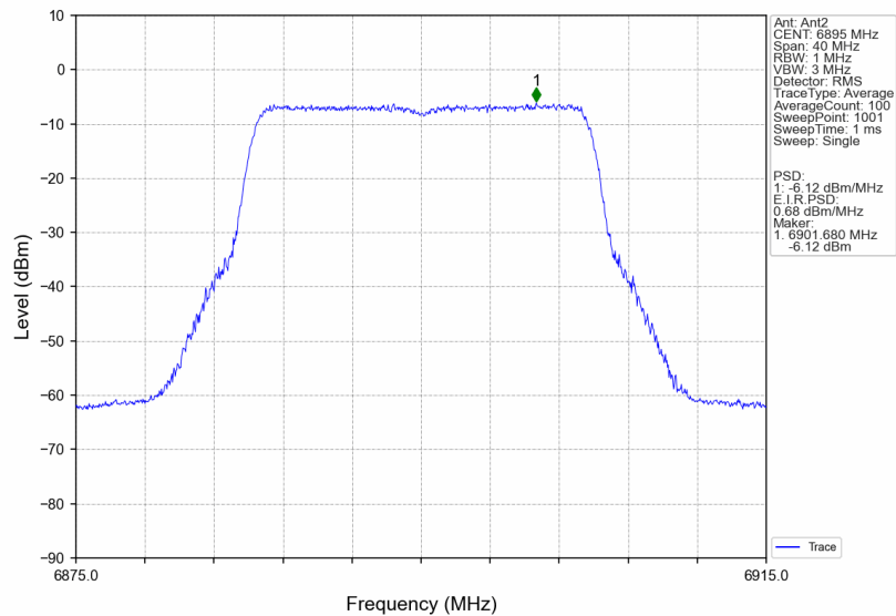
802.11be(EHT20)_LCH_6895MHz_RU242_Left_Ant2_NTNV
