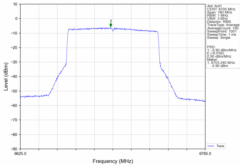
802.11be(EHT80)_MCH_6705MHz_RU996_Left_Ant1_NTNV
