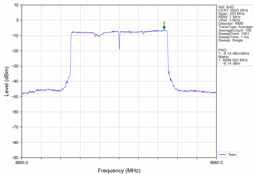
802.11be(EHT160)_HCH_6825MHz_2xRU996_Left_MIMO_NTNV
