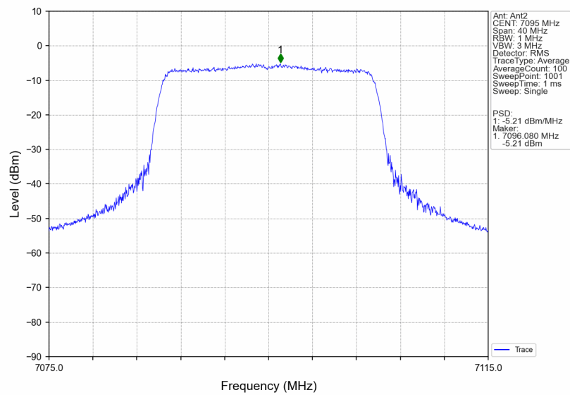
802.11be(EHT20)_HCH_7095MHz_RU242_Left_MIMO_NTNV
