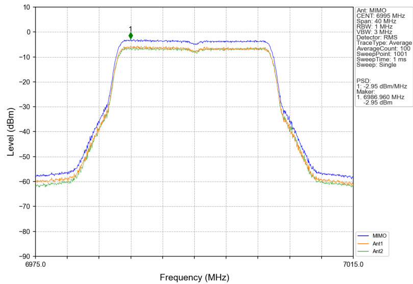
802.11be(EHT20)_MCH_6995MHz_RU242_Left_MIMO_NTNV
