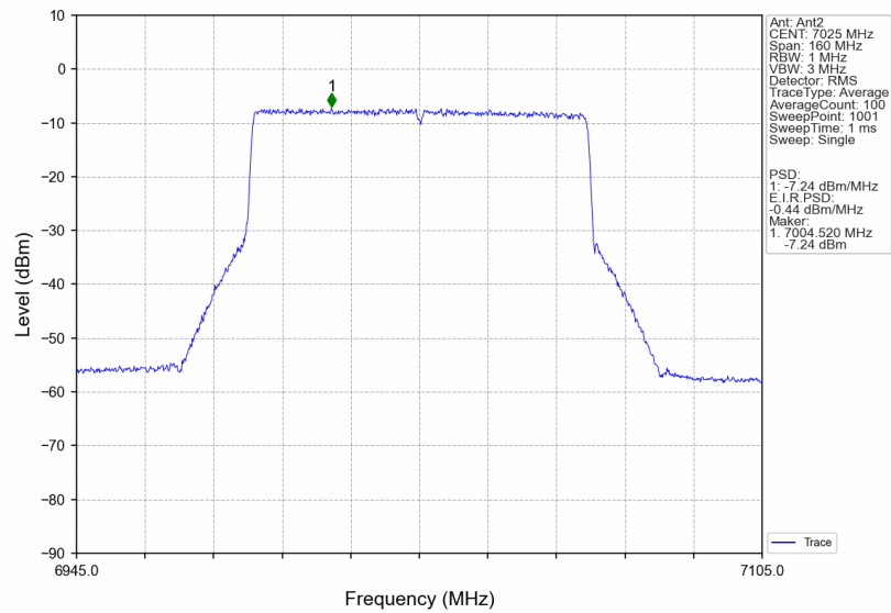
802.11be(EHT80)_HCH_7025MHz_RU996_Left_Ant2_NTNV
