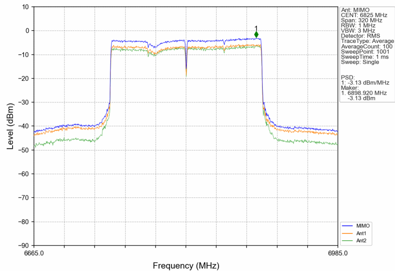
802.11be(EHT160)_HCH_6825MHz_2xRU996_Left_MIMO_NTNV
