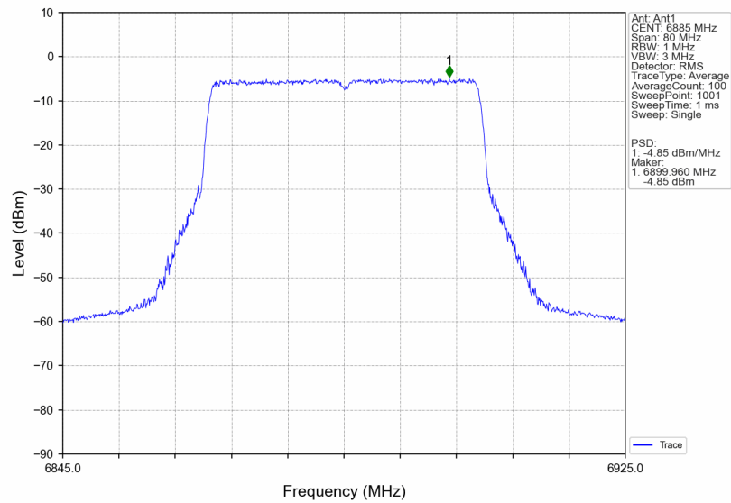
802.11be(EHT40)_HCH_6885MHz_RU484_Left_Ant1_NTNV
