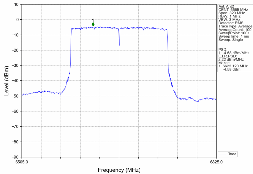
802.11be(EHT160)_MCH_6665MHz_2xRU996_Left_MIMO_NTNV
