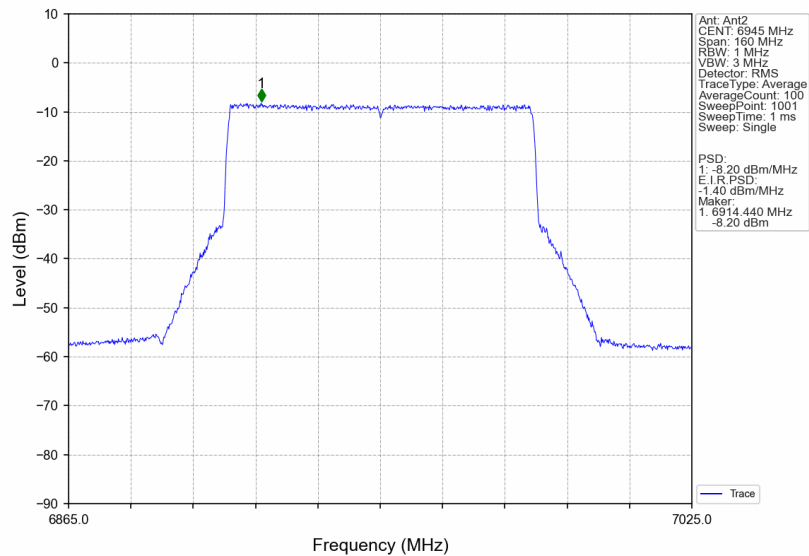
802.11be(EHT80)_LCH_6945MHz_RU996_Left_MIMO_NTNV
