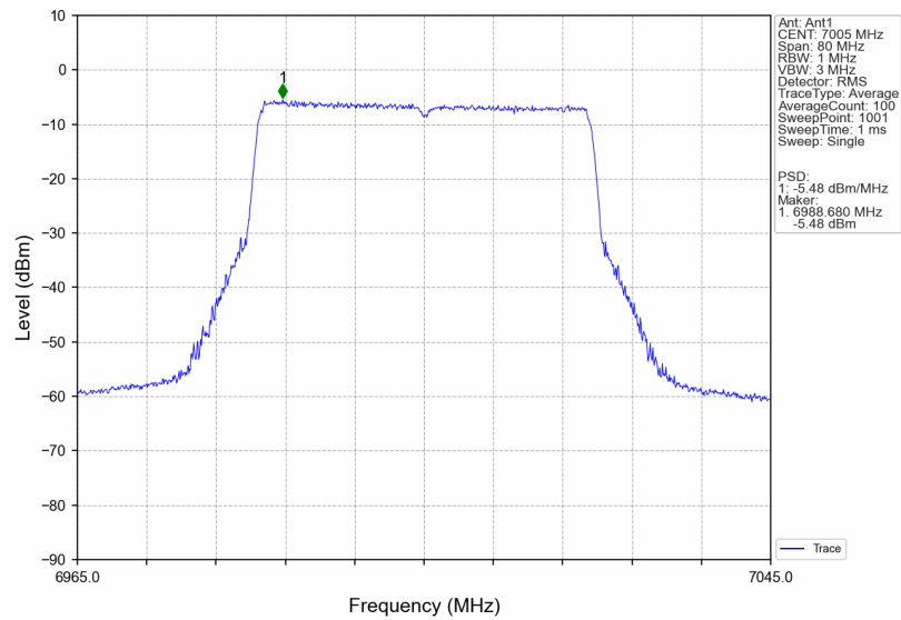
802.11be(EHT40)_MCH_7005MHz_RU484_Left_Ant1_NTNV
