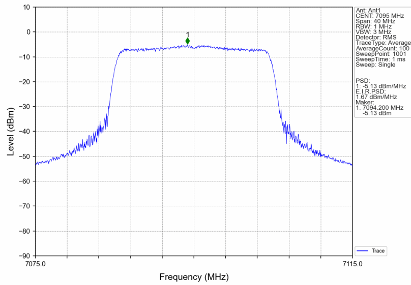
802.11be(EHT20)_HCH_7095MHz_RU242_Left_Ant1_NTNV
