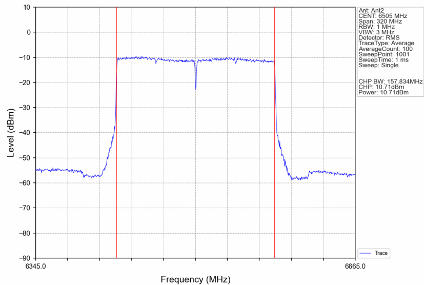
802.11be(EHT160)_HCH_6505MHz_2xRU996_Left_Ant2_NTNV
