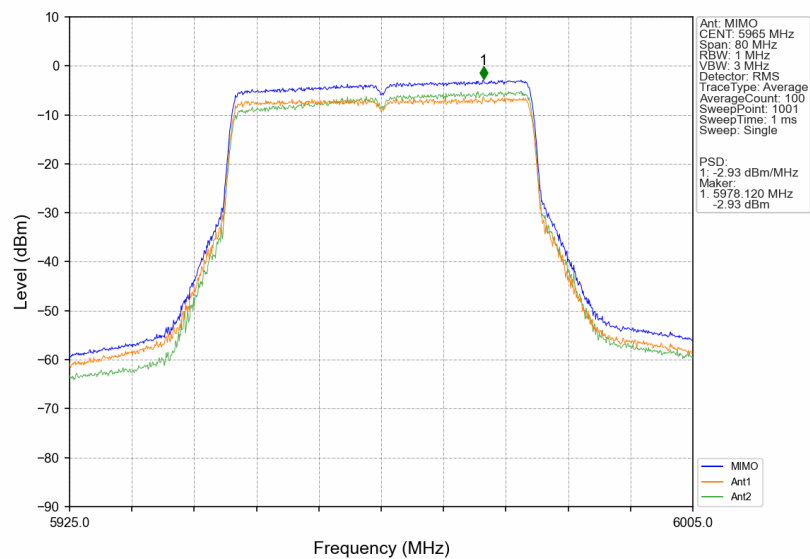
802.11be(EHT40)_LCH_5965MHz_RU484_Left_MIMO_NTNV
