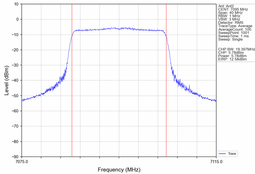
802.11be(EHT20)_HCH_7095MHz_RU242_Left_Ant2_NTNV
