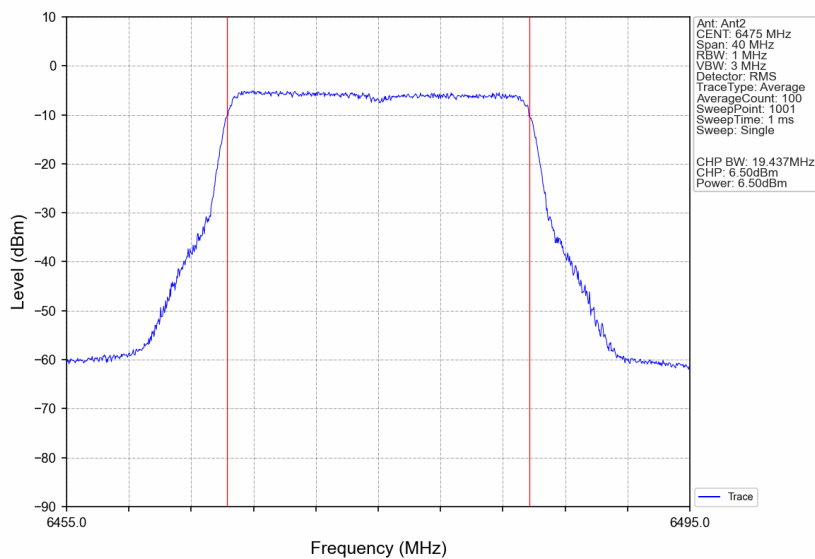
802.11be(EHT20)_MCH_6475MHz_RU242_Left_Ant2_NTNV
