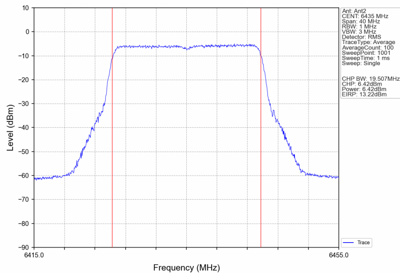
802.11be(EHT20)_LCH_6435MHz_RU242_Left_Ant2_NTNV
