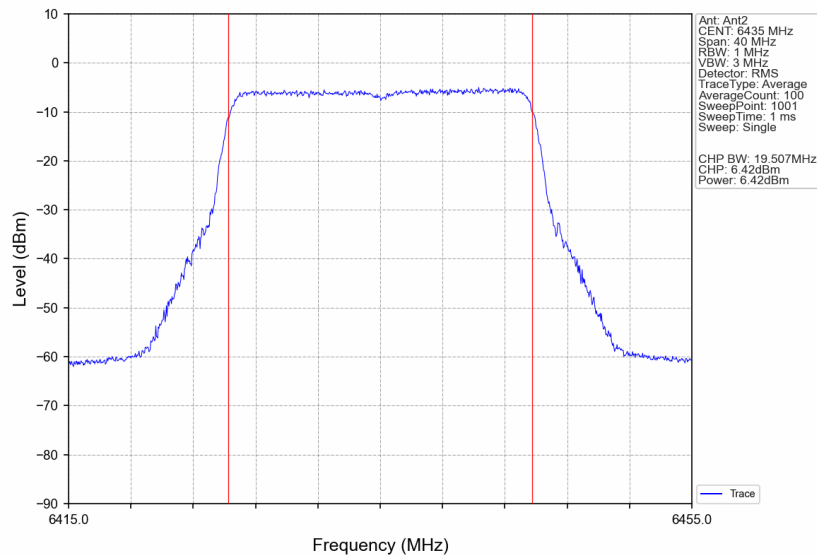
802.11be(EHT20)_LCH_6435MHz_RU242_Left_Ant2_NTNV
