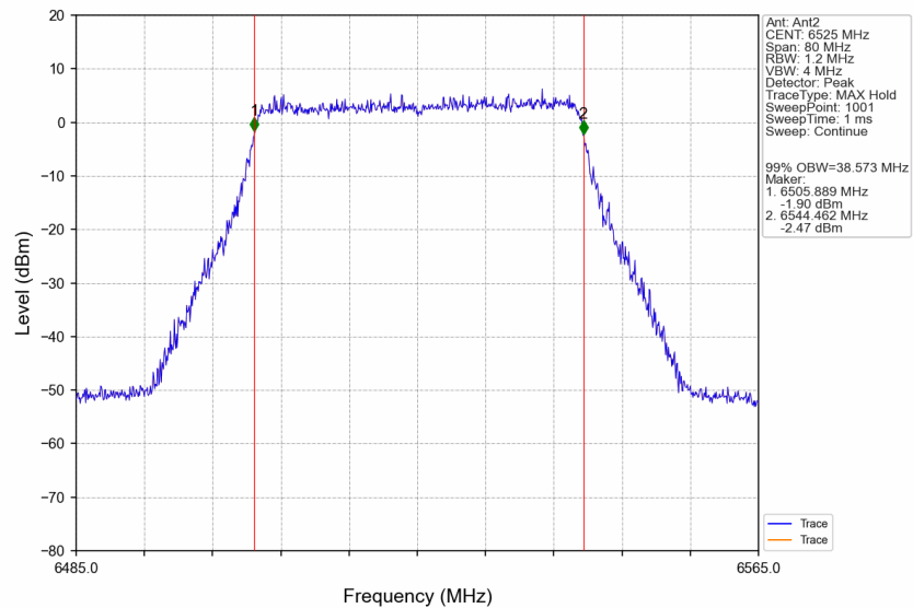
802.11be(EHT40)_HCH_6525MHz_RU484_Left_Ant2_NTNV
