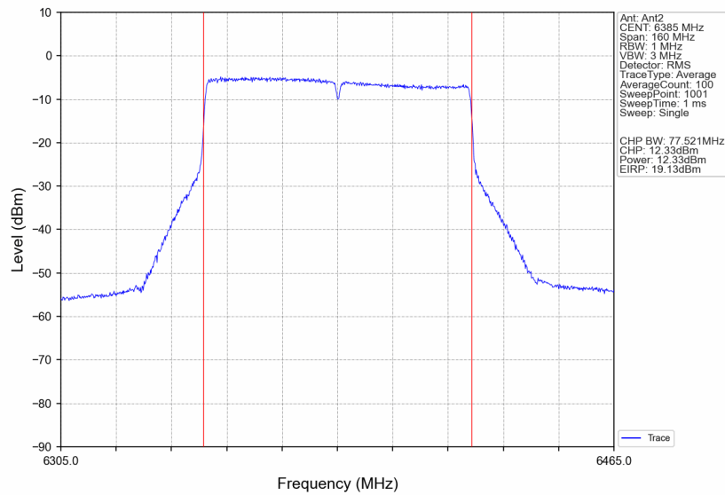
802.11ax(VHT80)_HCH_6385MHz_Ant2_NTNV
