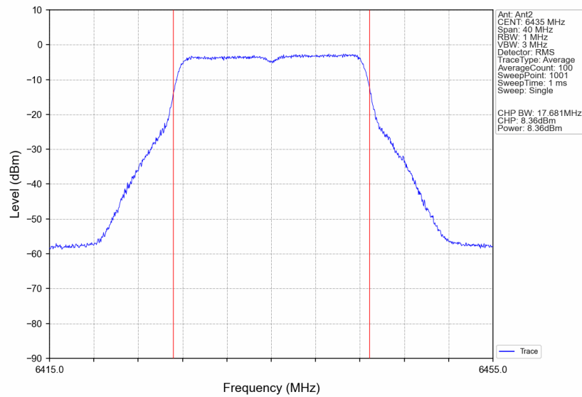
802.11a_LCH_6435MHz_Ant2_NTNV
