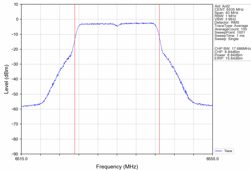
802.11a_LCH_6535MHz_Ant2_NTNV
