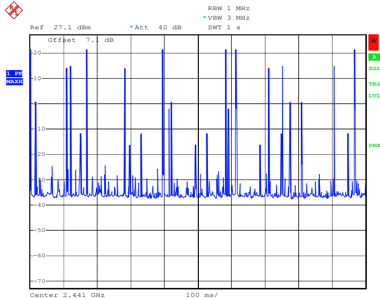
Figure 8. 5 DH 3 bursts
