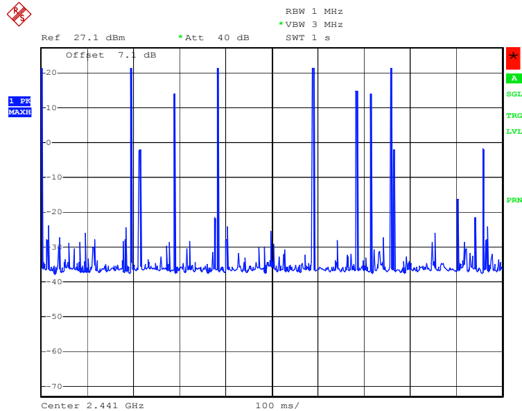
Figure 10. 4 DH 5 bursts
