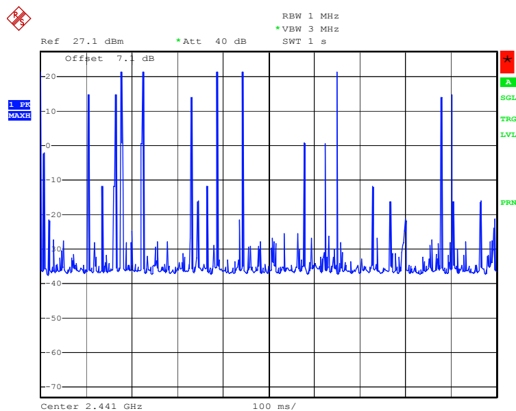
Figure 8. 5 DH 3 bursts
