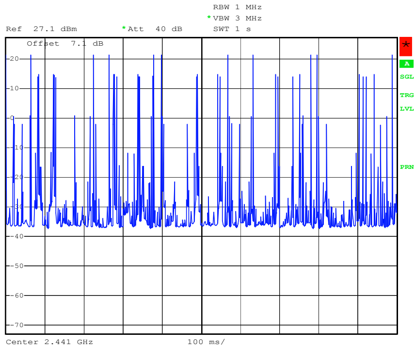
Figure 6. 10 DH 1 bursts
