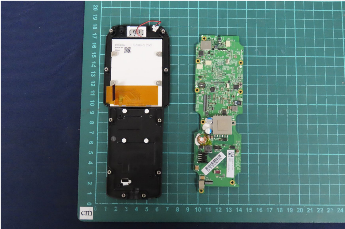
(16) EUT Photo
