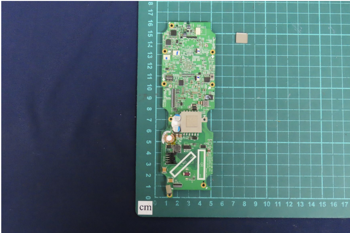
(30) EUT Photo
