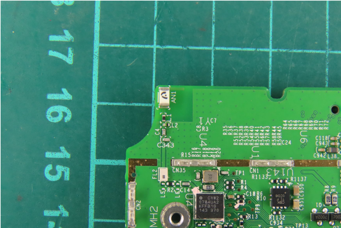
(37) EUT Photo
