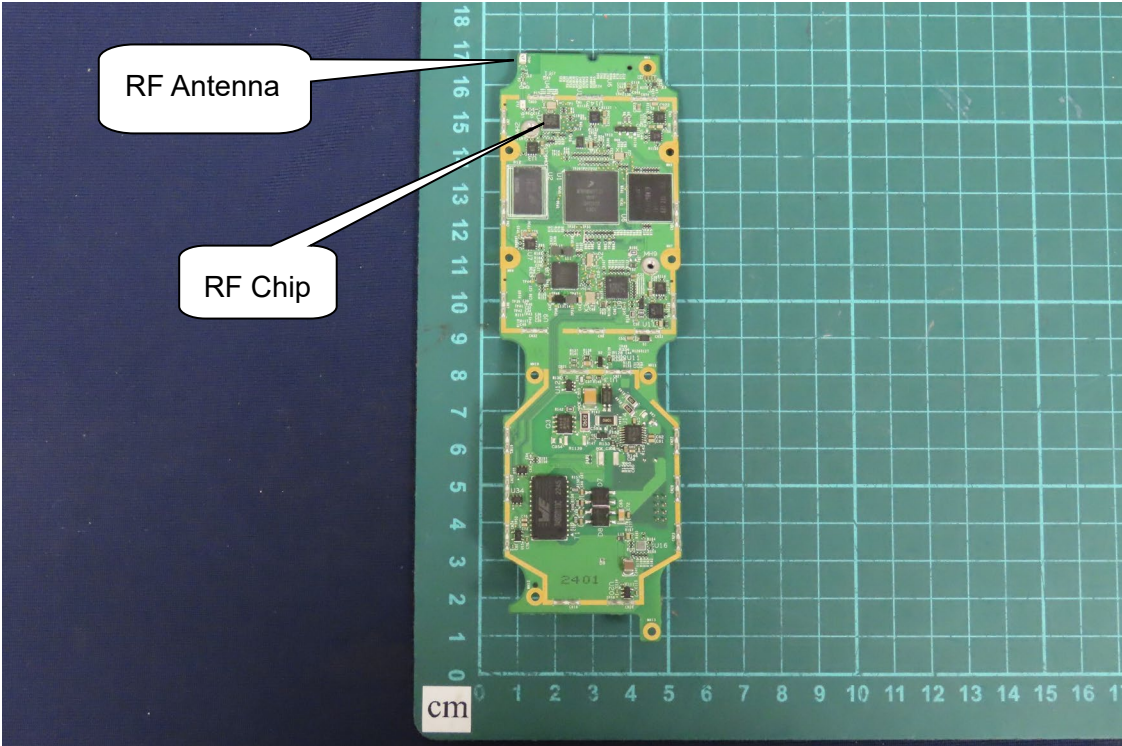
(24) EUT Photo
