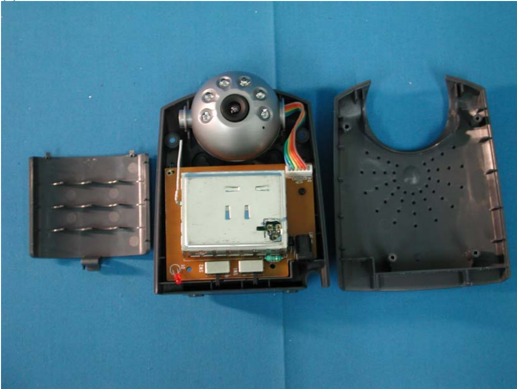
(4) EUT Photo
