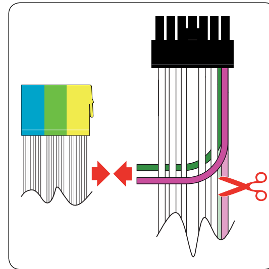
Fig. 06: Connection for the mini ISO connection cable
