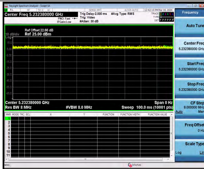
11AX40MIMO_Ant2_5230_484Tone_RU65
