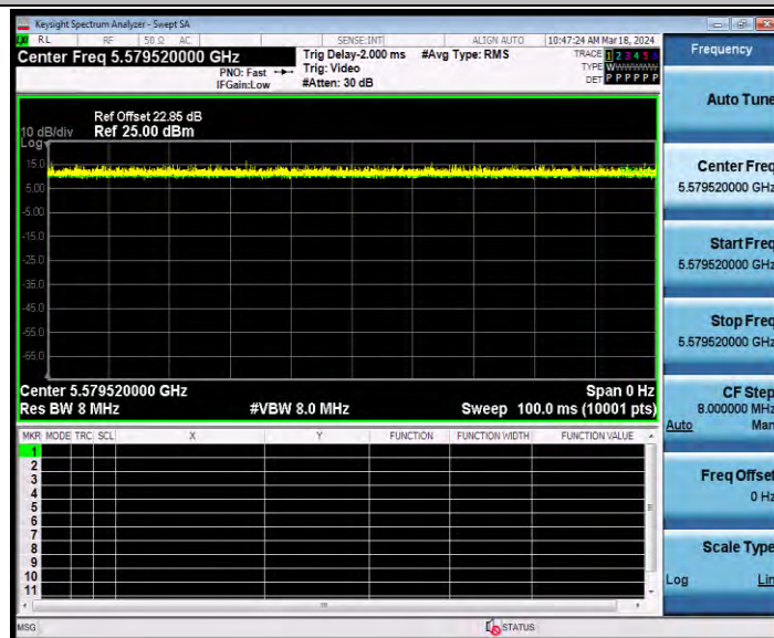
11AX20MIMO_Ant2_5580_26Tone_RU4
