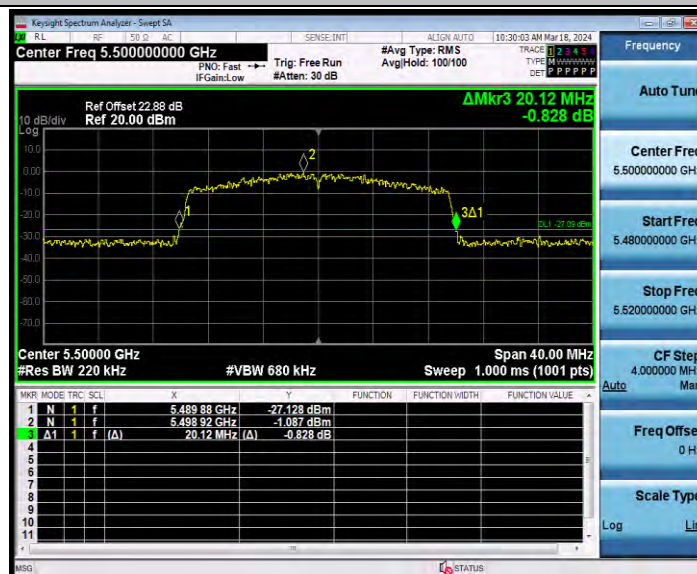
11AX20MIMO_Ant1_5500_242Tone_RU61
