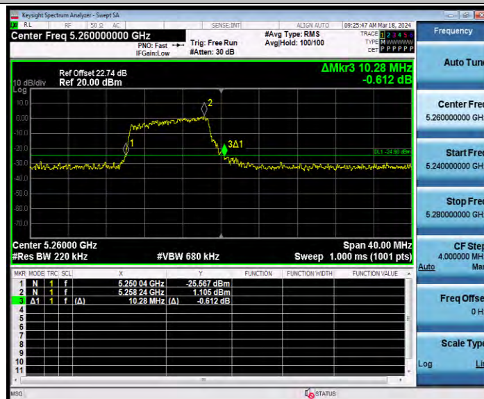
11AX20MIMO_Ant2_5260_242Tone_RU61
