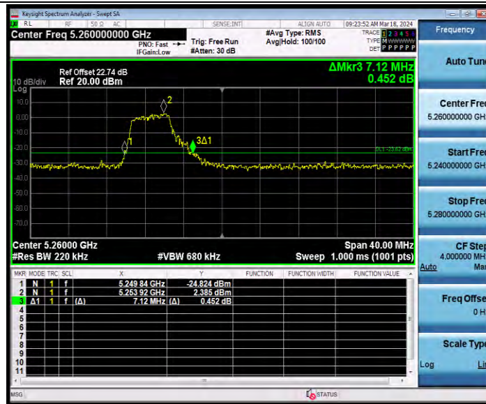
11AX20MIMO_Ant2_5260_106Tone_RU53
