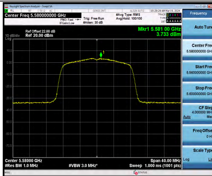
11A-CDD_Ant1_5700
