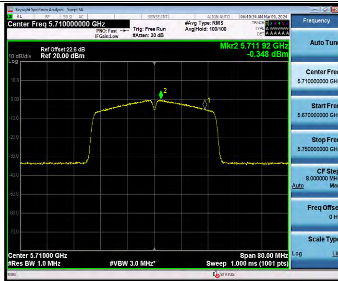
11N40MIMO_Ant1_5710_UNII-3
