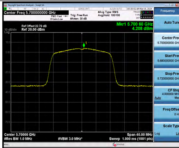
11A-CDD_Ant2_5700
