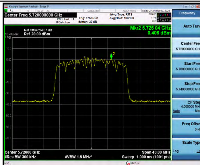
11N20MIMO_Ant1_5720_UNII-3
