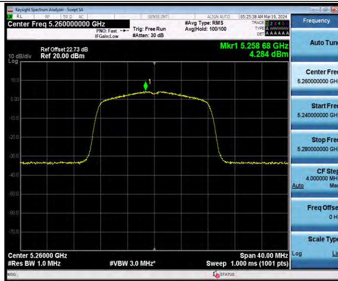
11A-CDD_Ant2_5260
