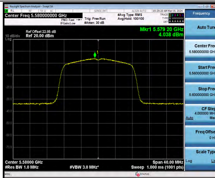
11A-CDD_Ant2_5580
