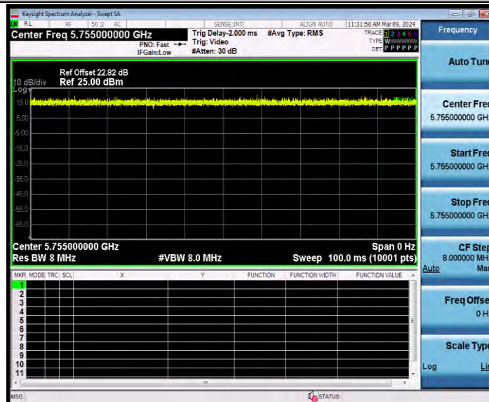
11AX40MIMO_Ant2_5755
