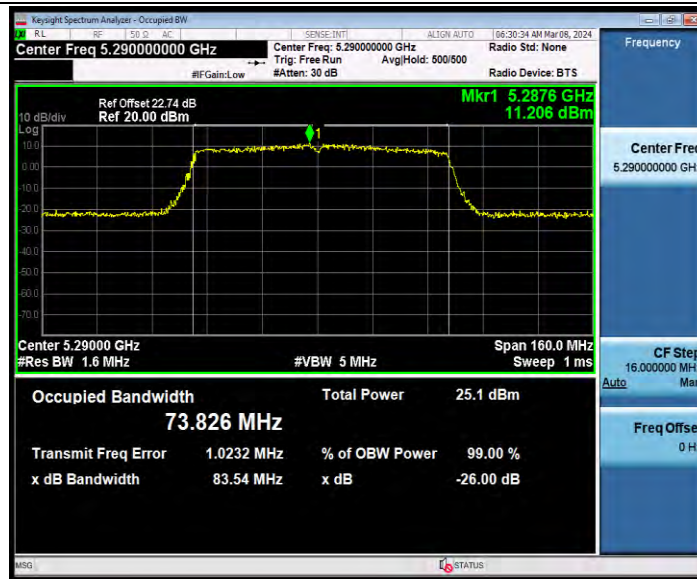
11AX80ISO_Ant2_5290
