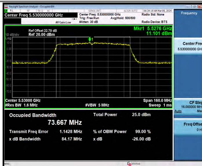
11AX80ISO_Ant1_5530
