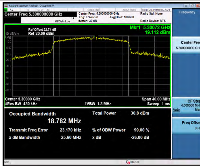
11AX20SISO_Ant2_5300
